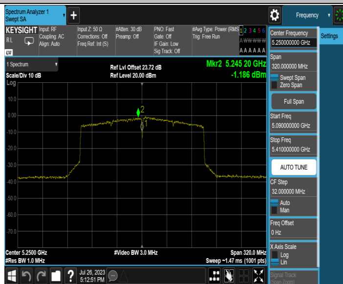
11AX160MIMO_Ant1_5250_UNII-2A
