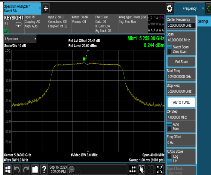
11AX20MIMO_Ant2_5260
