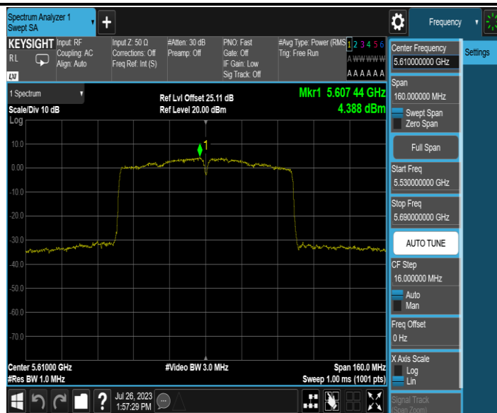
11AC80MIMO_Ant2_5610
