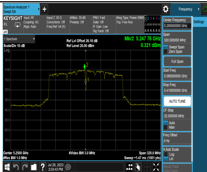
11AC160MIMO_Ant2_5250_UNII-1
