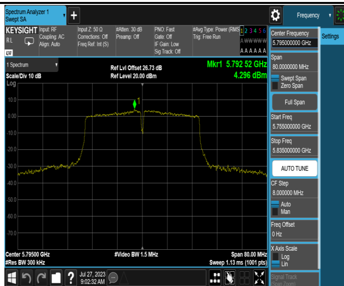
11N40MIMO_Ant2_5795
