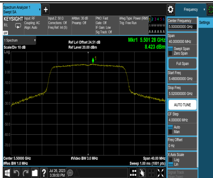
11AX20MIMO_Ant2_5500
