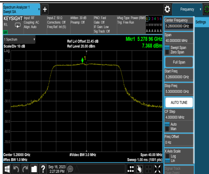
11AX20MIMO_Ant2_5280
