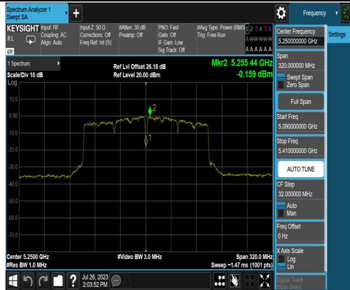
11AC160MIMO_Ant2_5250_UNII-2A
