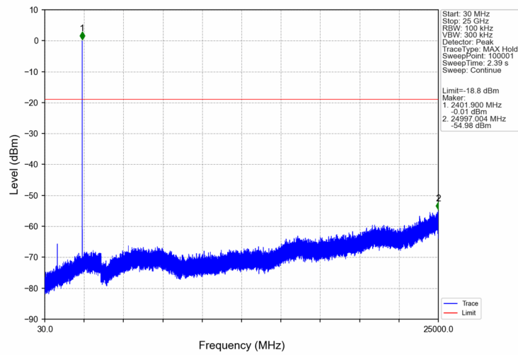
1M LCH 2402MHz Ant1 NTV
