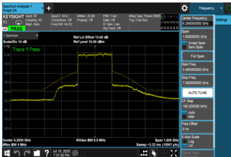
NTNV-11BE320MIMO-Ant0-6265-PASS
