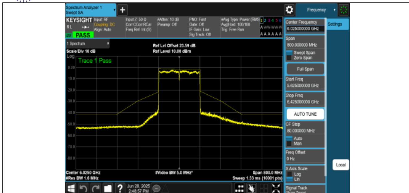
NTNV-11BE160MIMO-Ant1-6025-PASS
