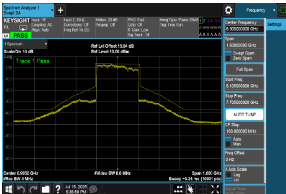
NTNV-11BE320MIMO-Ant0-6905-PASS
