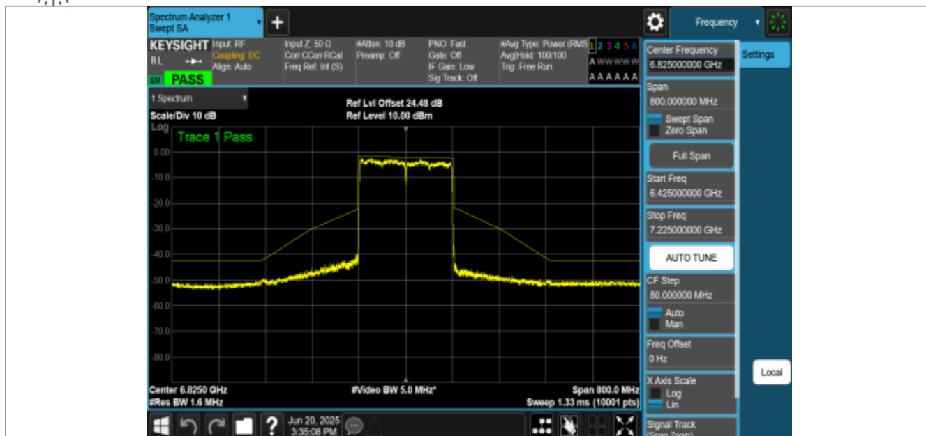
NTNV-11BE160MIMO-Ant1-6825-PASS
