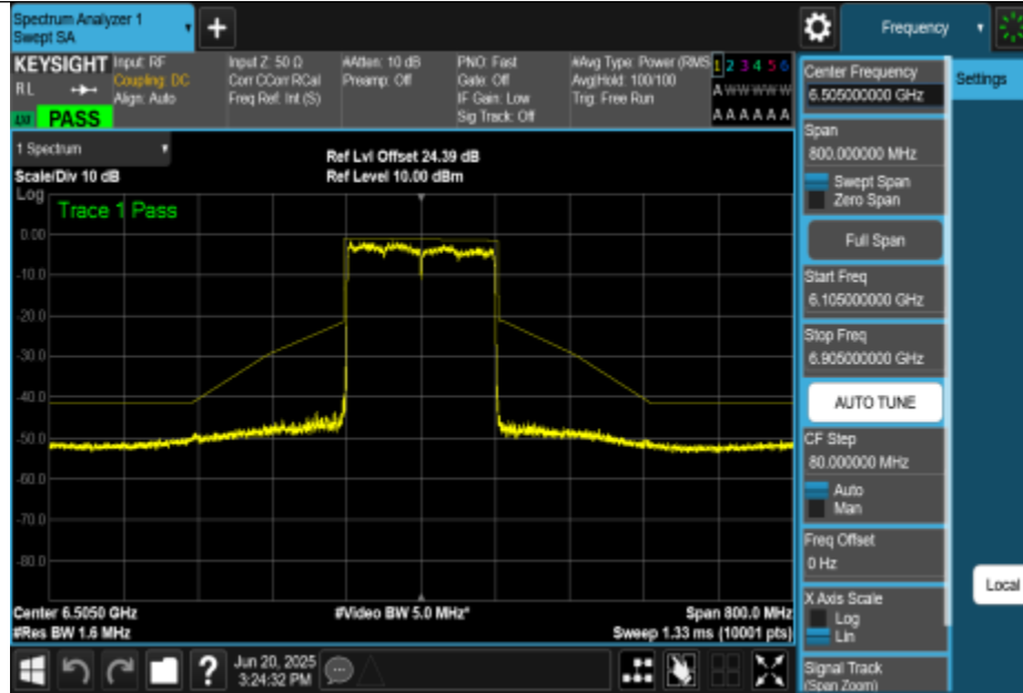
NTNV-11BE160MIMO-Ant1-6505-PASS
