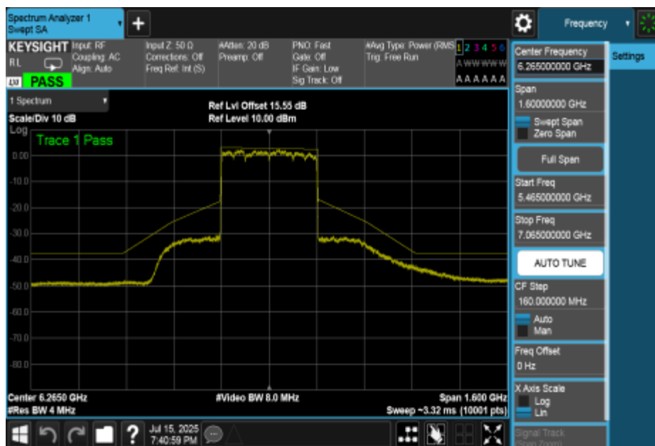
NTNV-11BE320MIMO-Ant1-6265-PASS
