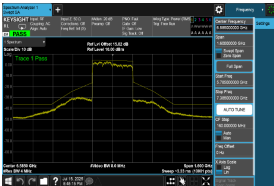
NTNV-11BE320MIMO-Ant1-6585-PASS
