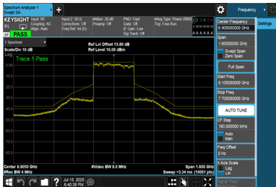
NTNV-11BE320MIMO-Ant1-6905-PASS
