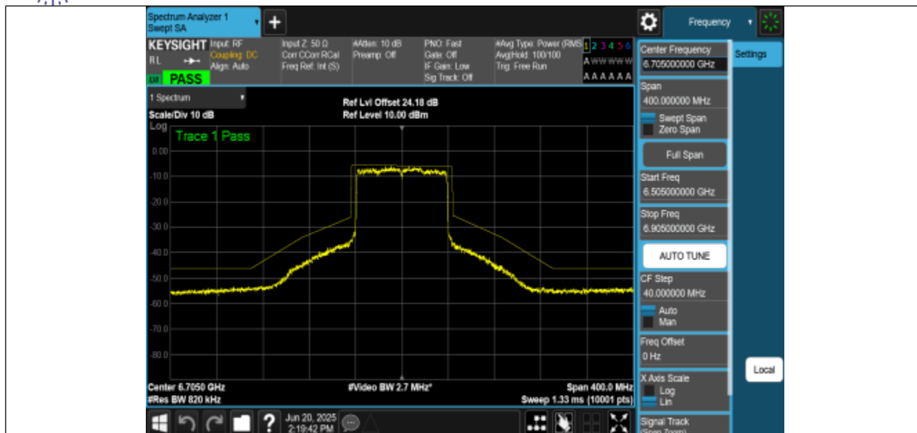
NTNV-11BE80MIMO-Ant1-6705-PASS
