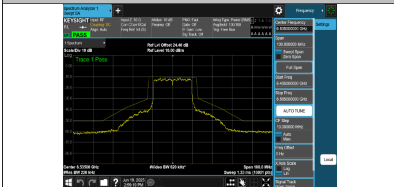
NTNV-11BE20MIMO-Ant1-6535-PASS
