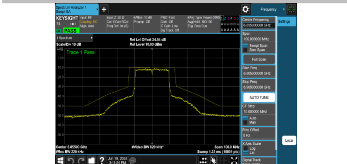
NTNV-11BE20MIMO-Ant1-6855-PASS
