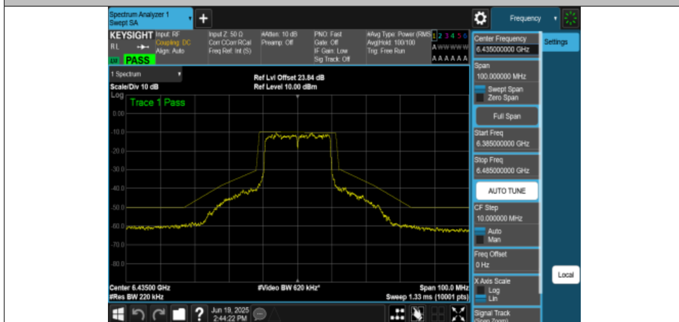
NTNV-11BE20MIMO-Ant1-6435-PASS
