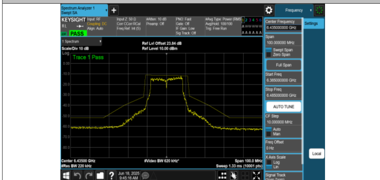
NTNV-11A-CDD-Ant1-6435-PASS
