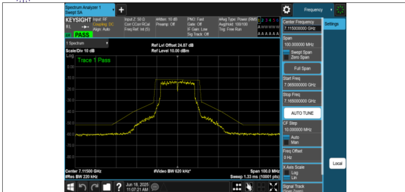
NTNV-11A-CDD-Ant0-7115-PASS
