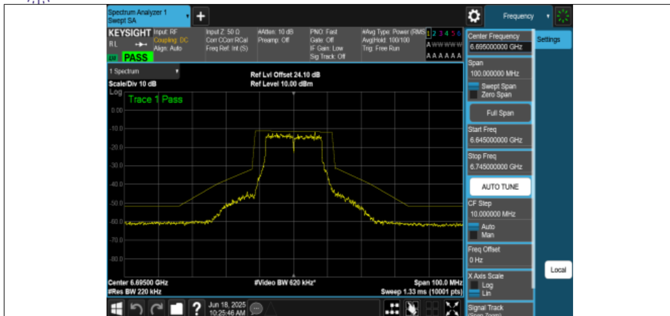
NTNV-11A-CDD-Ant0-6695-PASS
