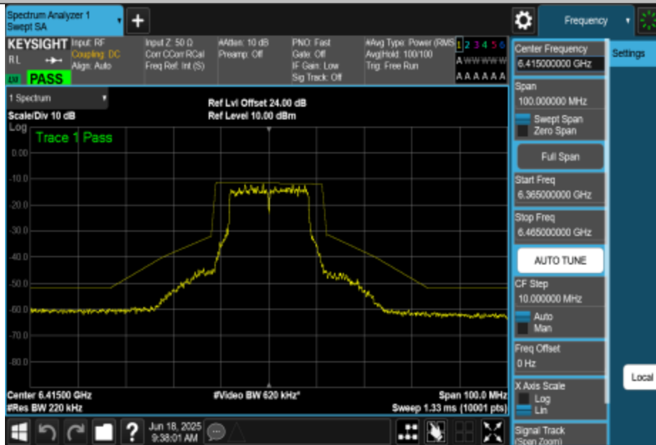
NTNV-11A-CDD-Ant1-6415-PASS
