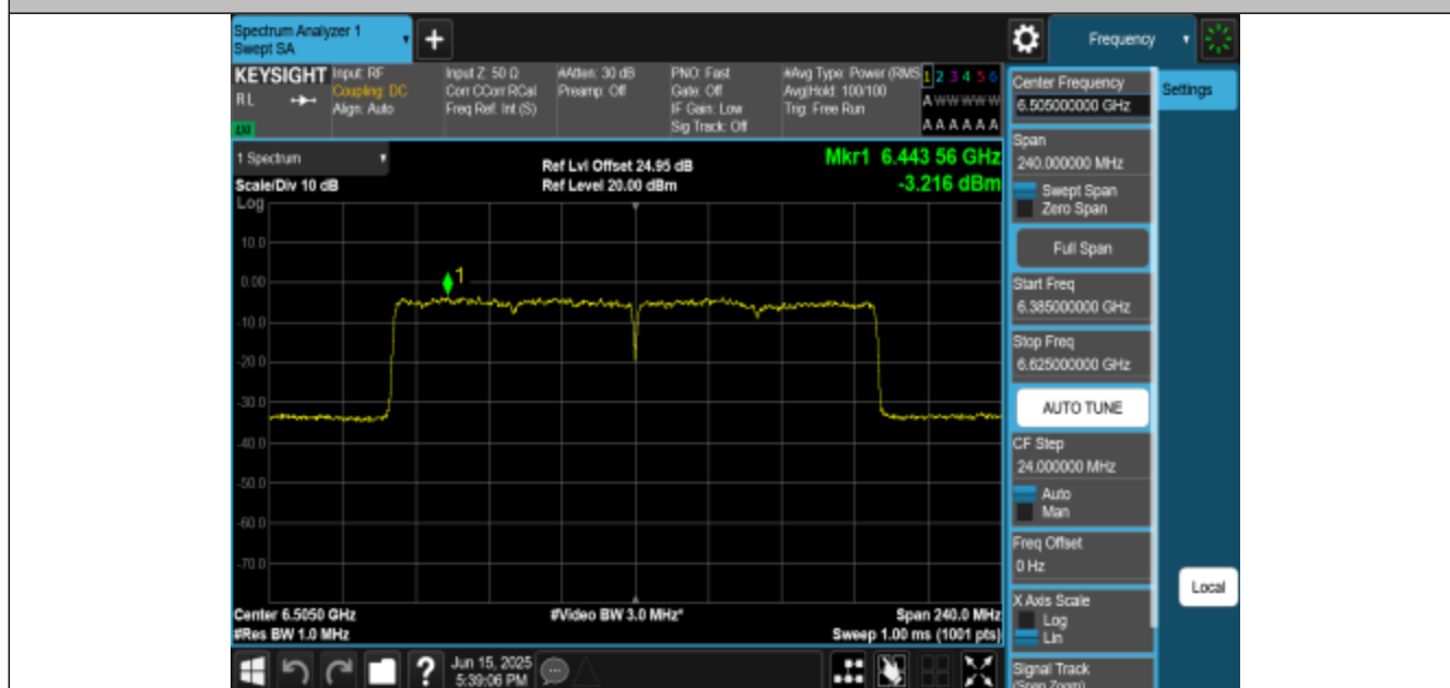
11BE160MIMO-Ant1-6505-PASS
