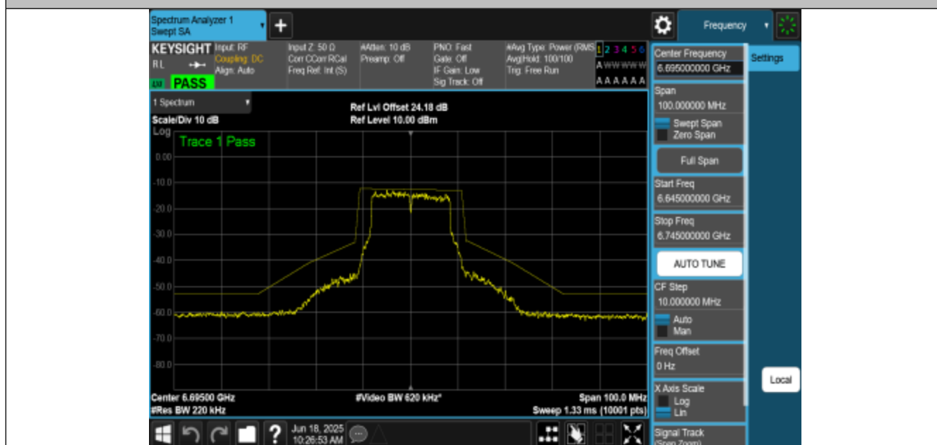
NTNV-11A-CDD-Ant1-6695-PASS
