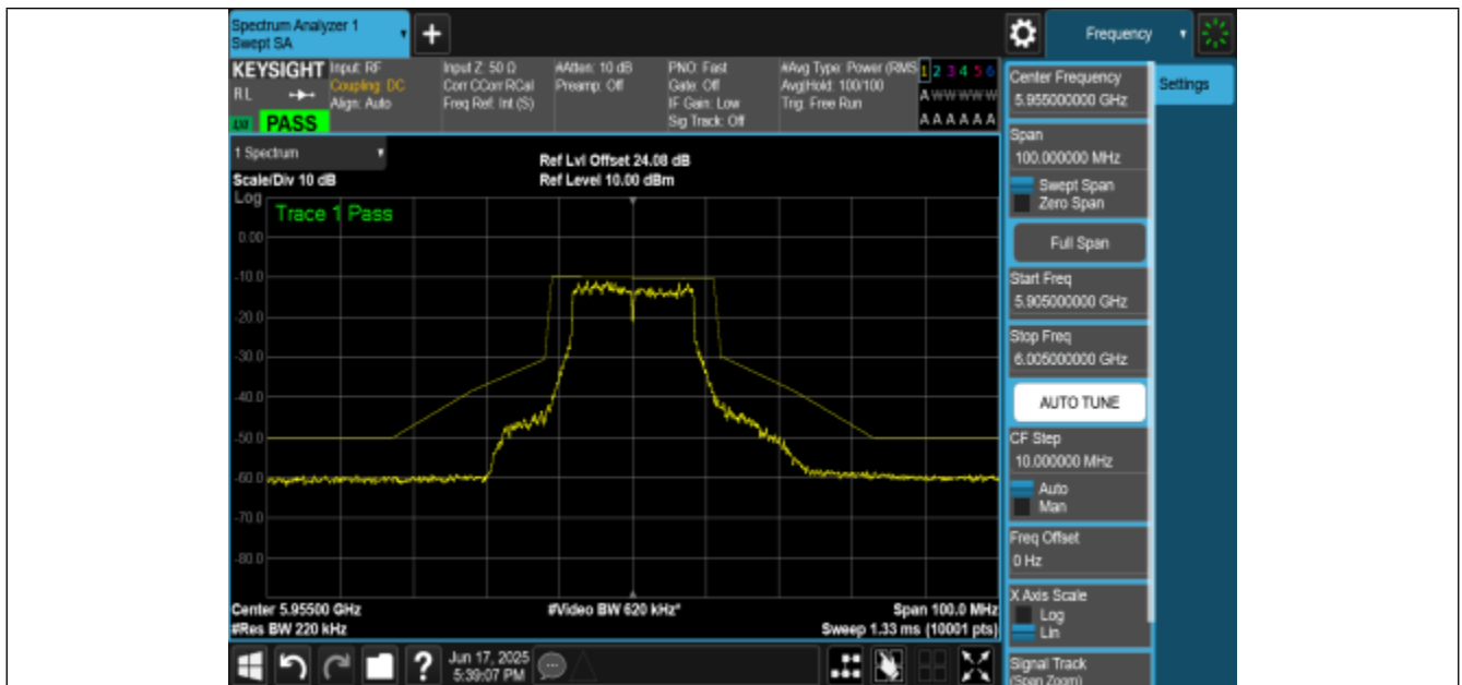
NTVN-11A-CDD-Ant0-5955-PASS
