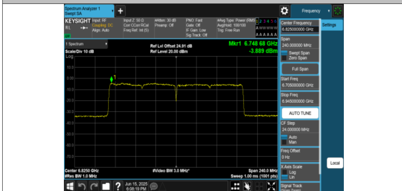
11BE160MIMO-Ant1-6825-PASS
