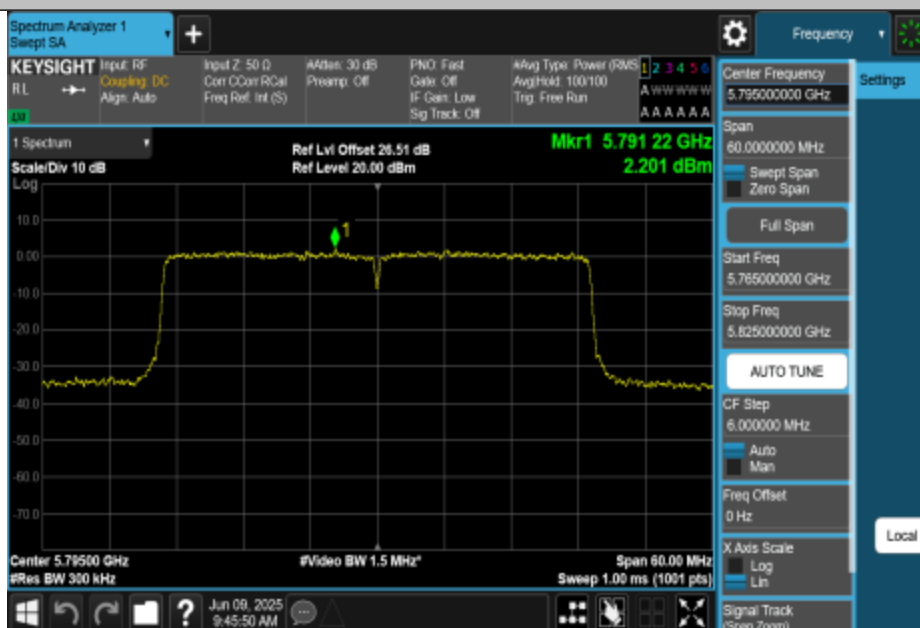
11AX40MIMO-Ant3-5795-PASS
