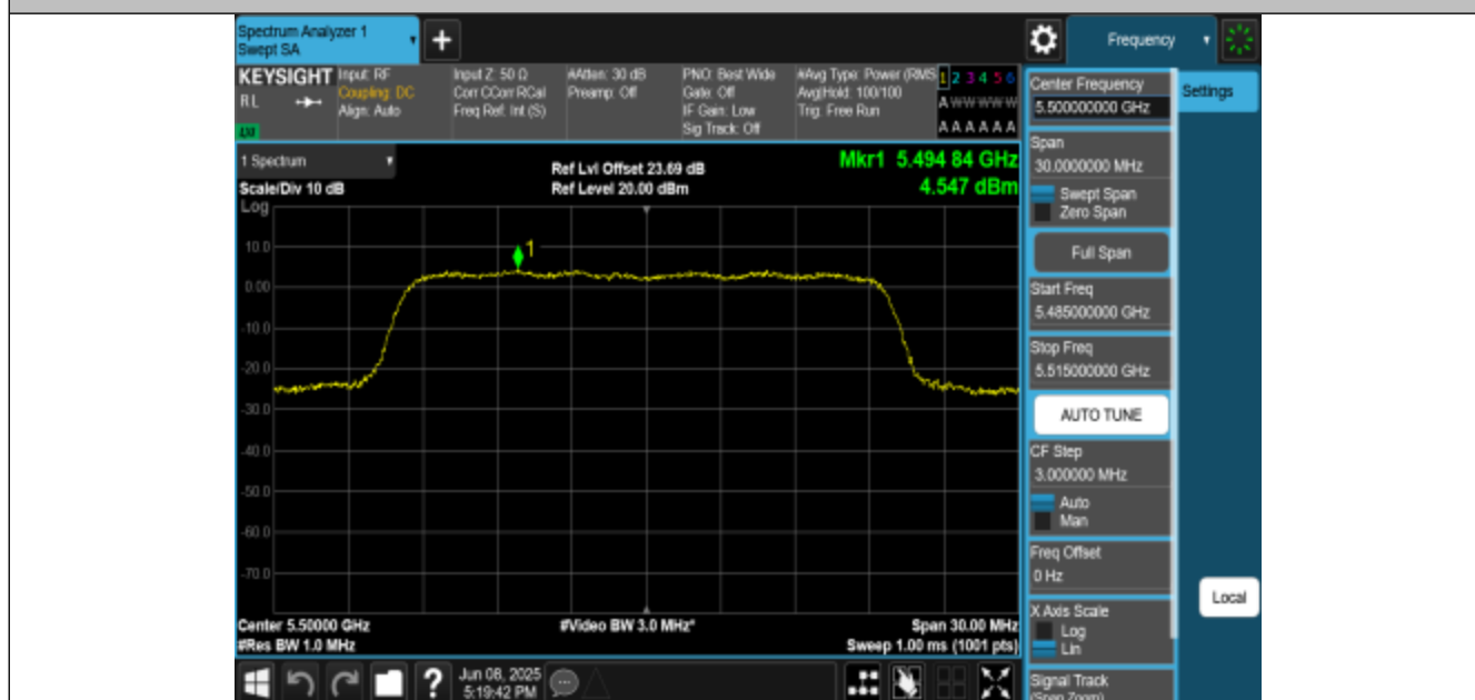
11AX20MIMO-Ant1-5500-PASS
