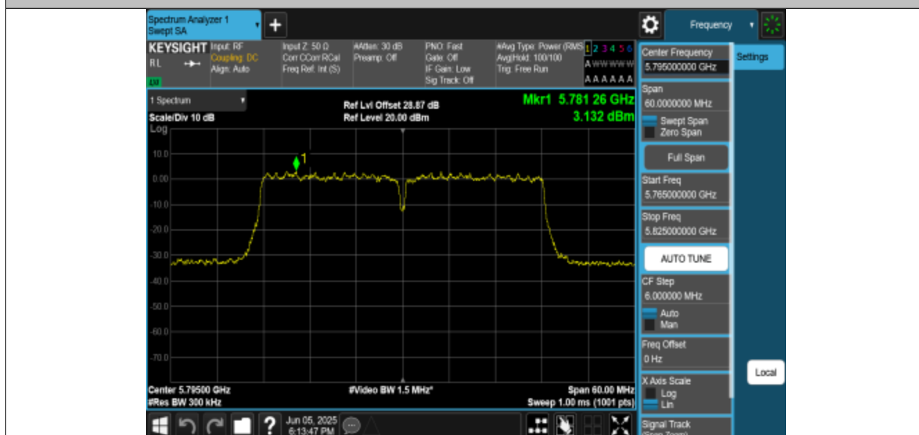
11N40MIMO-Ant1-5795-PASS
