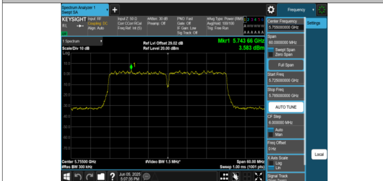
11N40MIMO-Ant1-5755-PASS
