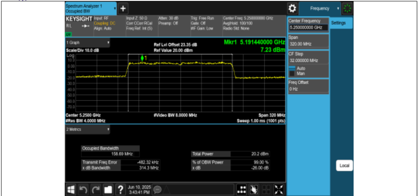
11BE160MIMO-Ant0-5250
