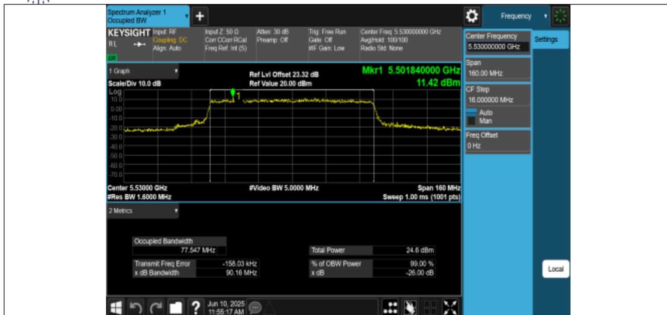
11BE80MIMO-Ant0-5530
