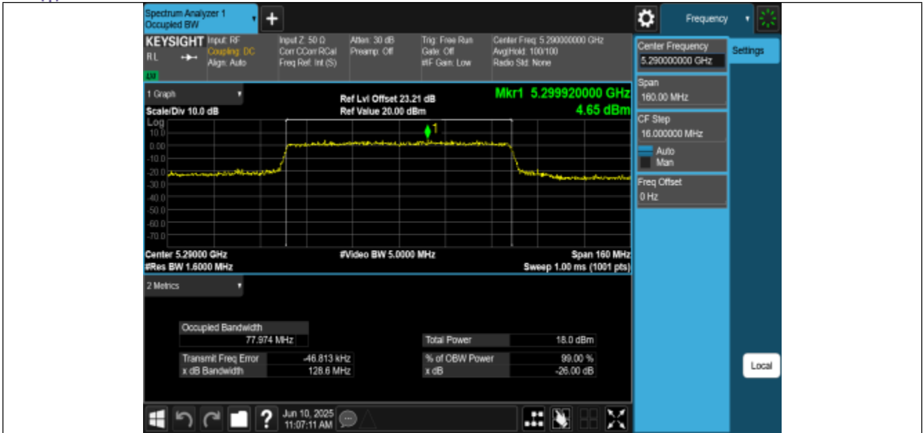
11BE80MIMO-Ant0-5290
