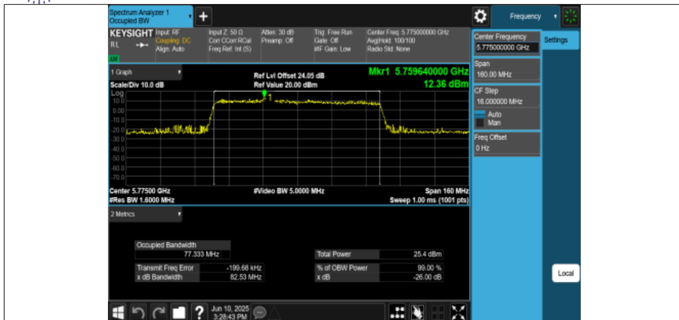
11BE80MIMO-Ant0-5775
