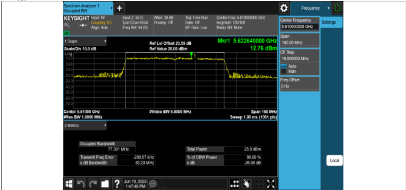
11BE80MIMO-Ant0-5610
