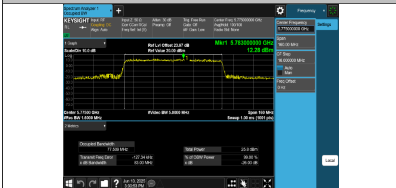
11BE80MIMO-Ant1-5775
