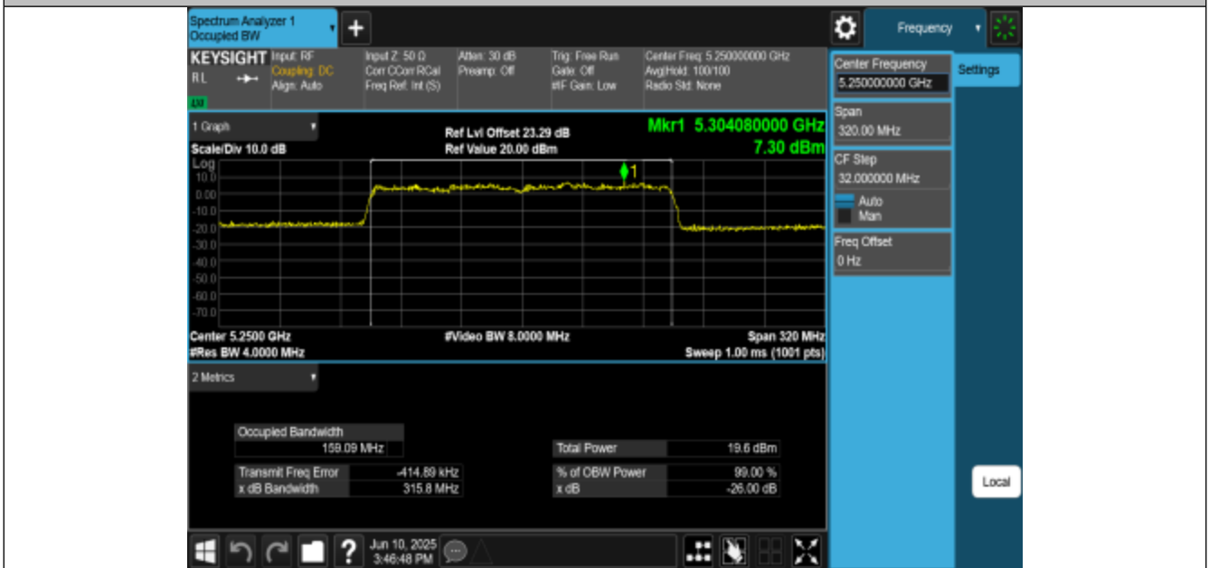
11BE160MIMO-Ant3-5250
