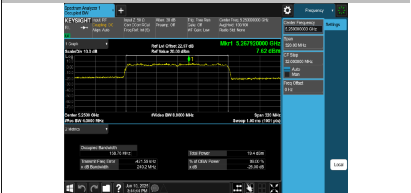
11BE160MIMO-Ant1-5250
