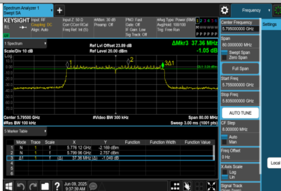
11AX40MIMO-Ant3-5795-PASS
