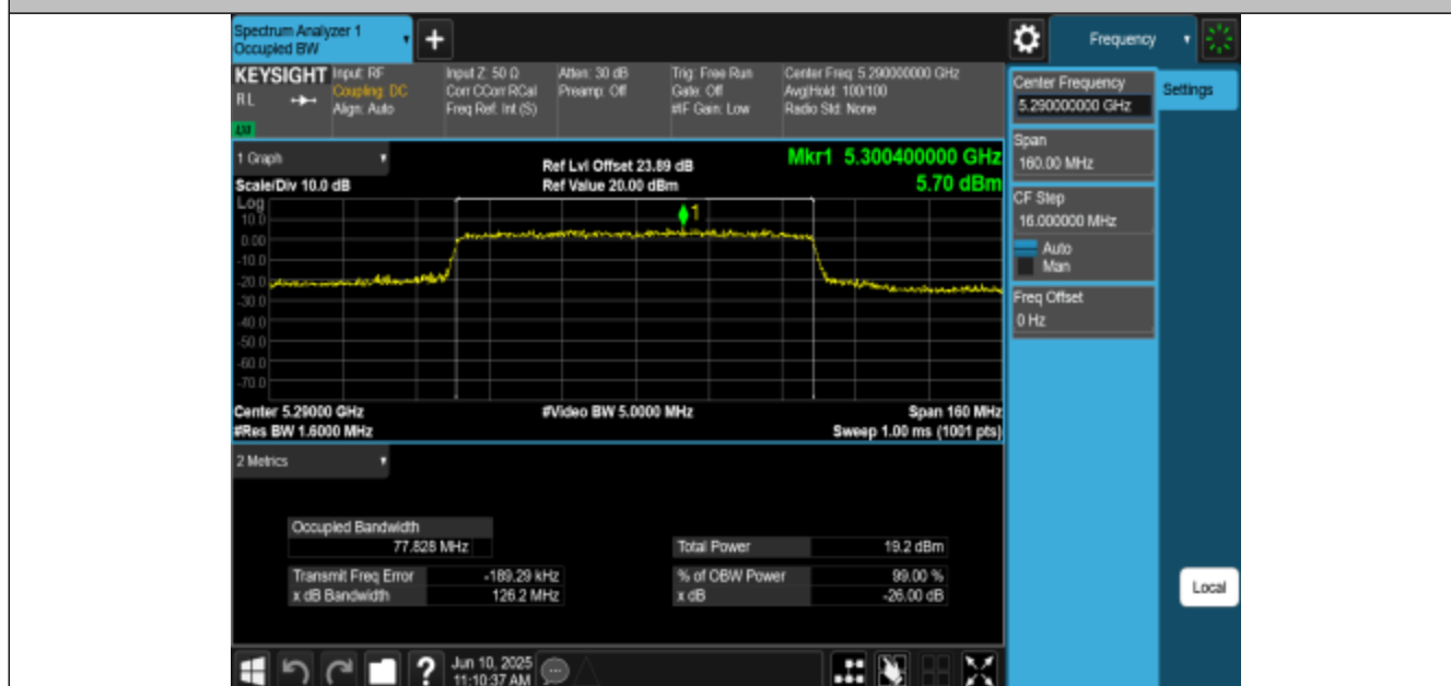
11BE80MIMO-Ant3-5290
