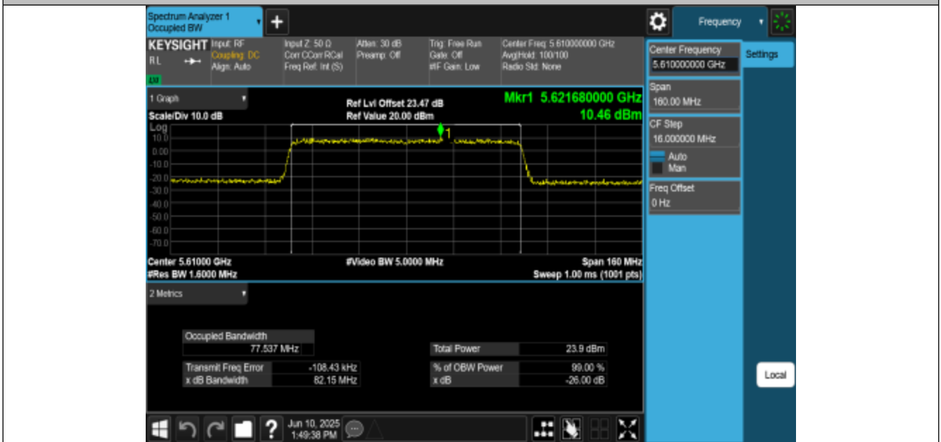
11BE80MIMO-Ant1-5610
