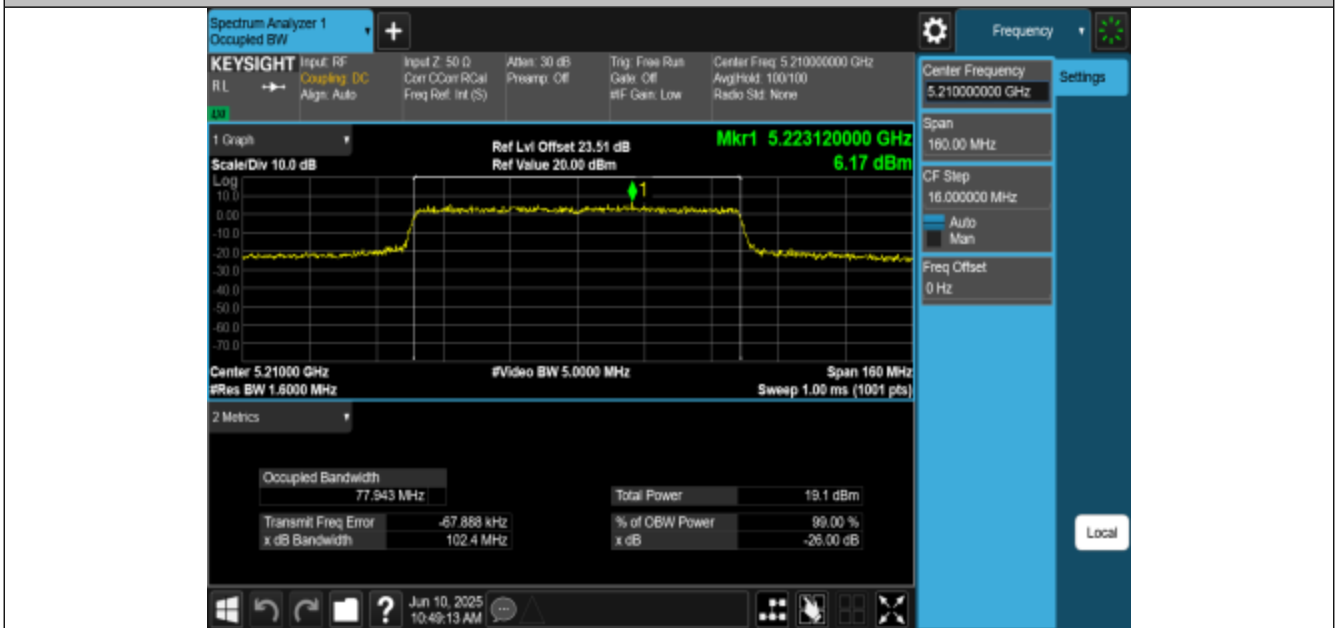
11BE80MIMO-Ant1-5210
