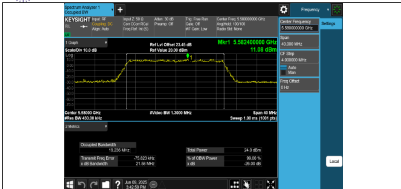
11BE20MIMO-Ant0-5580
