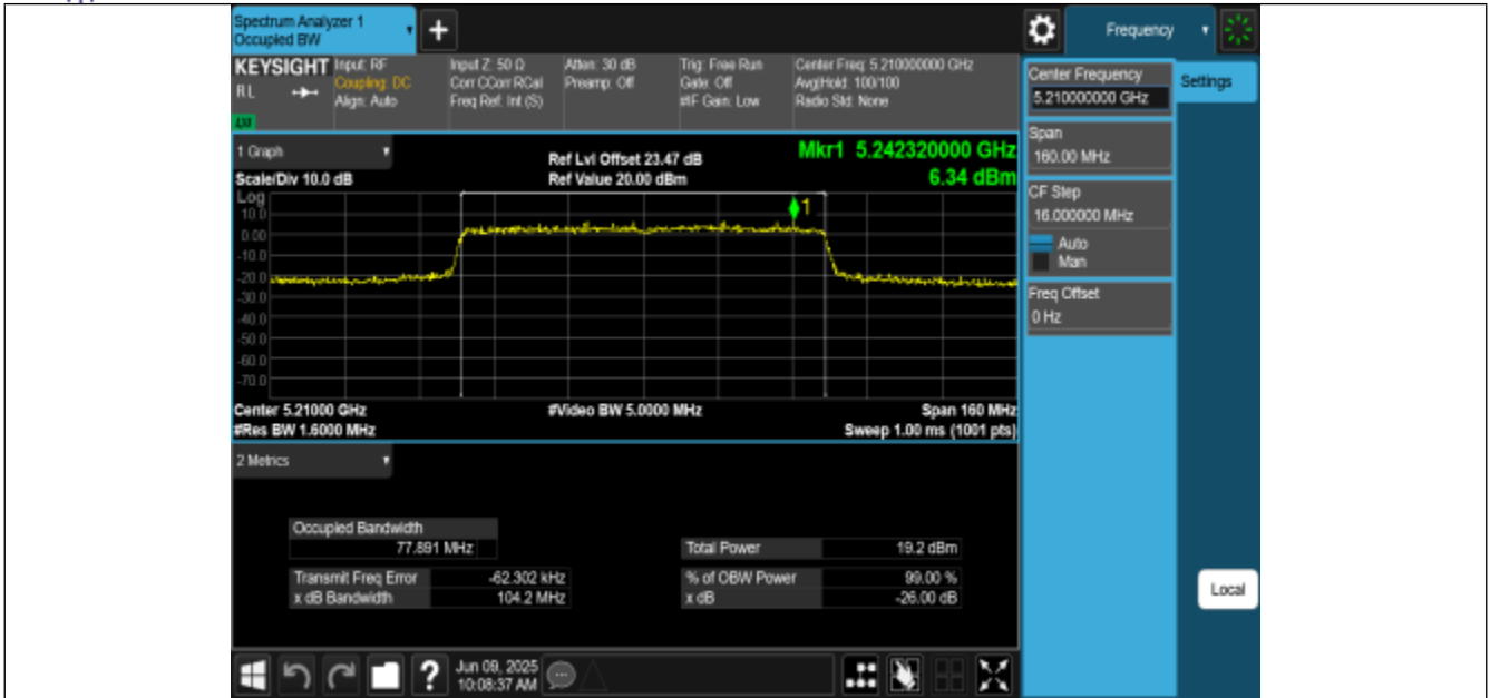
11AX80MIMO-Ant2-5210
