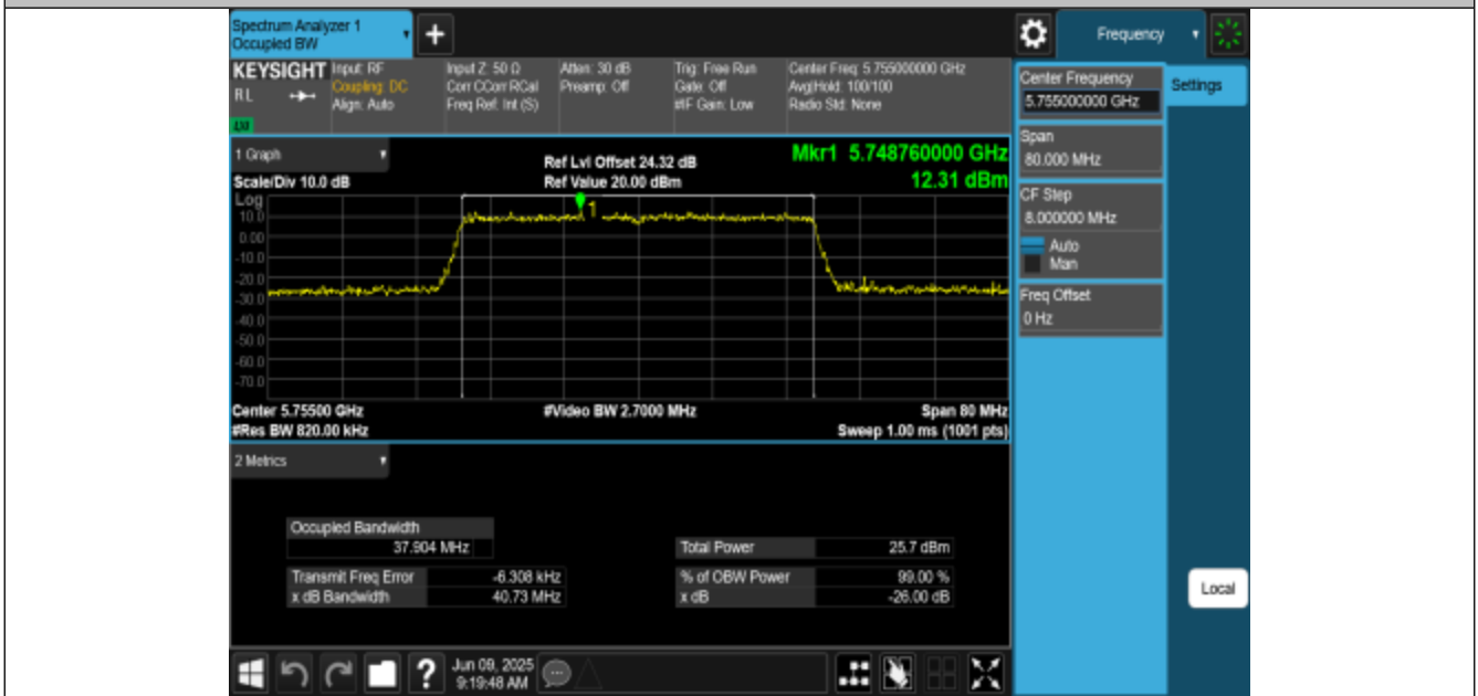
11AX40MIMO-Ant3-5755
