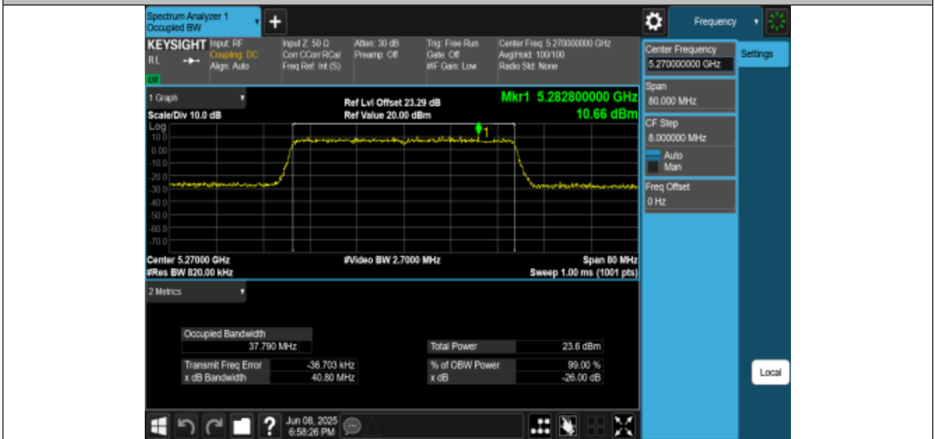
11AX40MIMO-Ant3-5270
