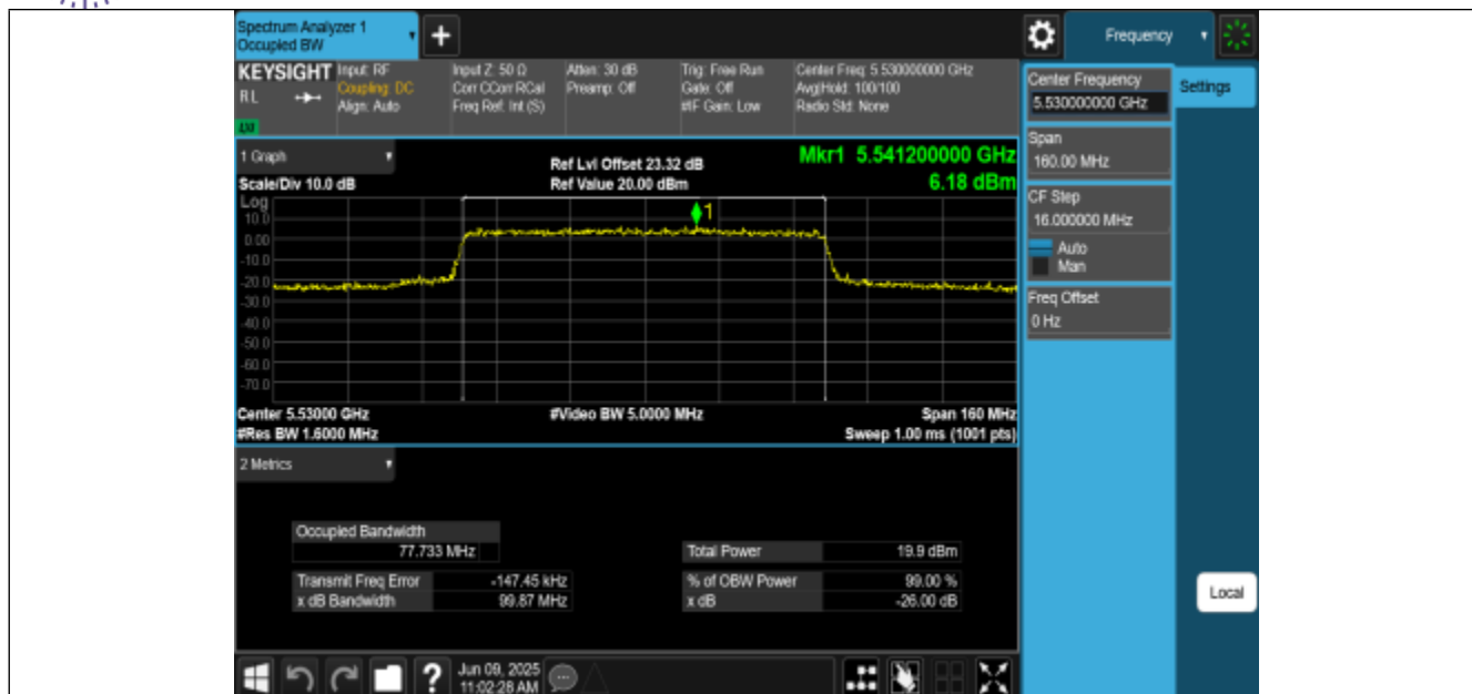
11AX80MIMO-Ant0-5530
