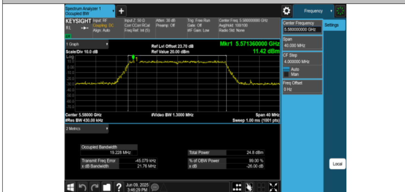
11BE20MIMO-Ant3-5580
