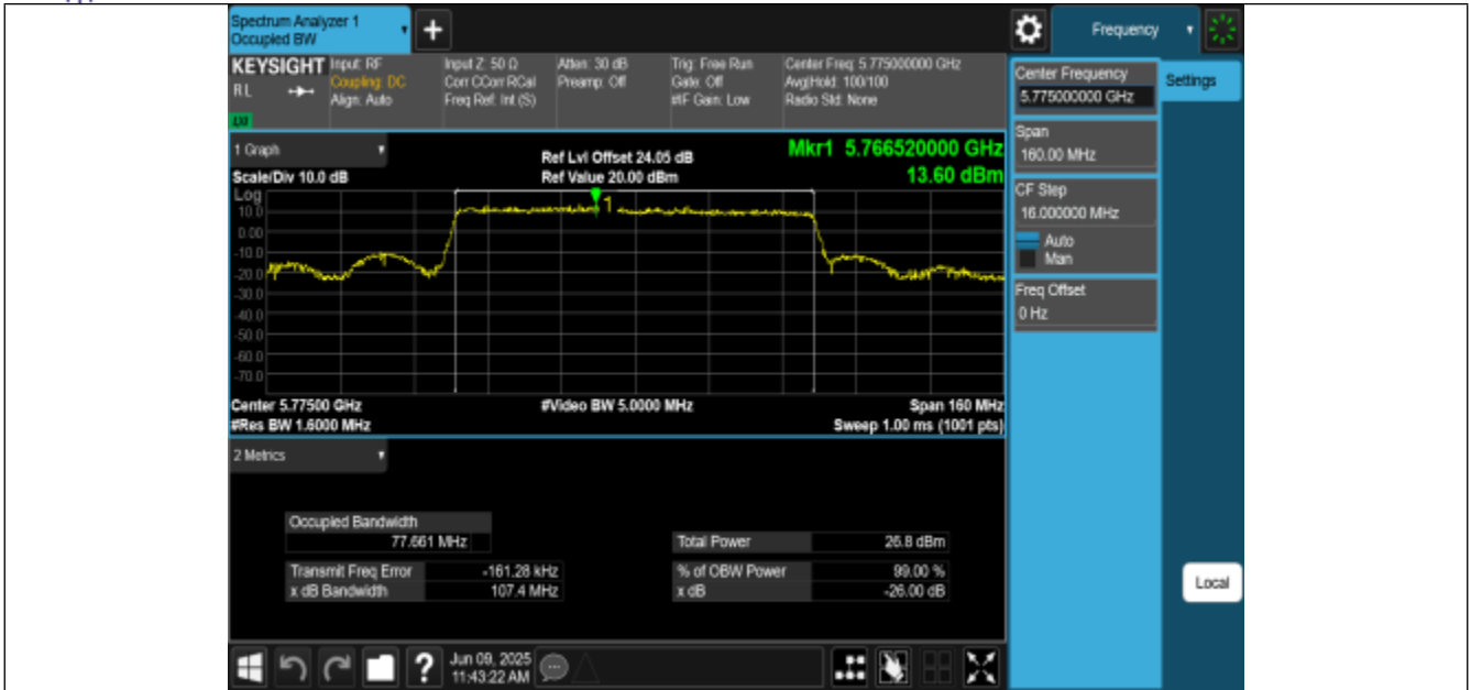
11AX80MIMO-Ant0-5775
