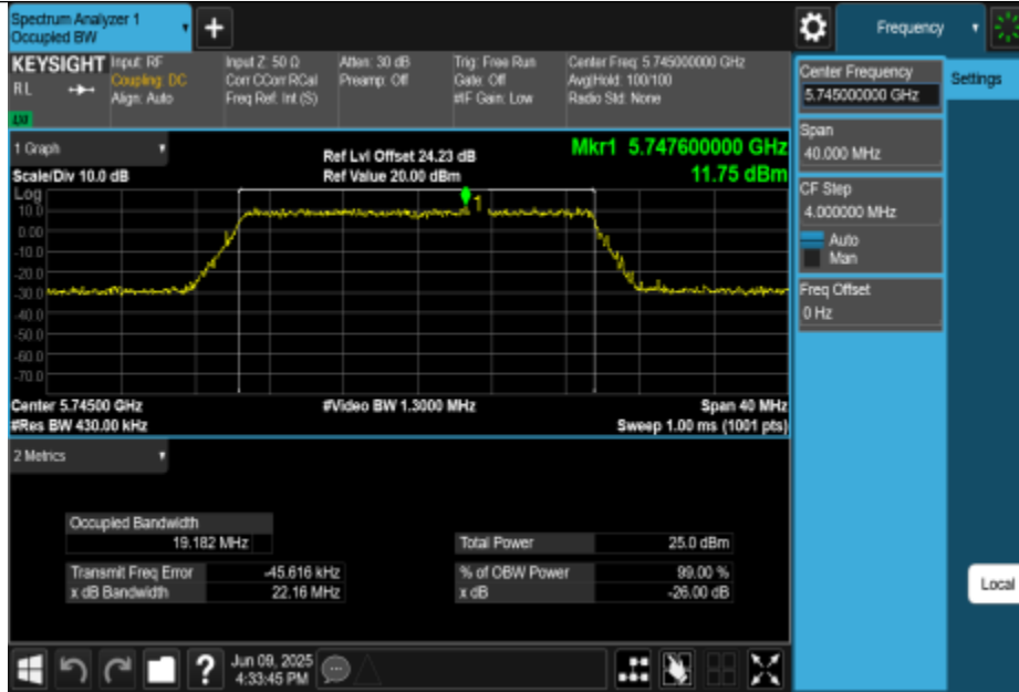
11BE20MIMO-Ant2-5745
