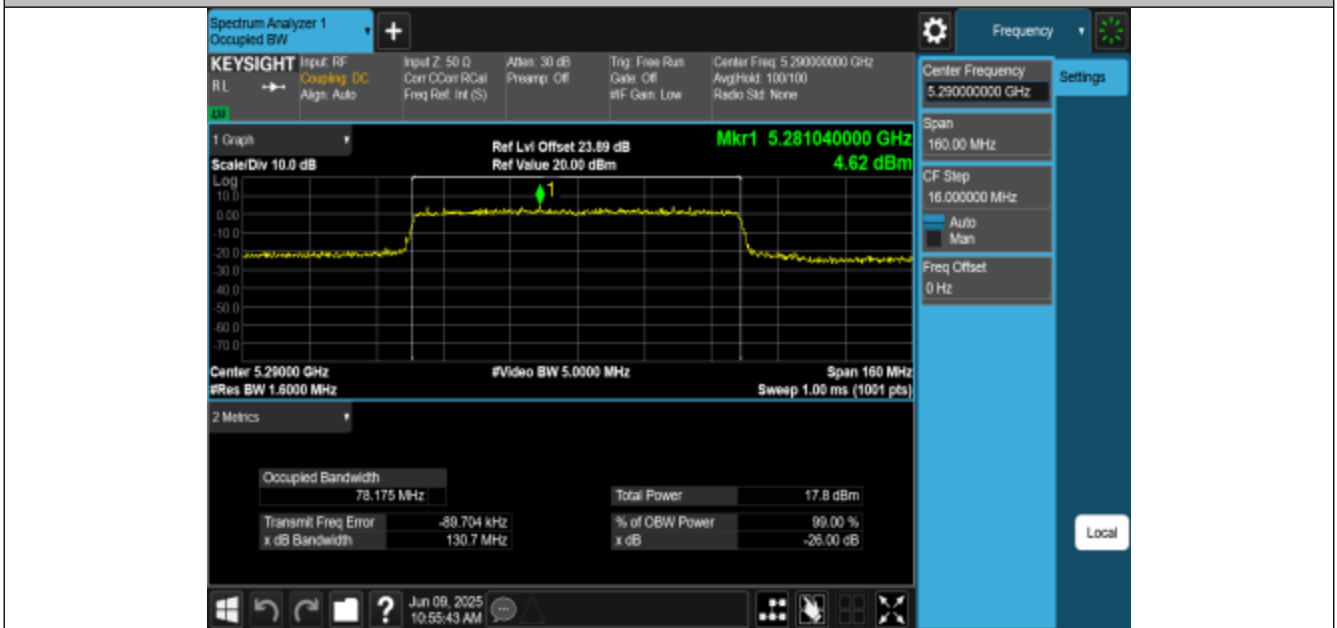
11AX80MIMO-Ant3-5290
