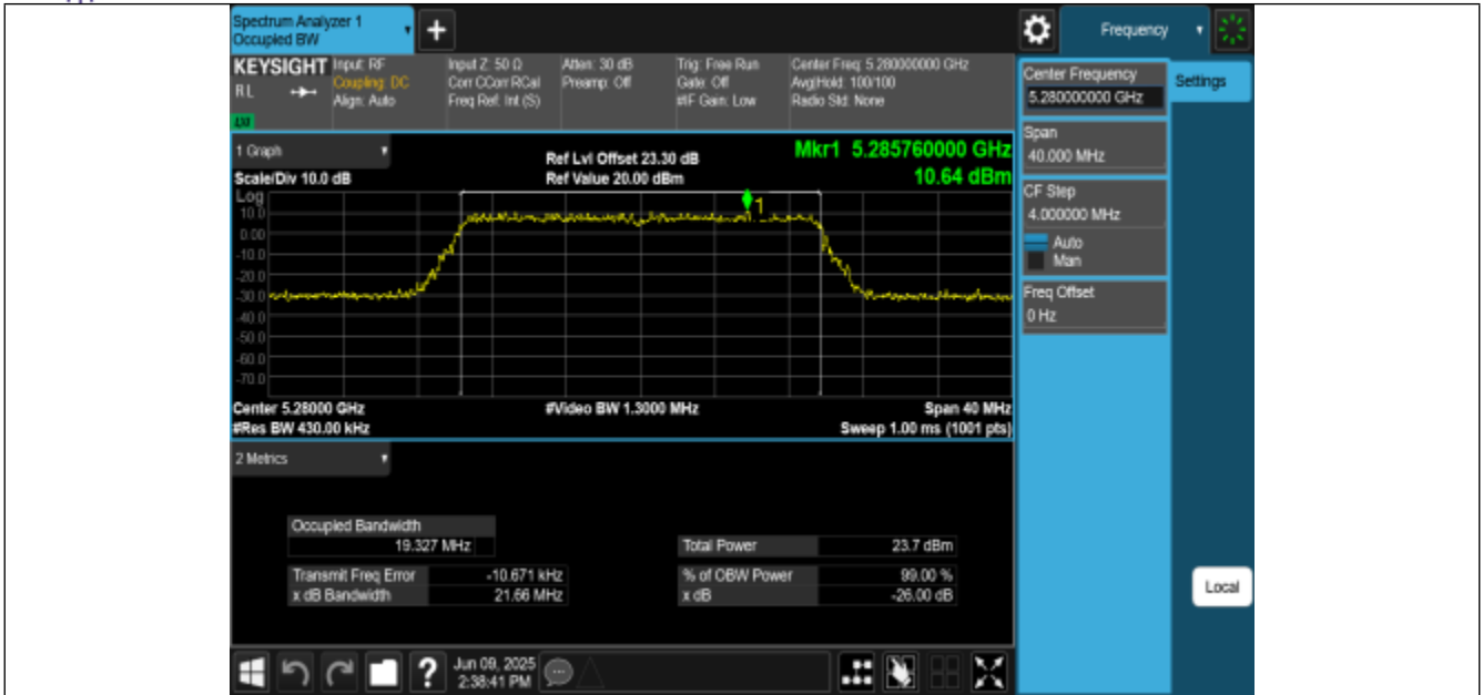
11BE20MIMO-Ant0-5280
