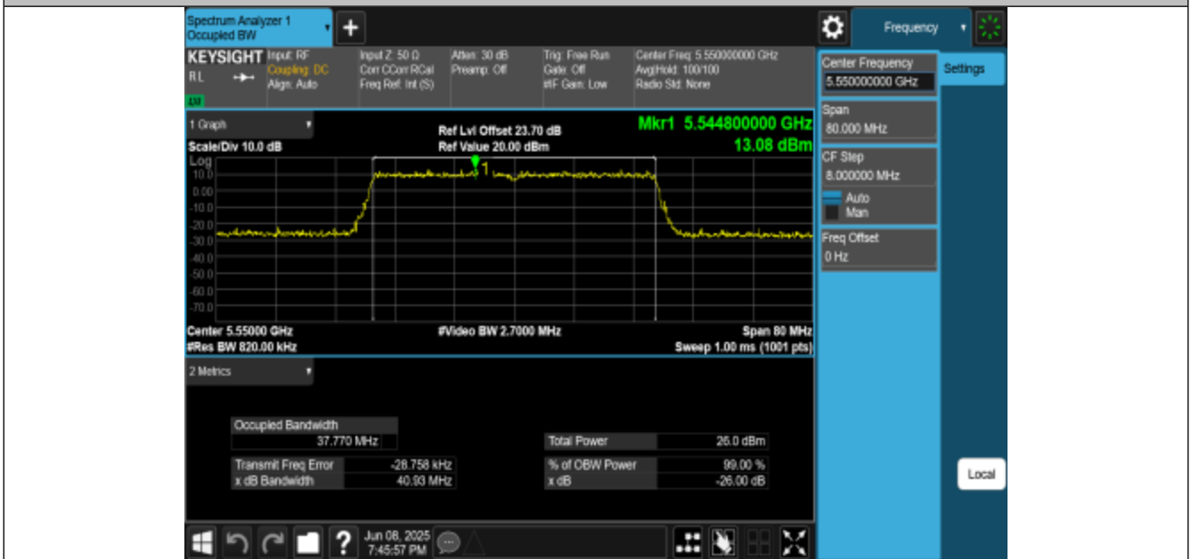
11AX40MIMO-Ant3-5550
