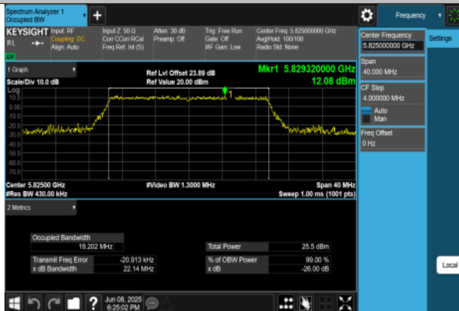
11AX20MIMO-Ant3-5825
