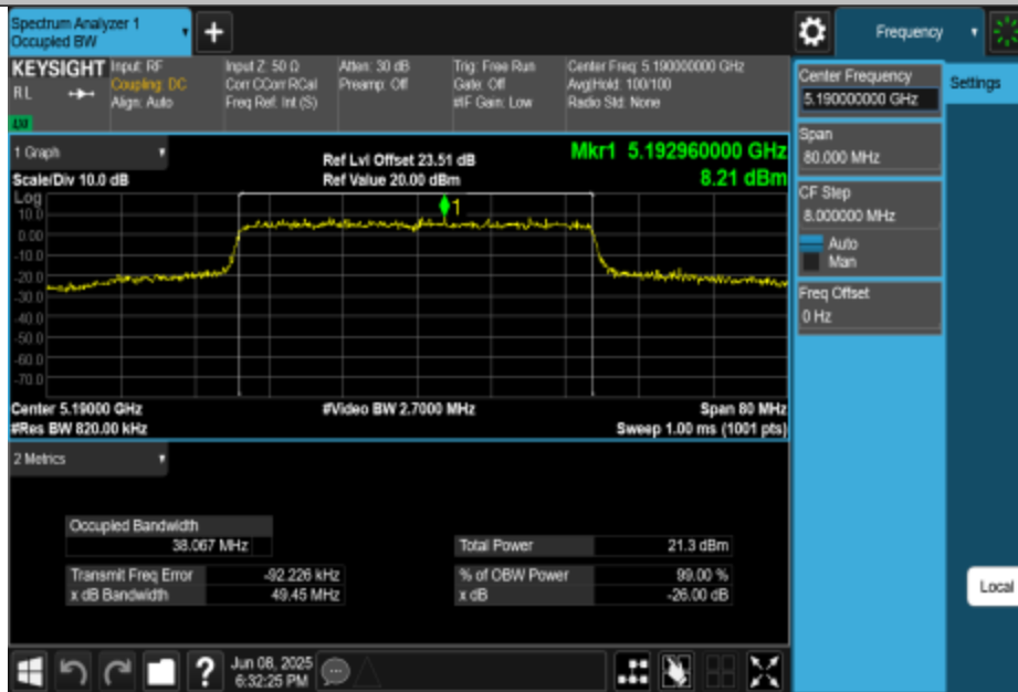
11AX40MIMO-Ant1-5190
