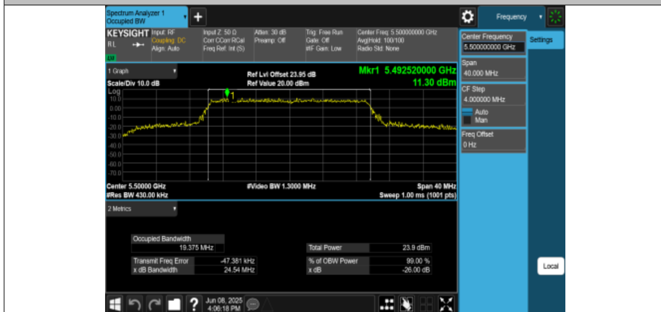
11AX20MIMO-Ant3-5500
