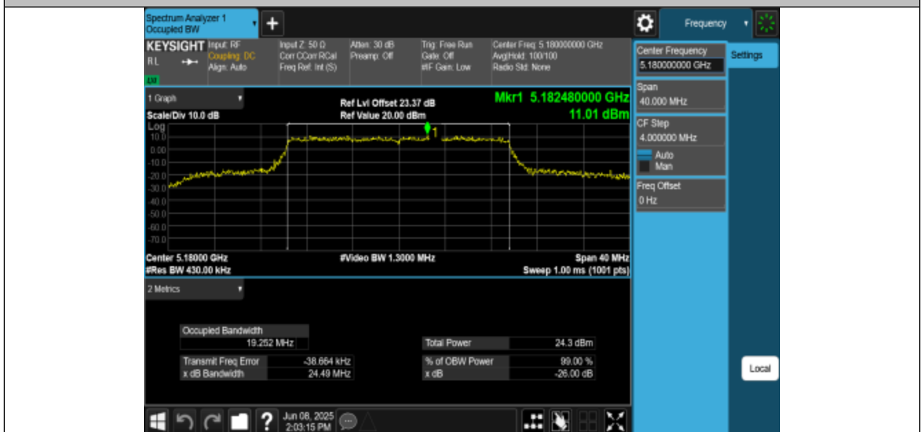
11AX20MIMO-Ant1-5180
