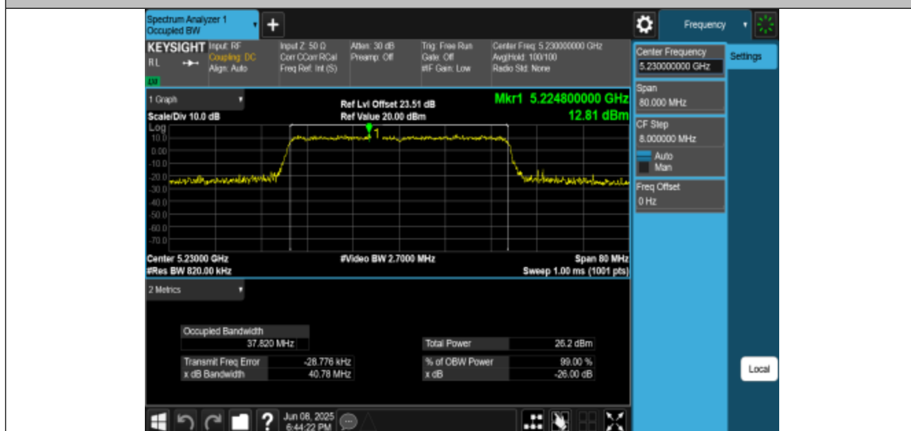
11AX40MIMO-Ant1-5230
