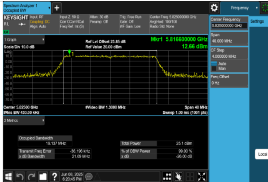
11AX20MIMO-Ant2-5825
