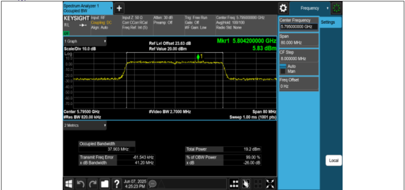
11AC40MIMO-Ant0-5795
