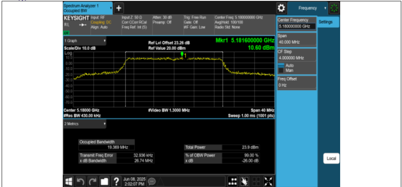
11AX20MIMO-Ant0-5180
