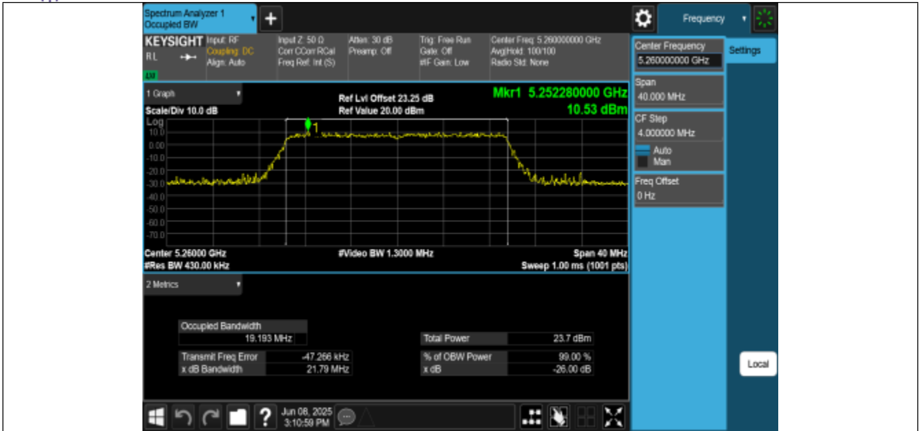
11AX20MIMO-Ant2-5260
