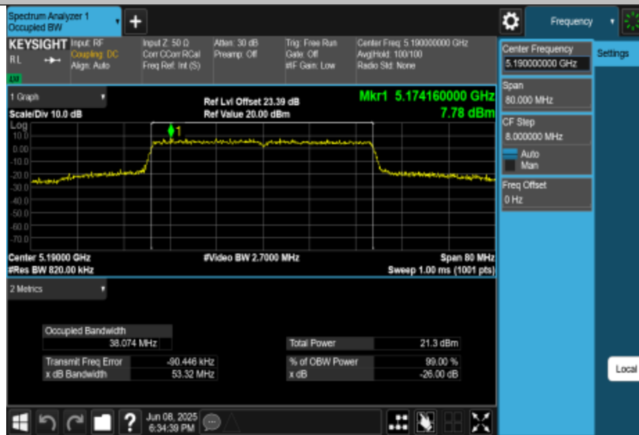
11AX40MIMO-Ant3-5190
