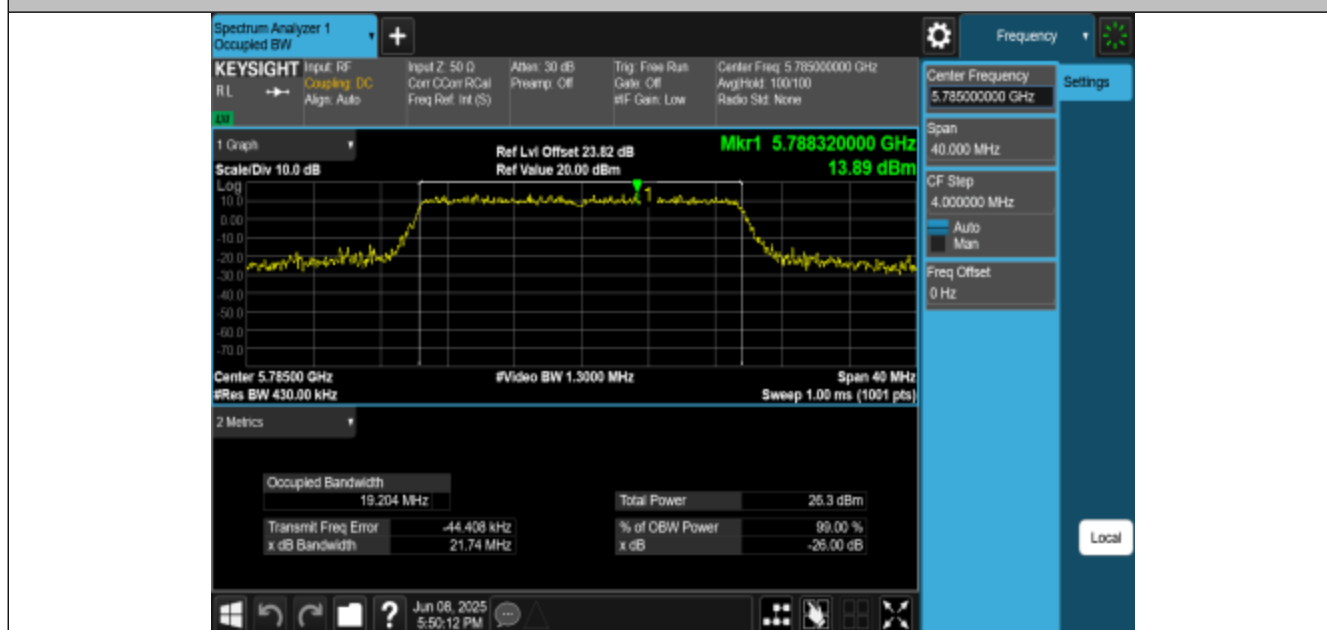
11AX20MIMO-Ant1-5785
