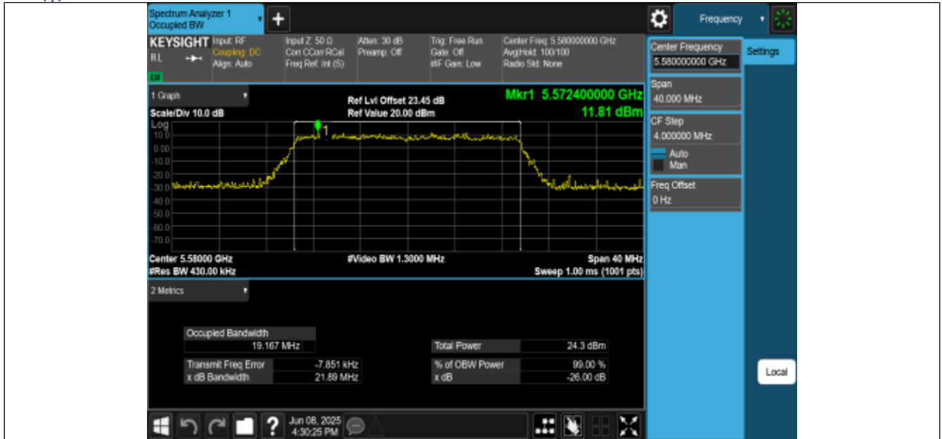
11AX20MIMO-Ant0-5580
