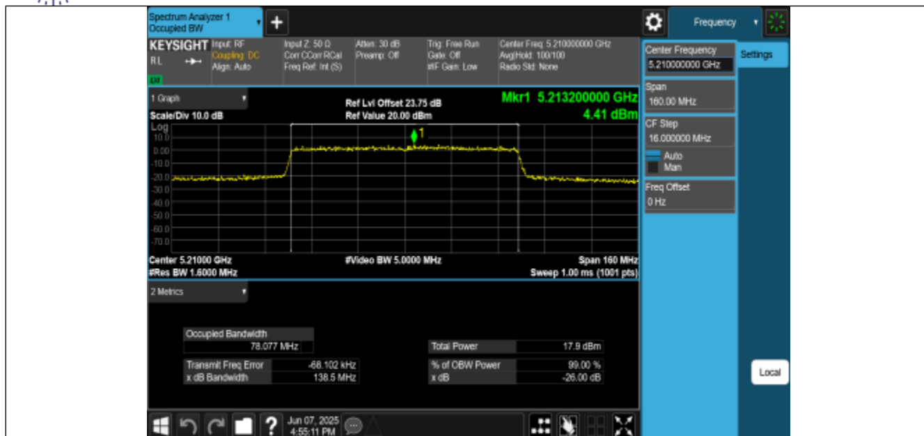
11AC80MIMO-Ant0-5210
