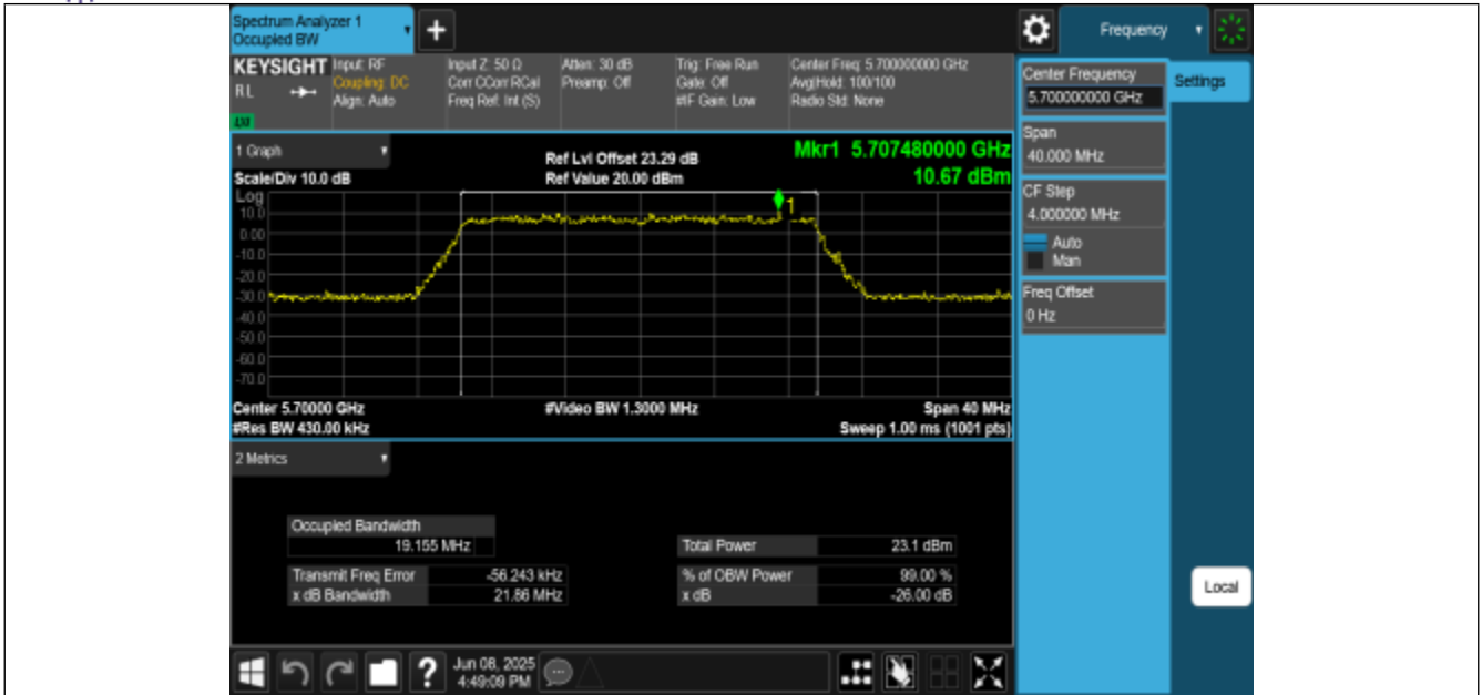
11AX20MIMO-Ant0-5700
