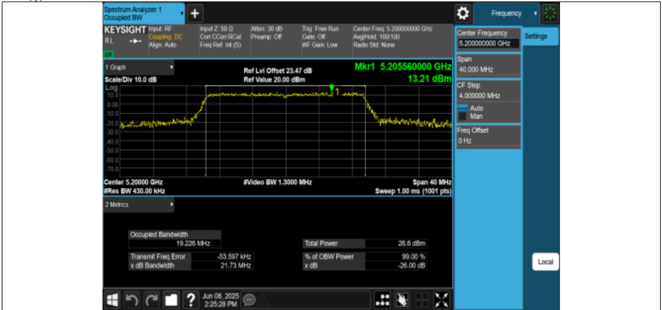
11AX20MIMO-Ant2-5200
