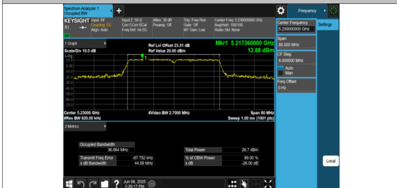
11AC40MIMO-Ant1-5230
