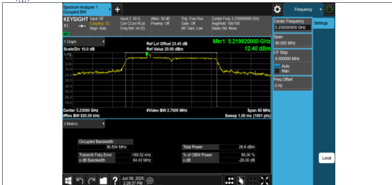
11AC40MIMO-Ant0-5230
