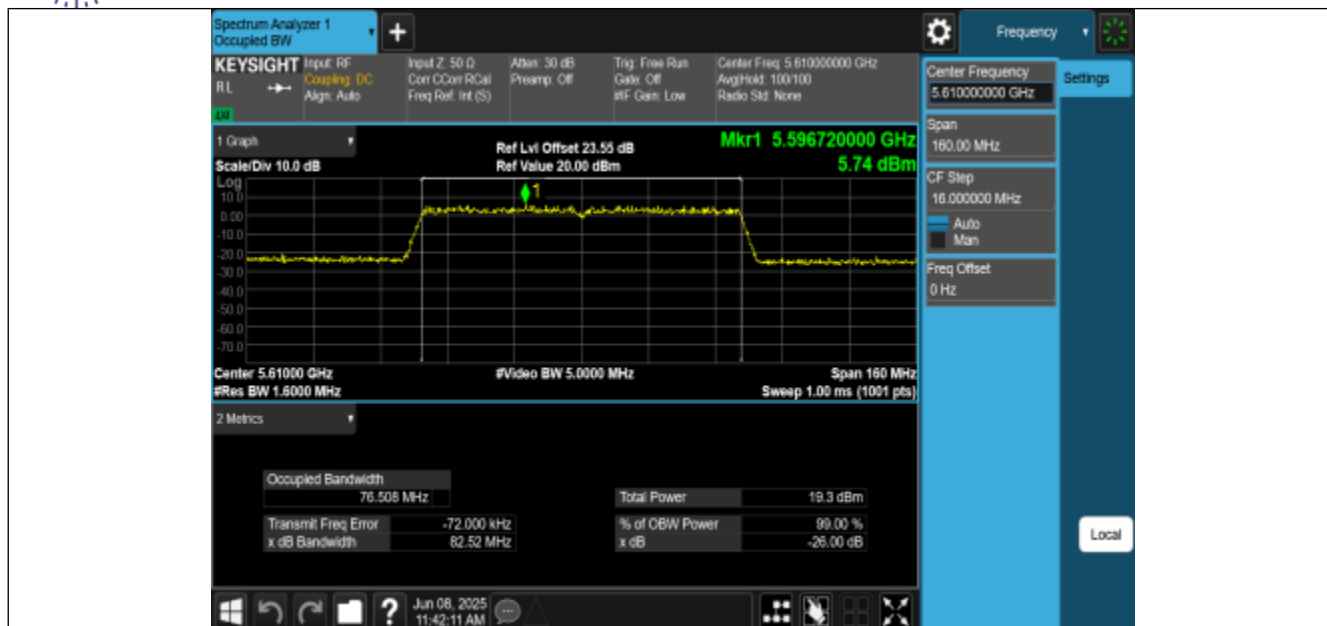
11AC80MIMO-Ant0-5610
