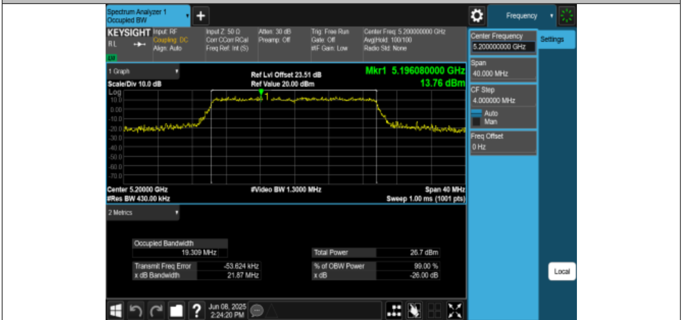
11AX20MIMO-Ant1-5200
