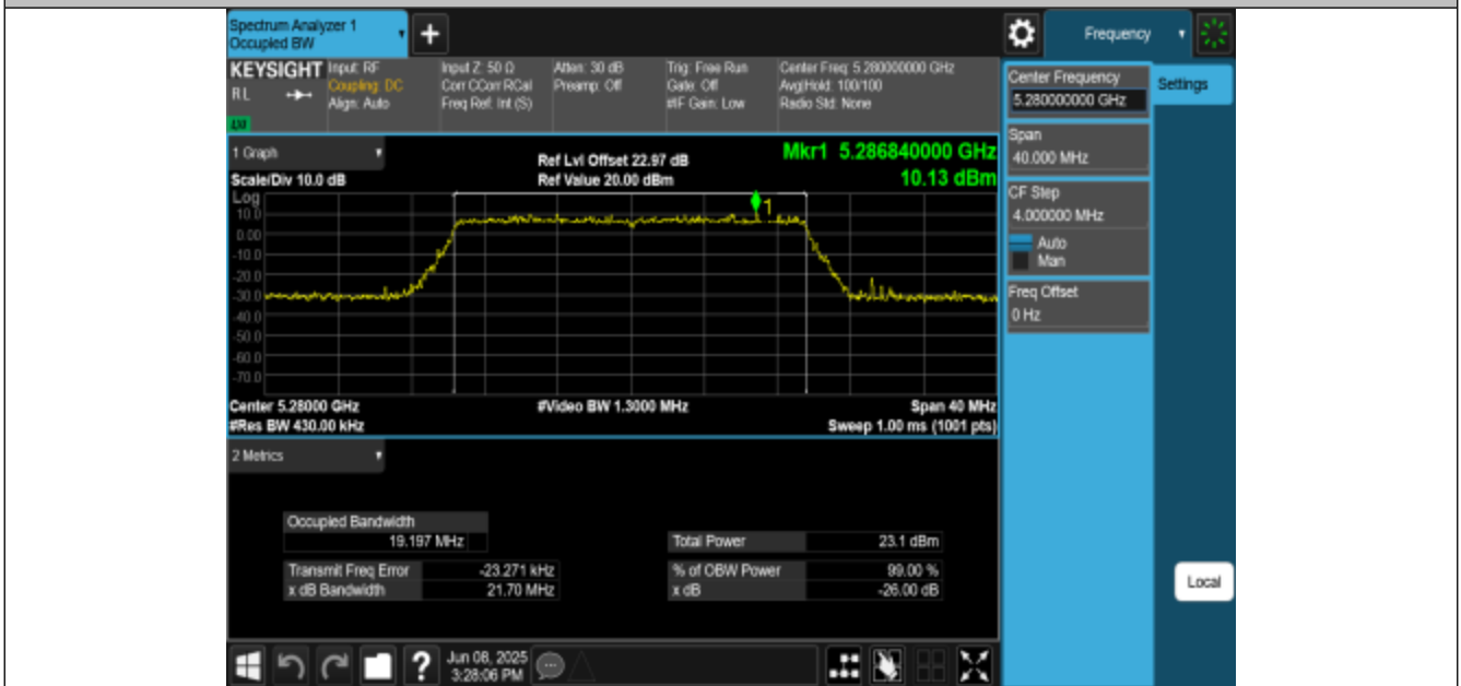
11AX20MIMO-Ant1-5280
