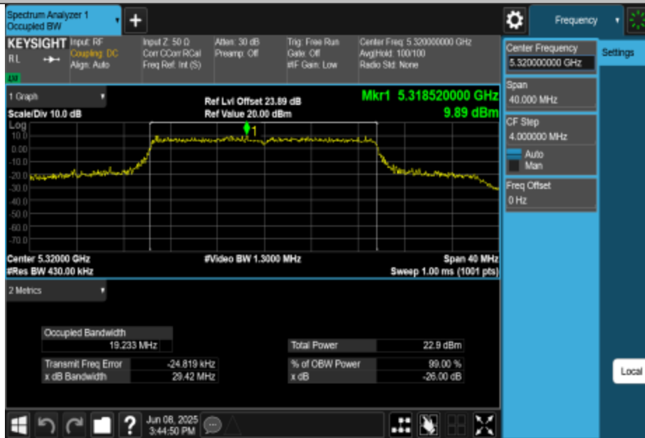
11AX20MIMO-Ant3-5320
