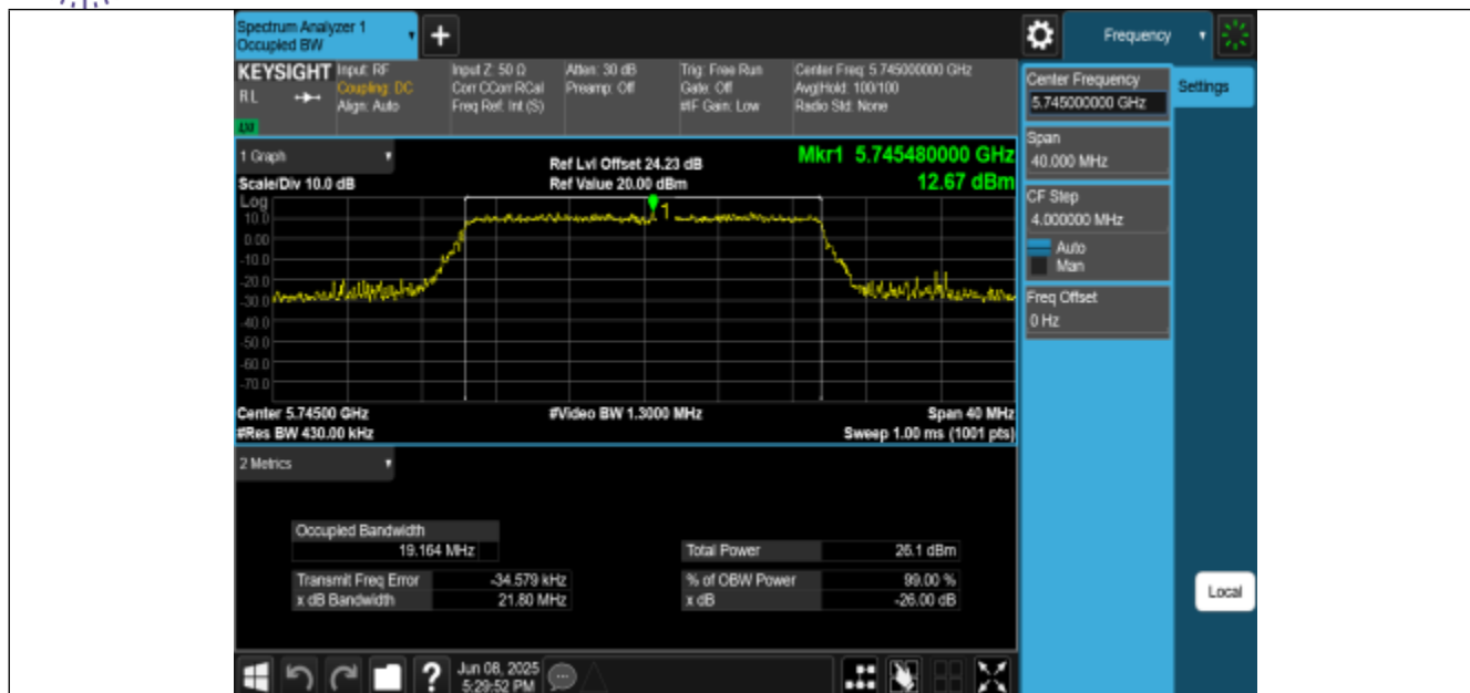
11AX20MIMO-Ant2-5745
