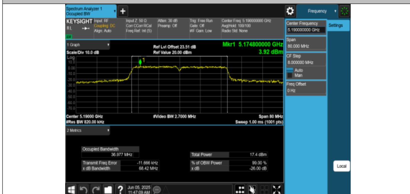
11N40MIMO-Ant1-5190
