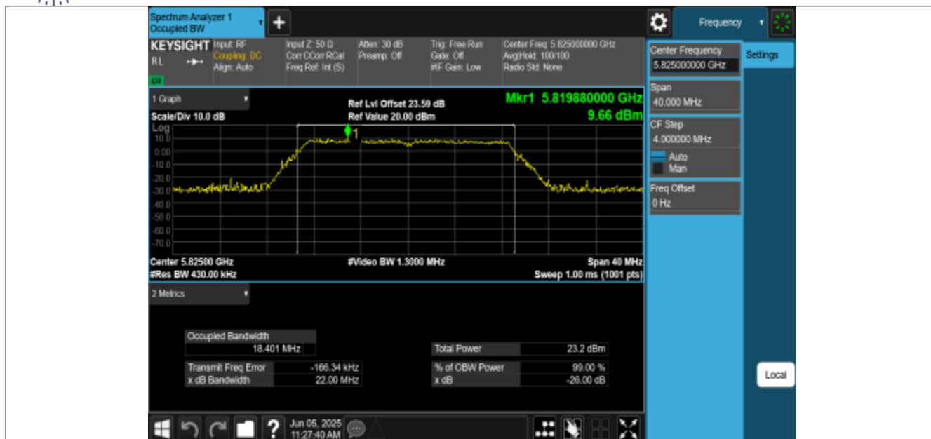
11N20MIMO-Ant0-5825
