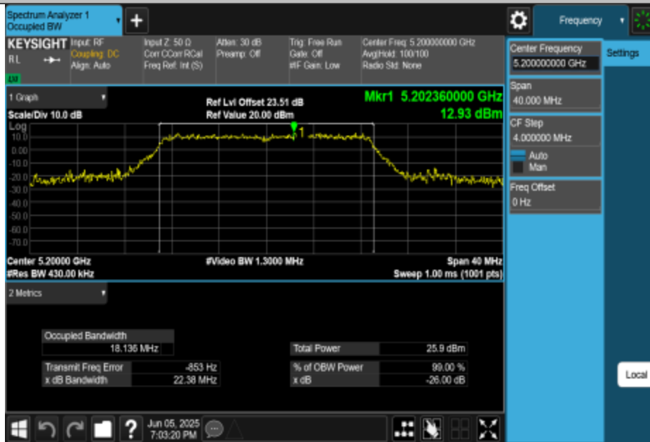
11AC20MIMO-Ant1-5200
