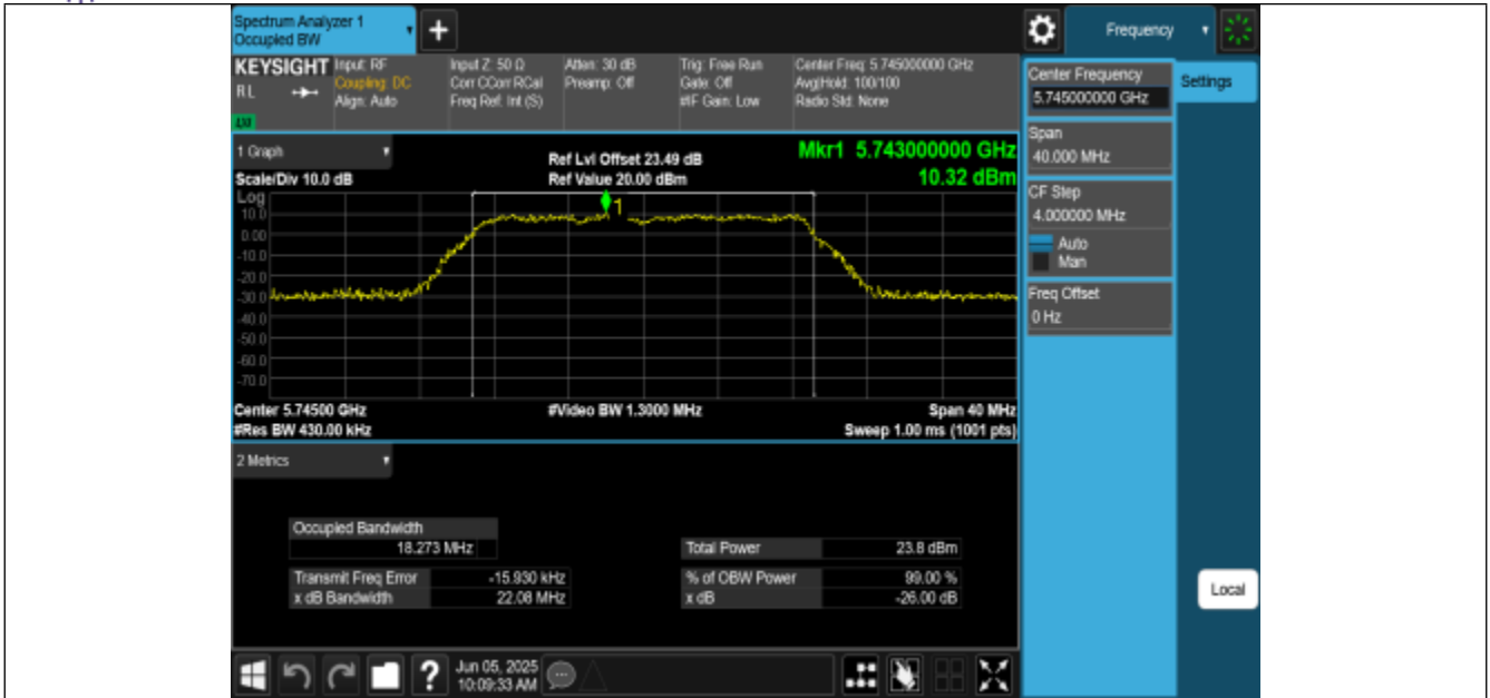
11N20MIMO-Ant0-5745
