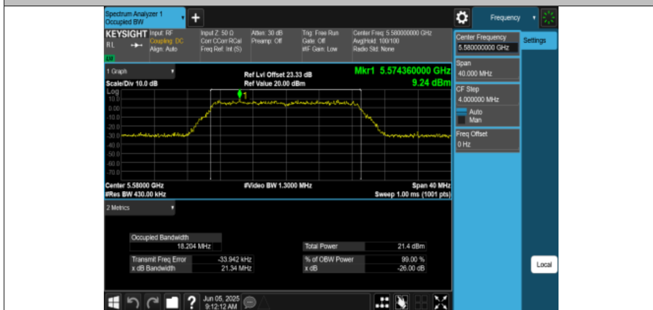
11N20MIMO-Ant1-5580
