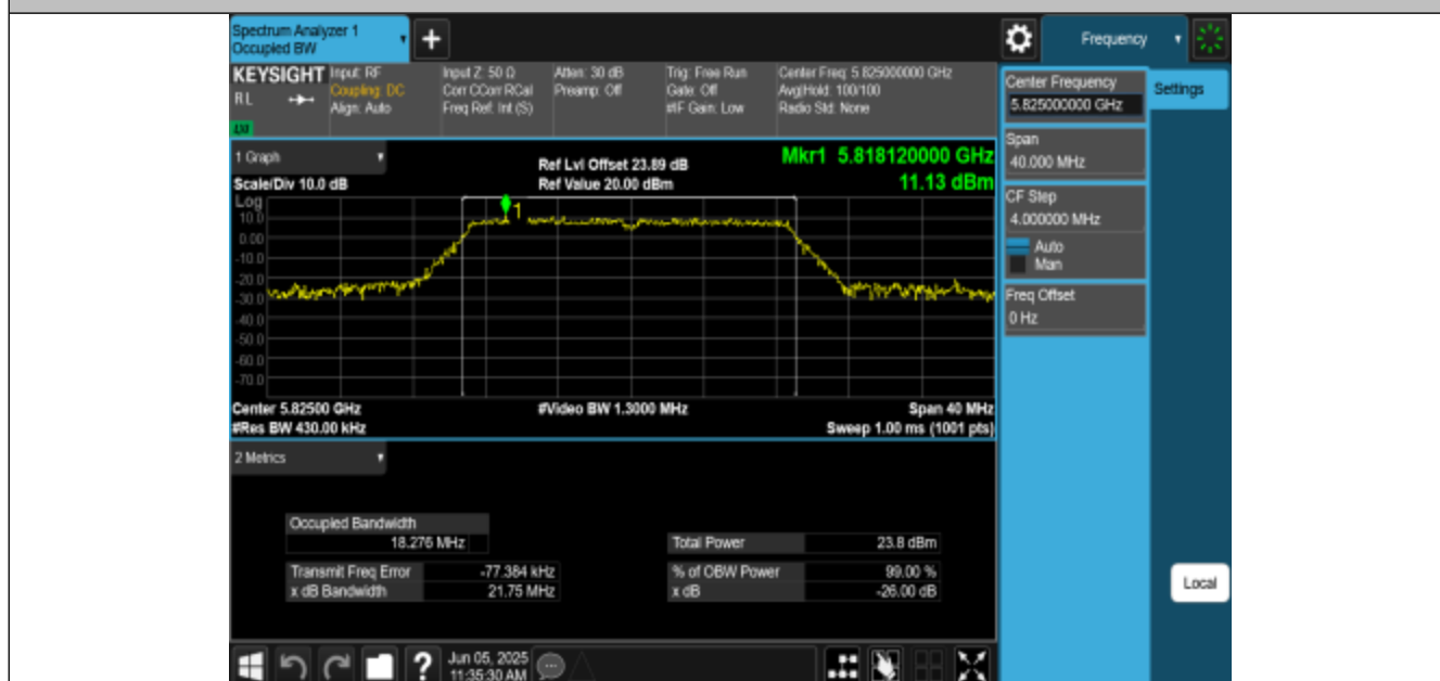
11N20MIMO-Ant3-5825
