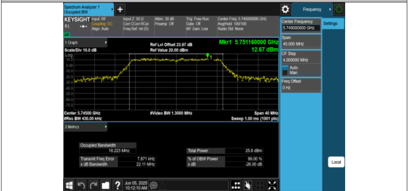
11N20MIMO-Ant1-5745
