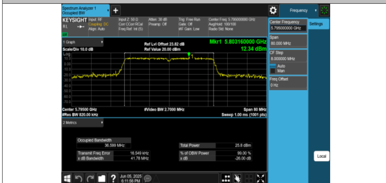
11N40MIMO-Ant1-5795
