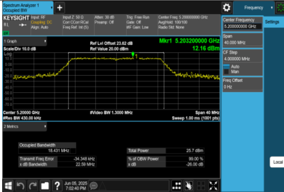
11AC20MIMO-Ant0-5200
