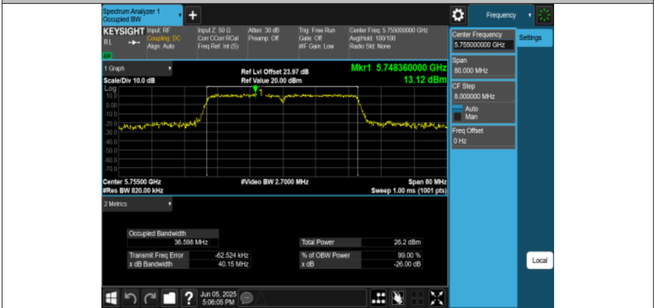
11N40MIMO-Ant1-5755
