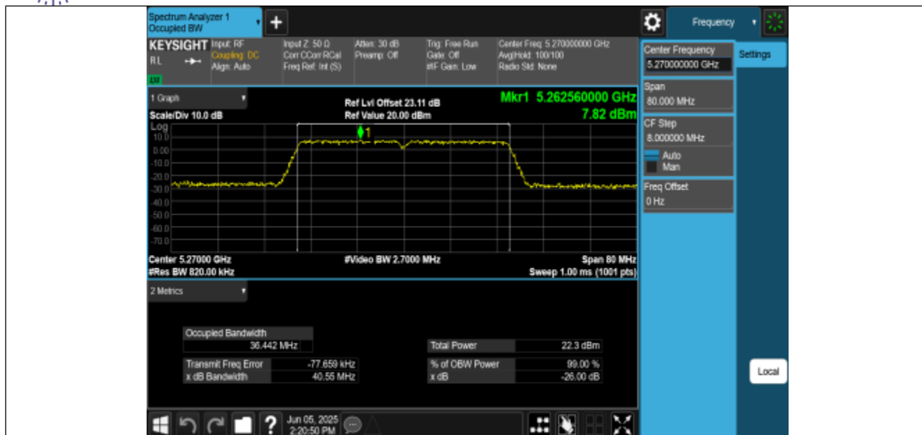
11N40MIMO-Ant0-5270
