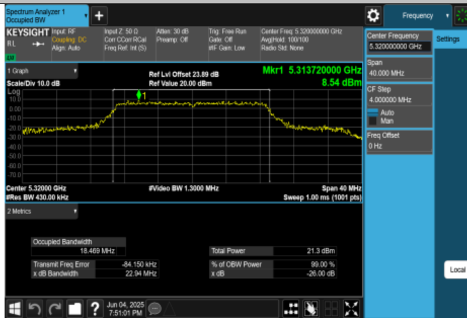
11N20MIMO-Ant3-5320
