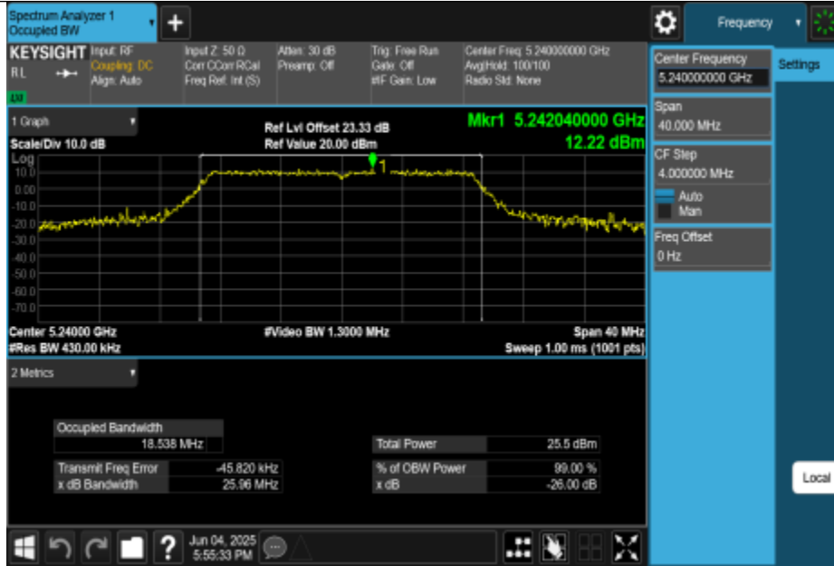
11N20MIMO-Ant0-5240
