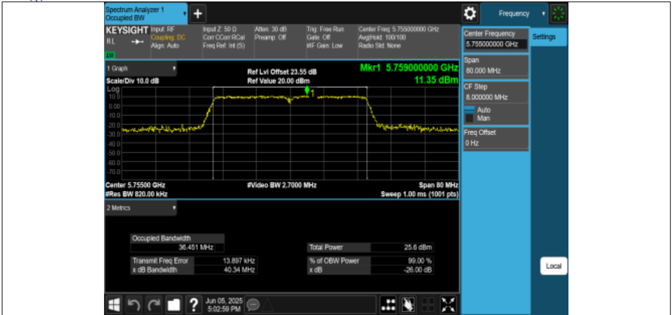
11N40MIMO-Ant0-5755
