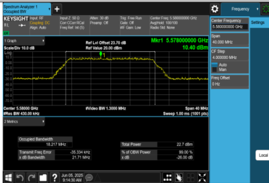
11N20MIMO-Ant3-5580
