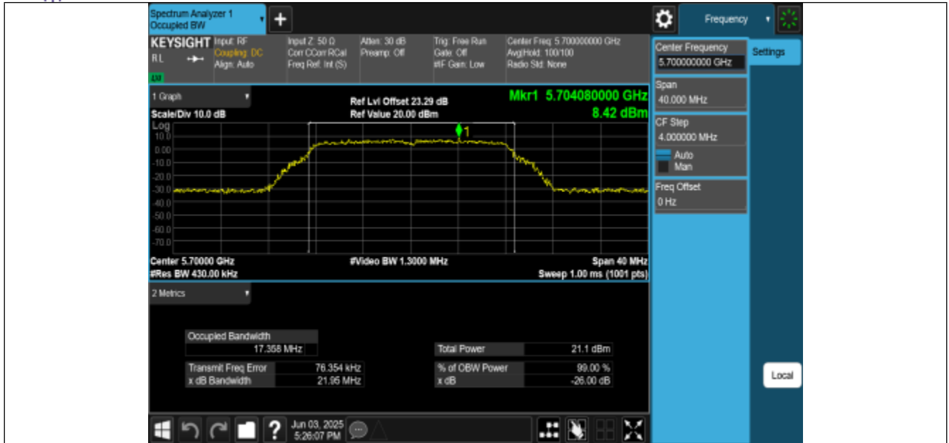
11A-CDD-Ant0-5700
