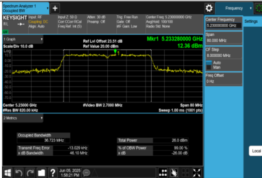
11N40MIMO-Ant1-5230
