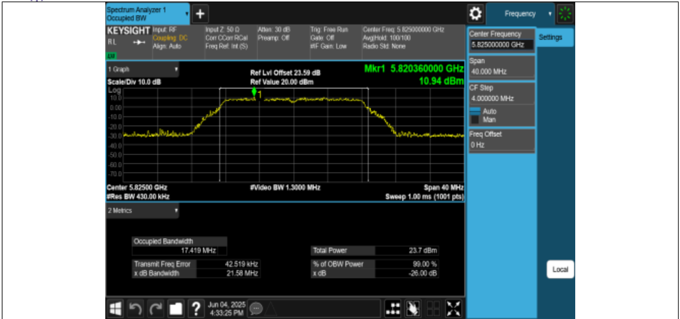
11A-CDD-Ant0-5825
