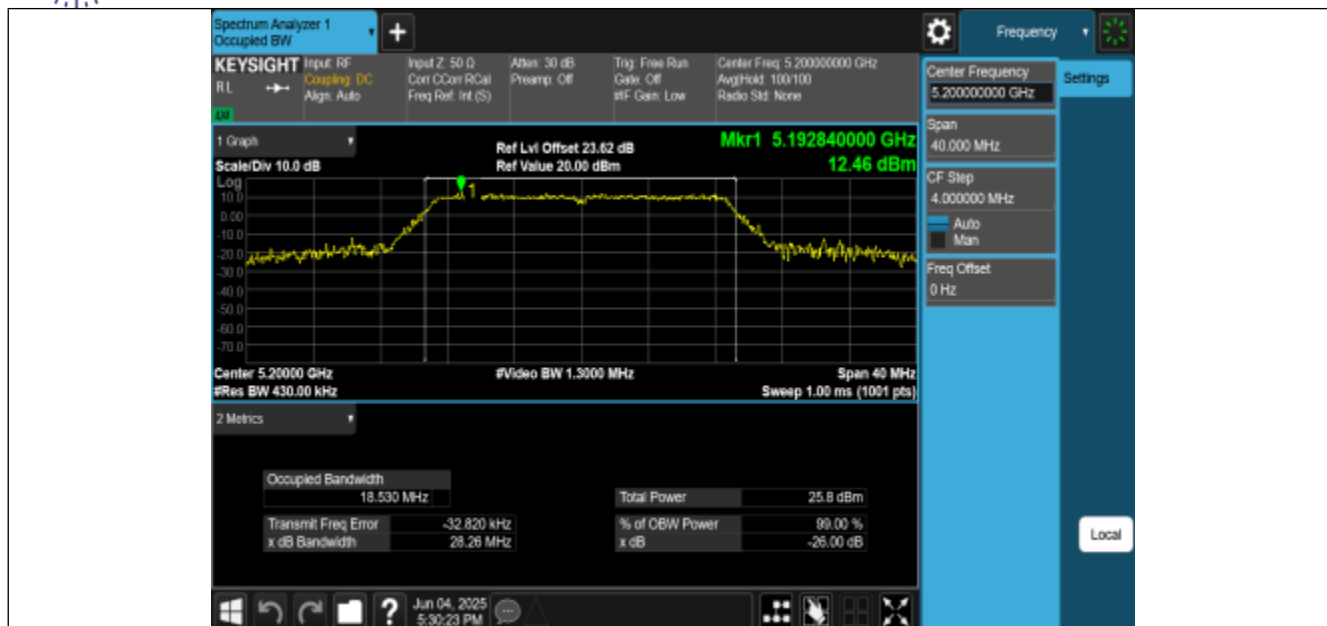
11N20MIMO-Ant0-5200
