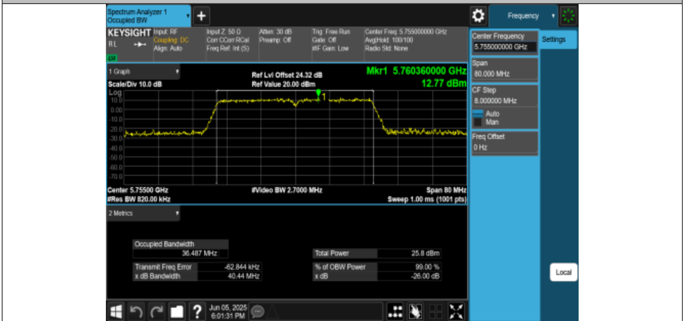
11N40MIMO-Ant3-5755
