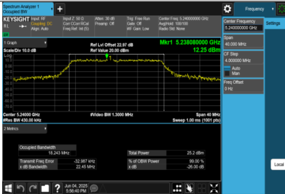
11N20MIMO-Ant1-5240
