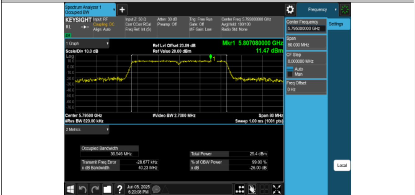
11N40MIMO-Ant3-5795
