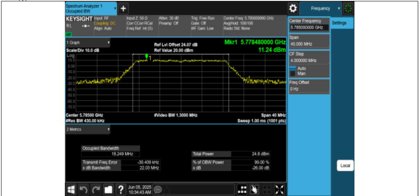
11N20MIMO-Ant0-5785
