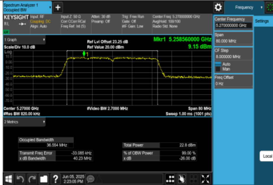
11N40MIMO-Ant2-5270
