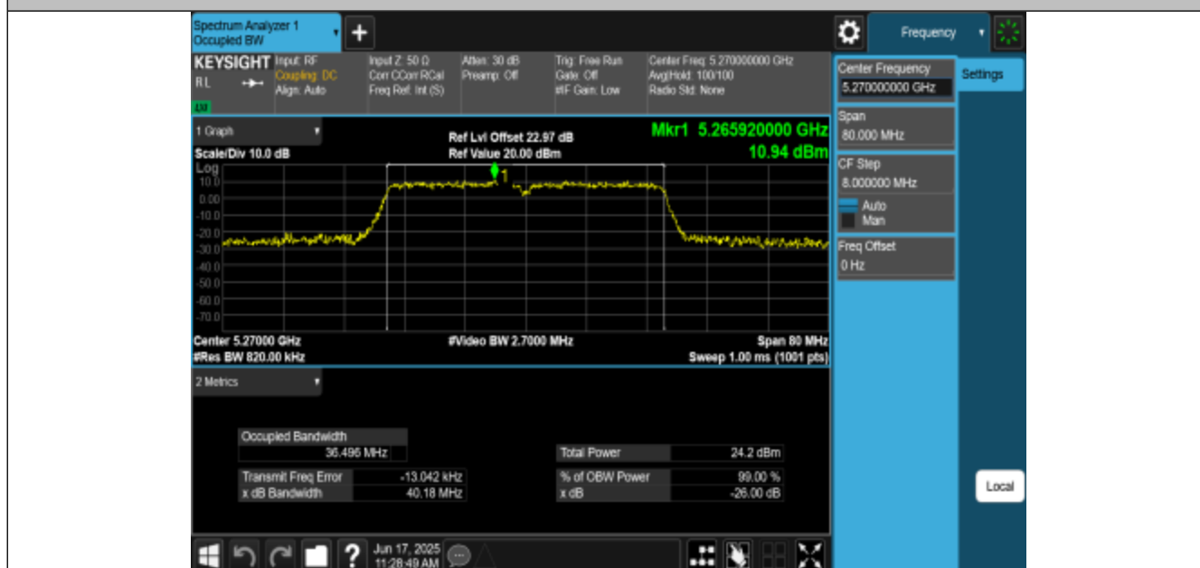
11N40MIMO-Ant1-5270
