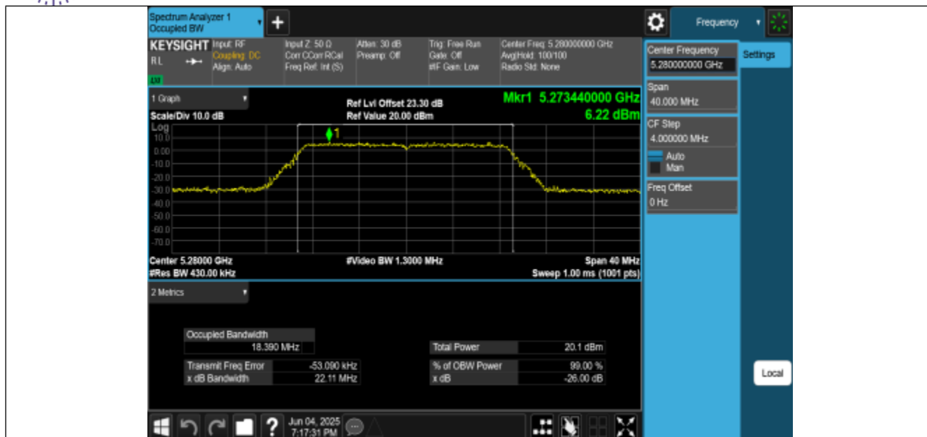
11N20MIMO-Ant0-5280
