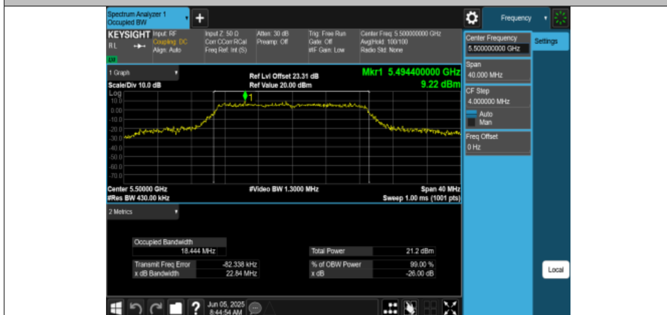
11N20MIMO-Ant1-5500
