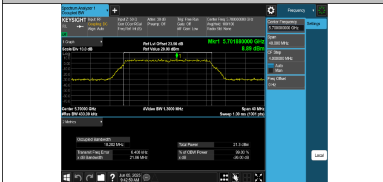
11N20MIMO-Ant3-5700
