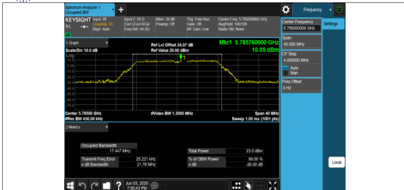
11A-CDD-Ant0-5785
