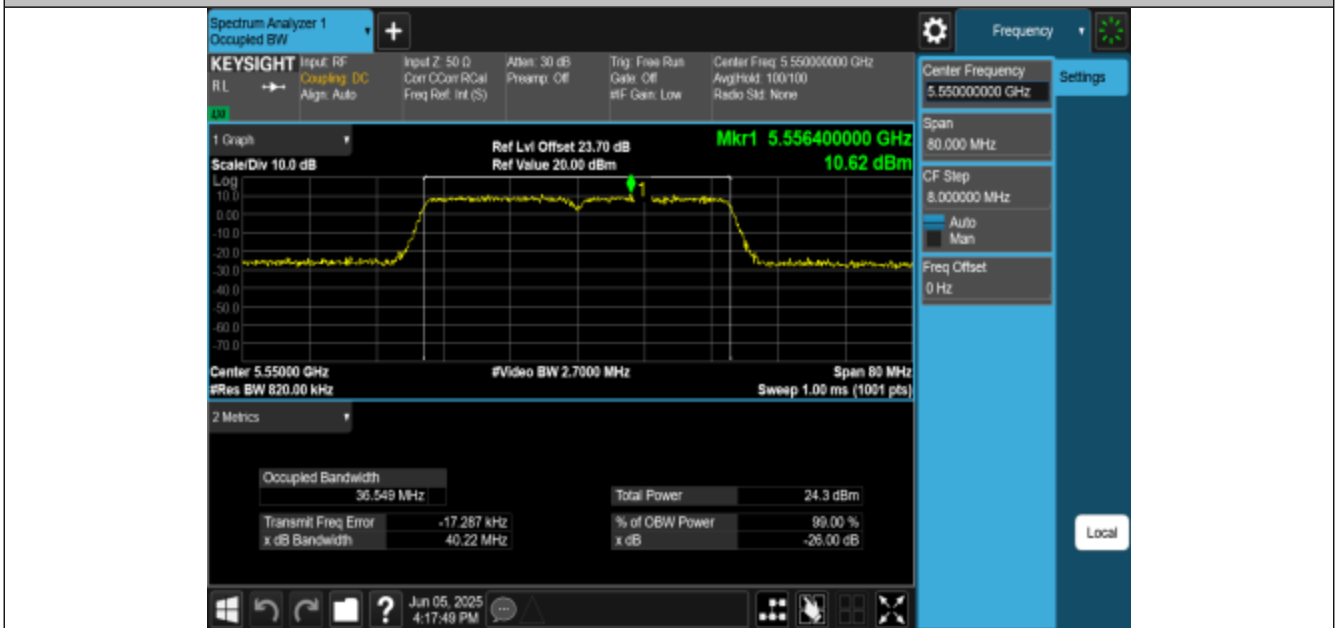
11N40MIMO-Ant3-5550
