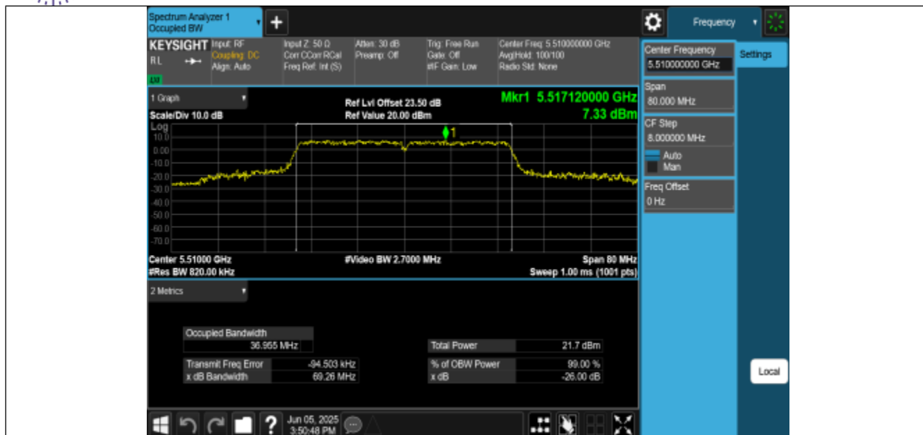
11N40MIMO-Ant0-5510
