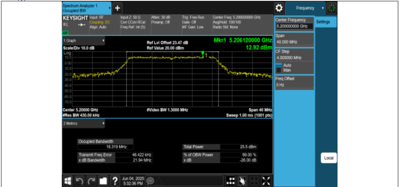
11N20MIMO-Ant2-5200
