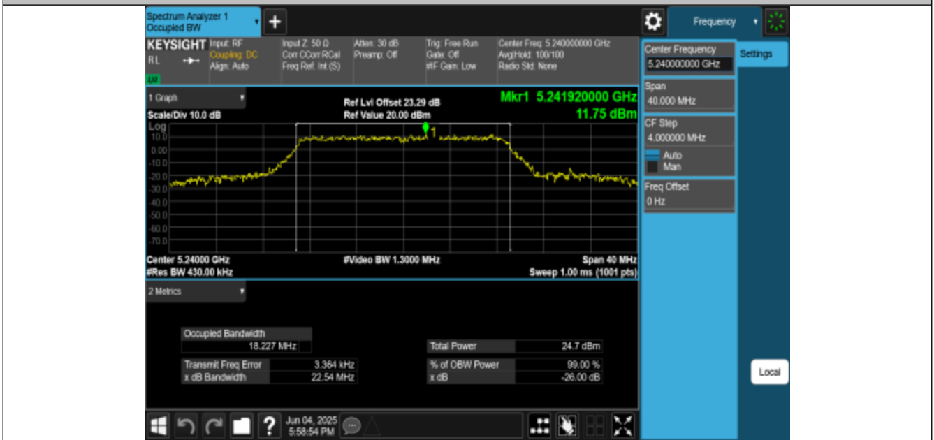
11N20MIMO-Ant3-5240
