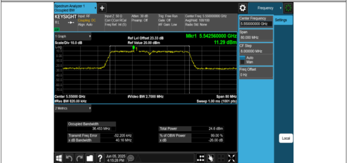
11N40MIMO-Ant1-5550
