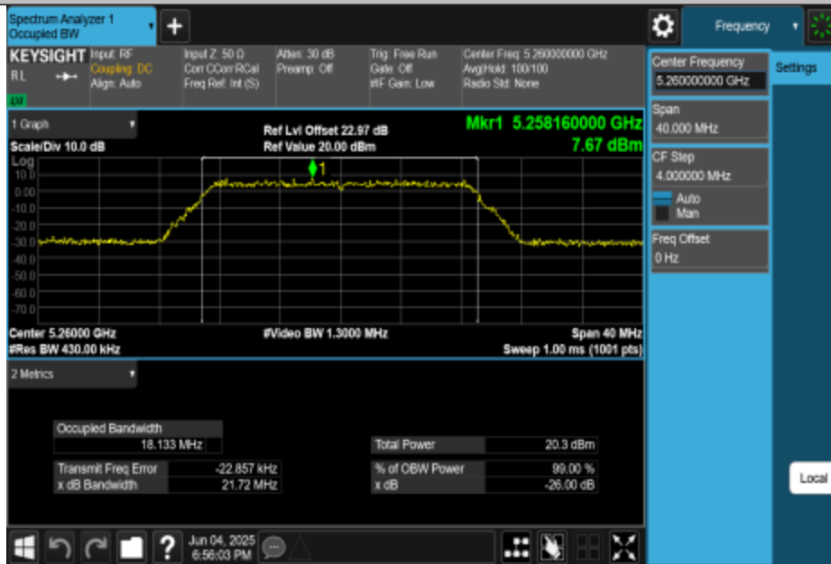
11N20MIMO-Ant1-5260
