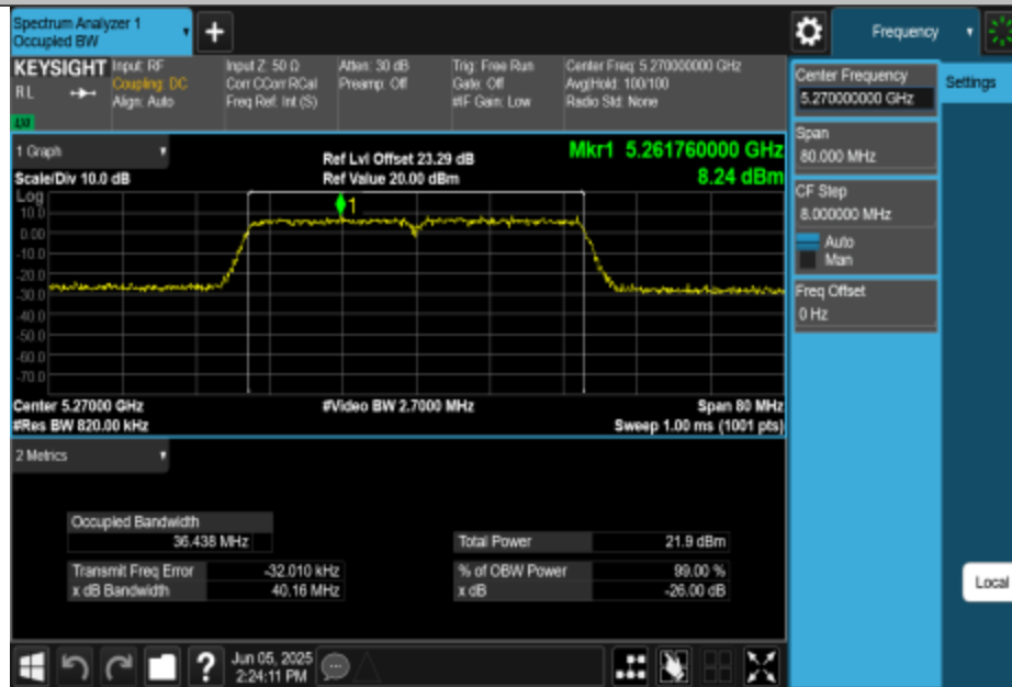
11N40MIMO-Ant3-5270
