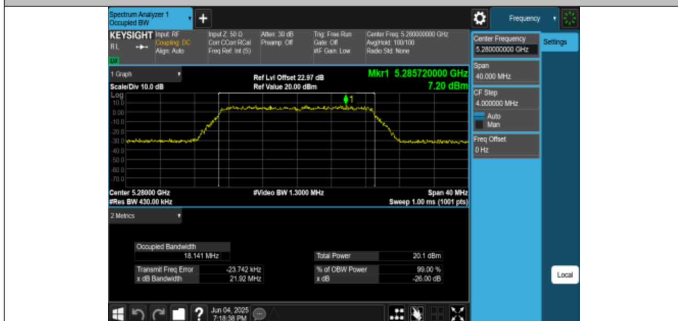
11N20MIMO-Ant1-5280
