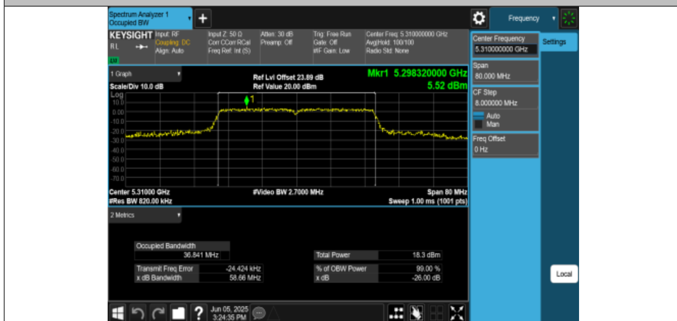
11N40MIMO-Ant3-5310
