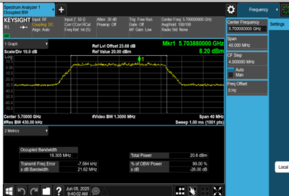
11N20MIMO-Ant1-5700
