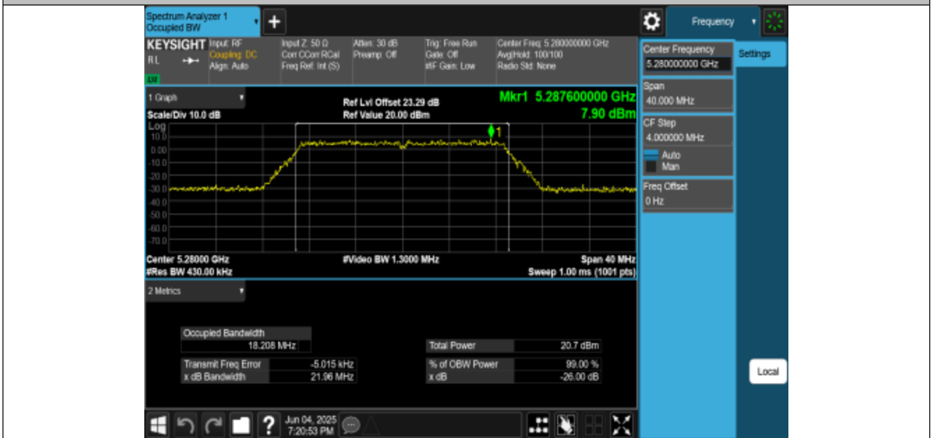
11N20MIMO-Ant3-5280
