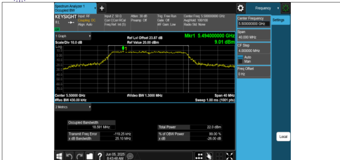
11N20MIMO-Ant0-5500
