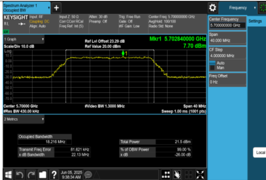
11N20MIMO-Ant0-5700
