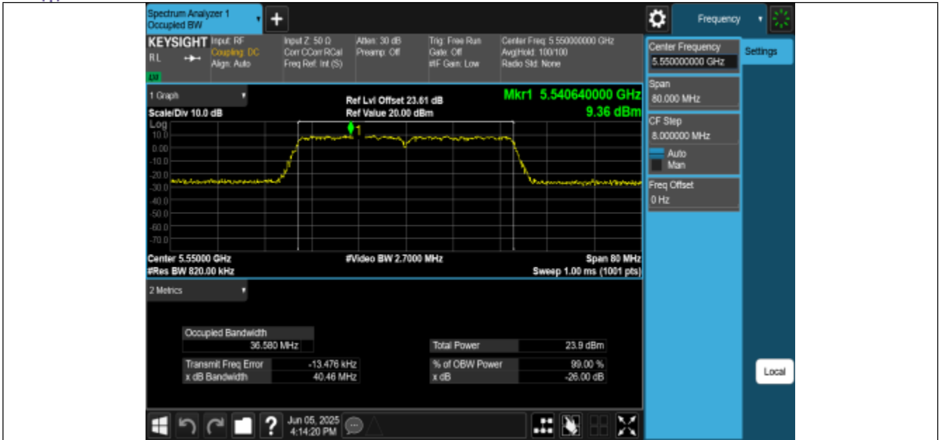
11N40MIMO-Ant0-5550
