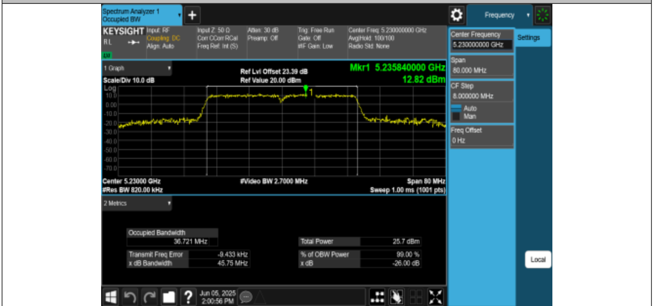
11N40MIMO-Ant3-5230
