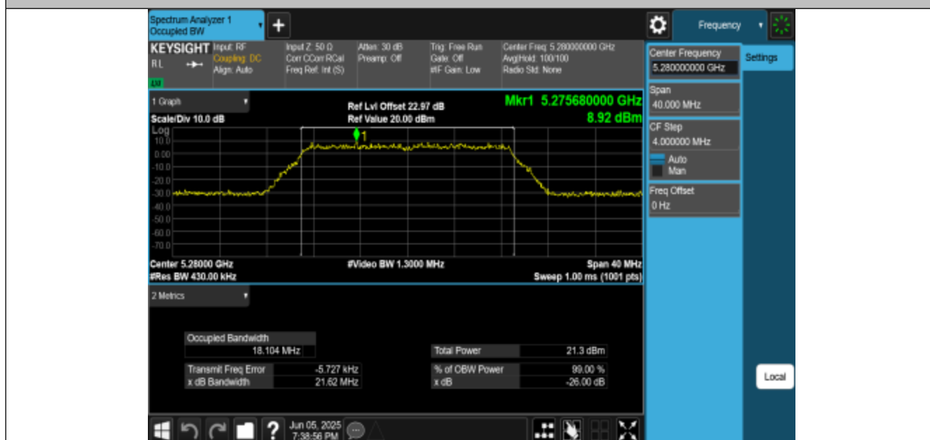
11AC20MIMO-Ant1-5280
