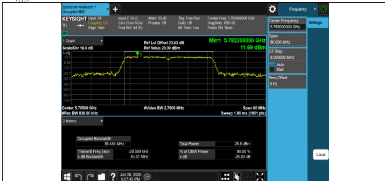
11N40MIMO-Ant0-5795
