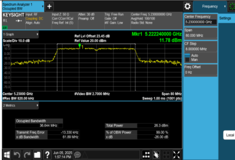
11N40MIMO-Ant0-5230
