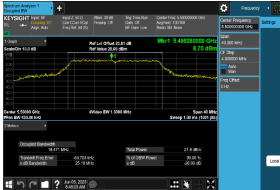
11N20MIMO-Ant2-5500
