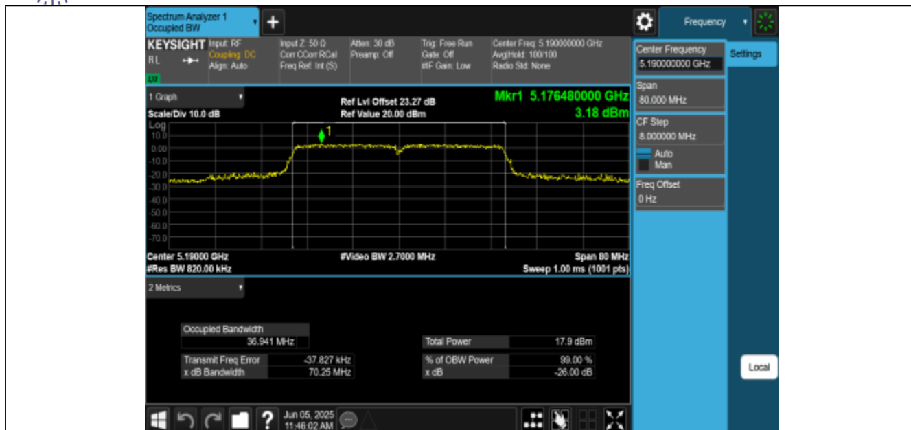
11N40MIMO-Ant0-5190
