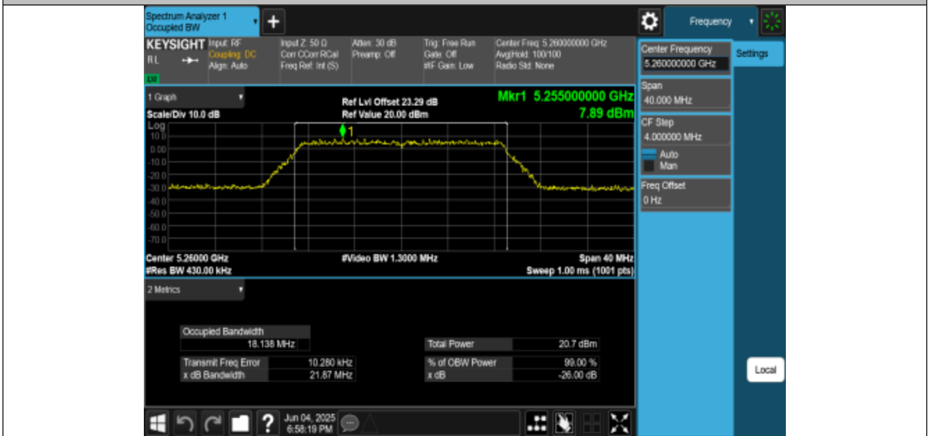
11N20MIMO-Ant3-5260
