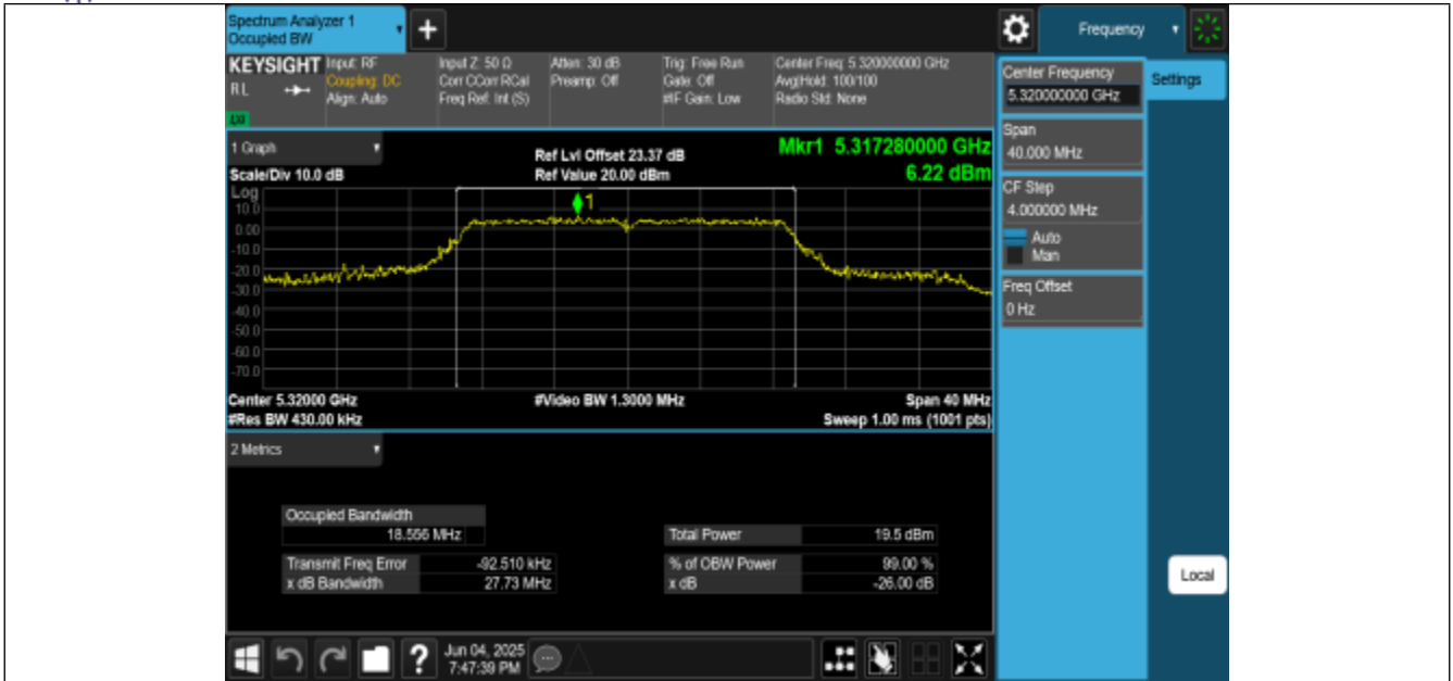
11N20MIMO-Ant0-5320
