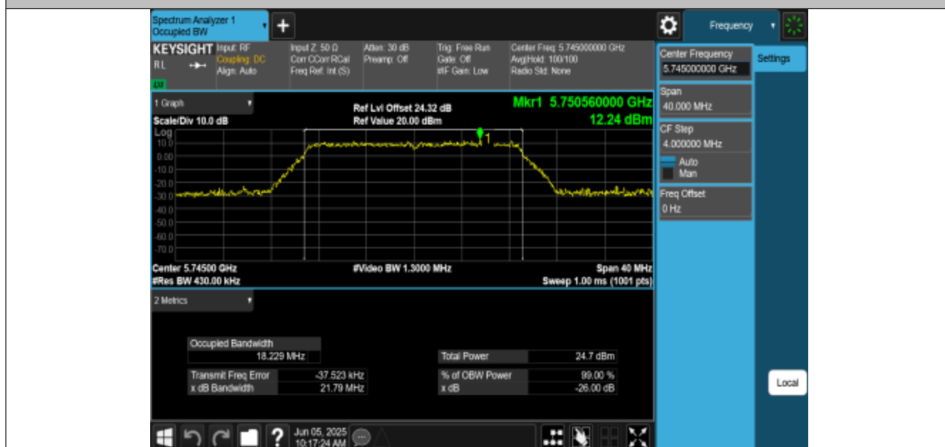
11N20MIMO-Ant3-5745
