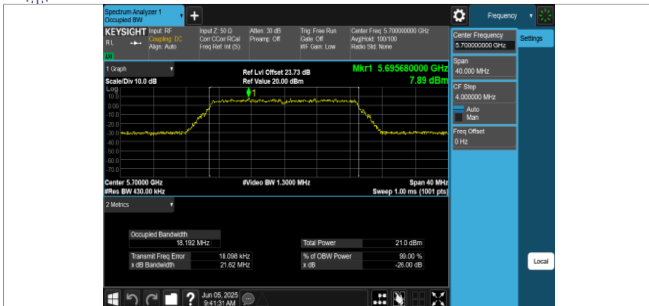
11N20MIMO-Ant2-5700
