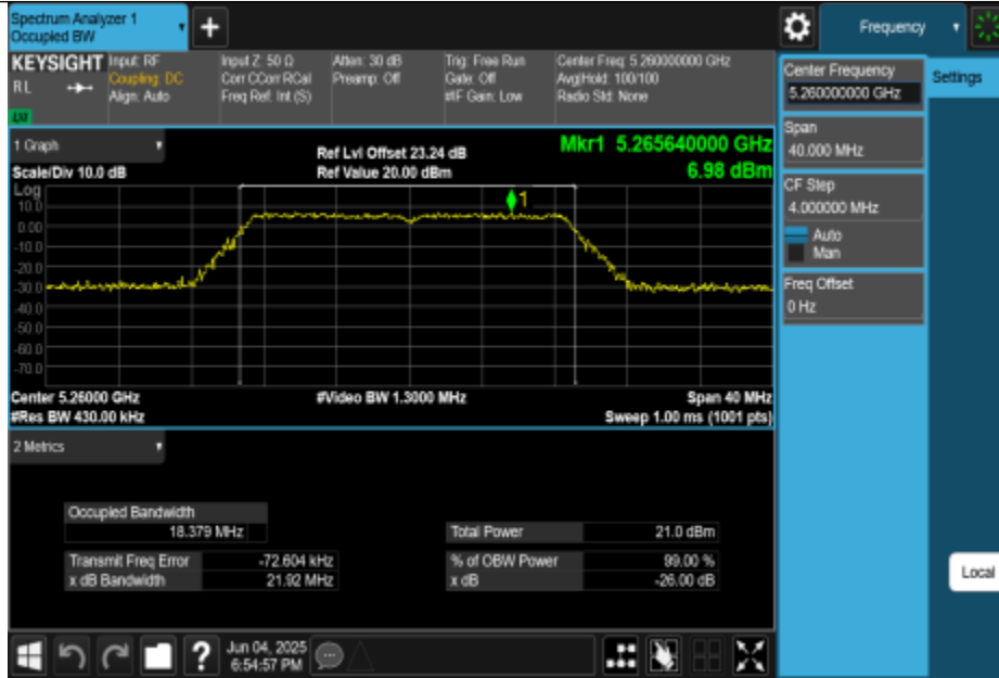
11N20MIMO-Ant0-5260
