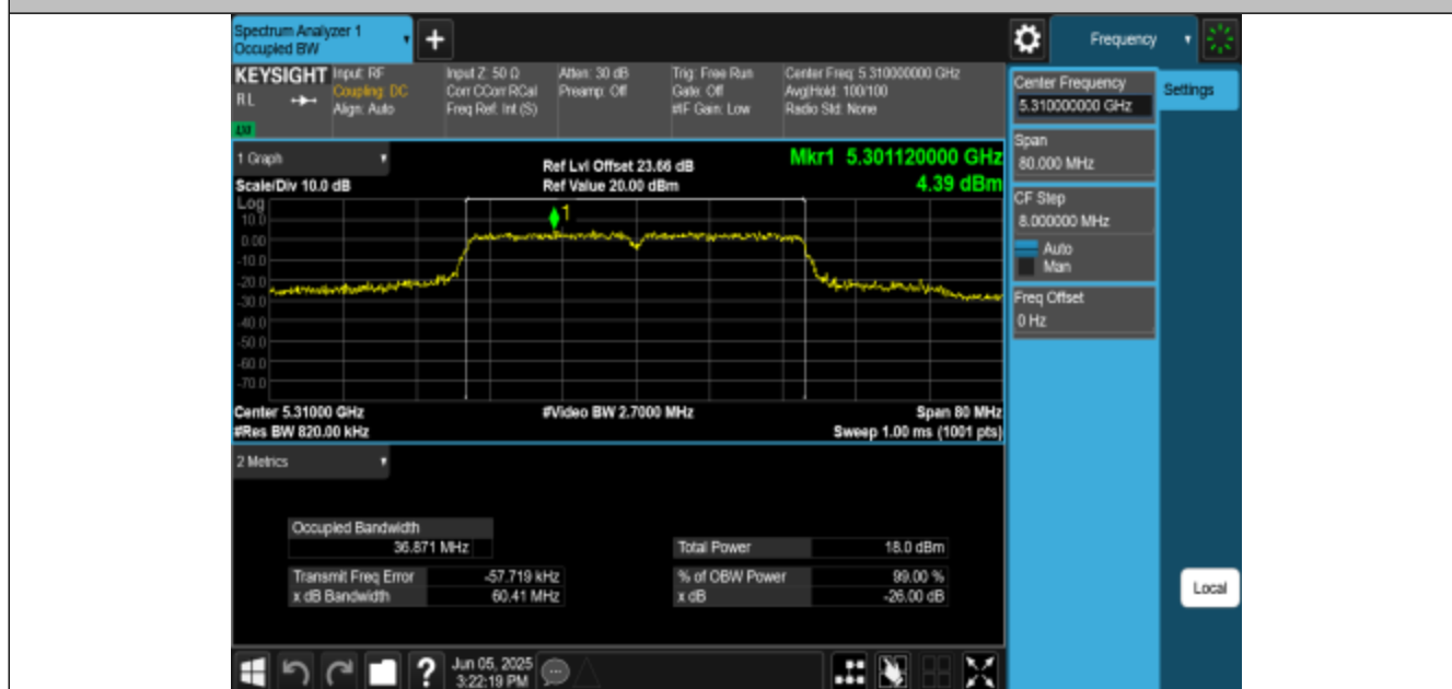
11N40MIMO-Ant1-5310
