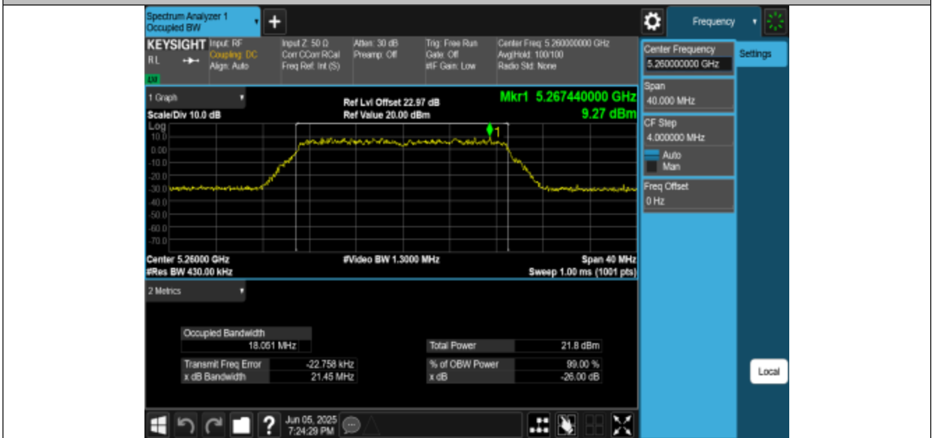
11AC20MIMO-Ant1-5260
