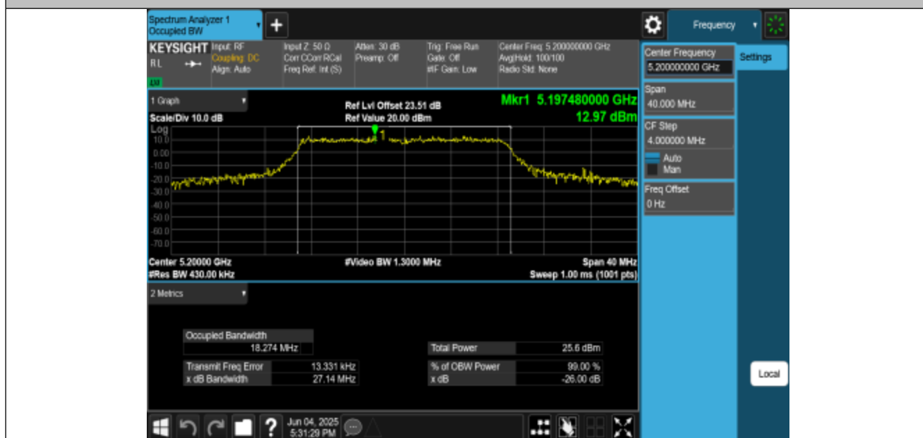
11N20MIMO-Ant1-5200
