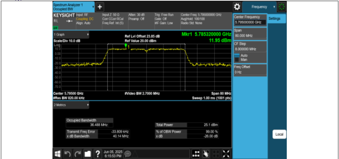
11N40MIMO-Ant2-5795
