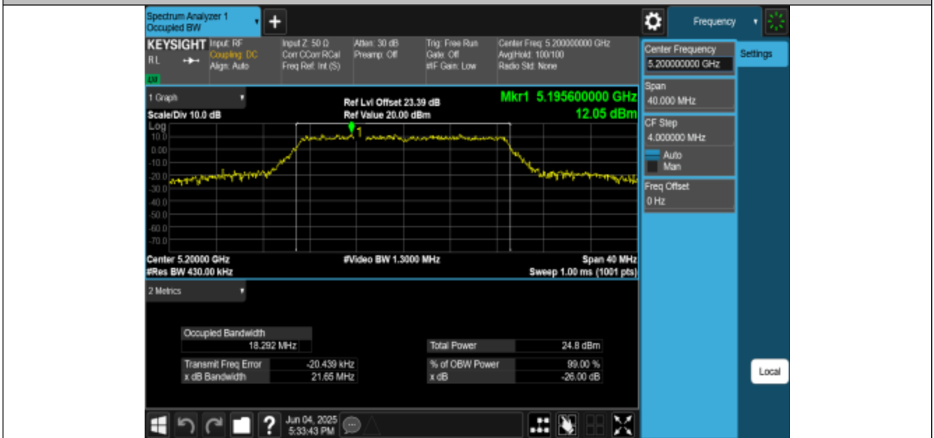
11N20MIMO-Ant3-5200
