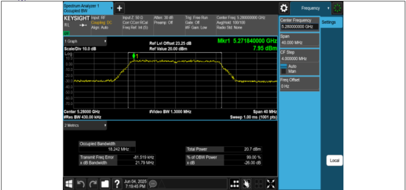
11N20MIMO-Ant2-5280
