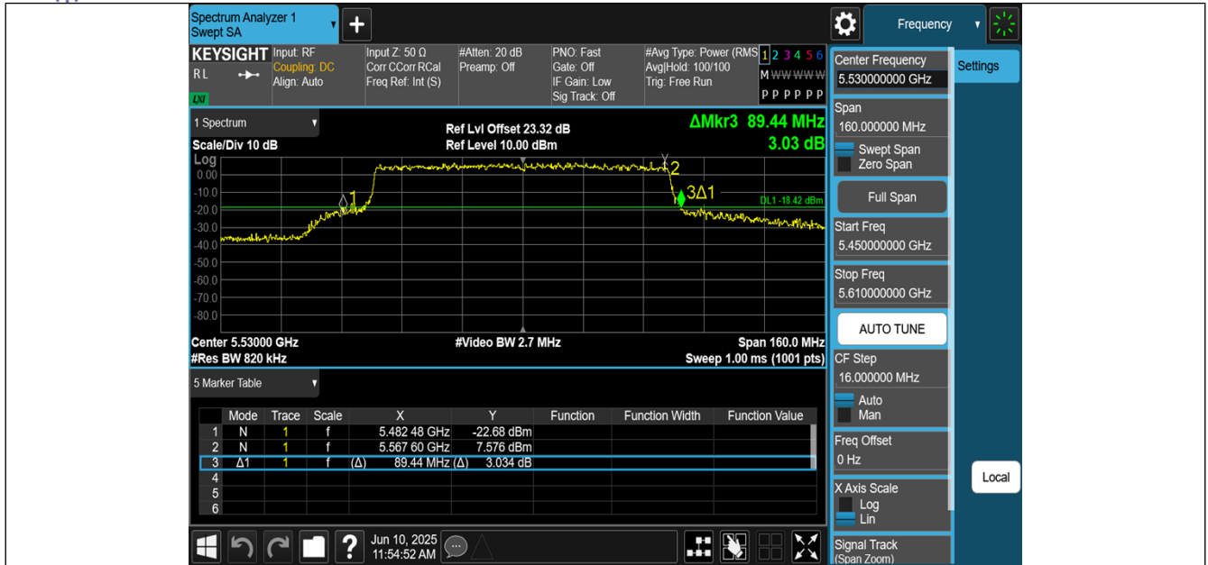
11BE80MIMO-Ant0-5530
