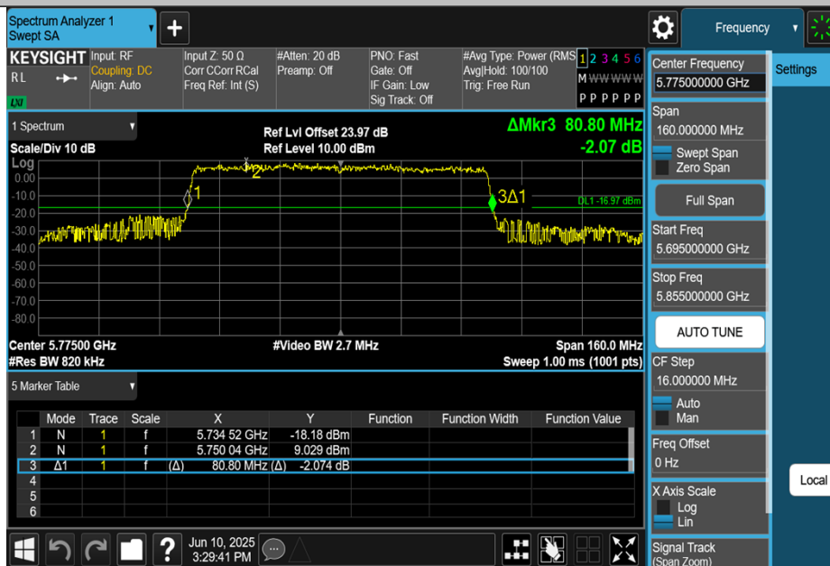
11BE80MIMO-Ant1-5775
