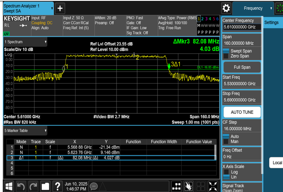
11BE80MIMO-Ant0-5610
