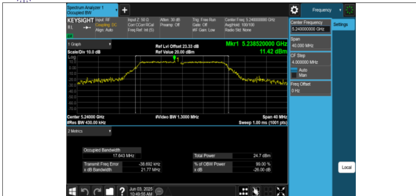
11A-CDD-Ant0-5240
