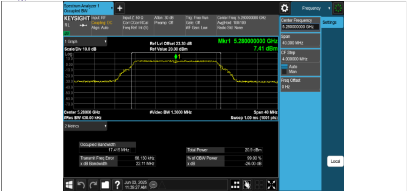
11A-CDD-Ant0-5280
