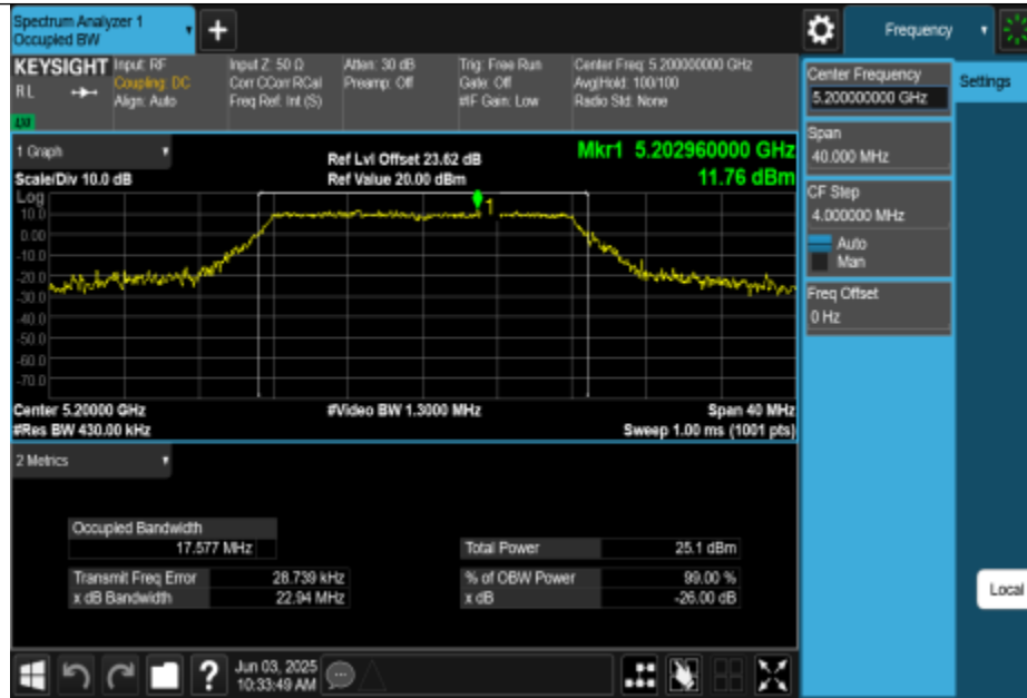
11A-CDD-Ant0-5200
