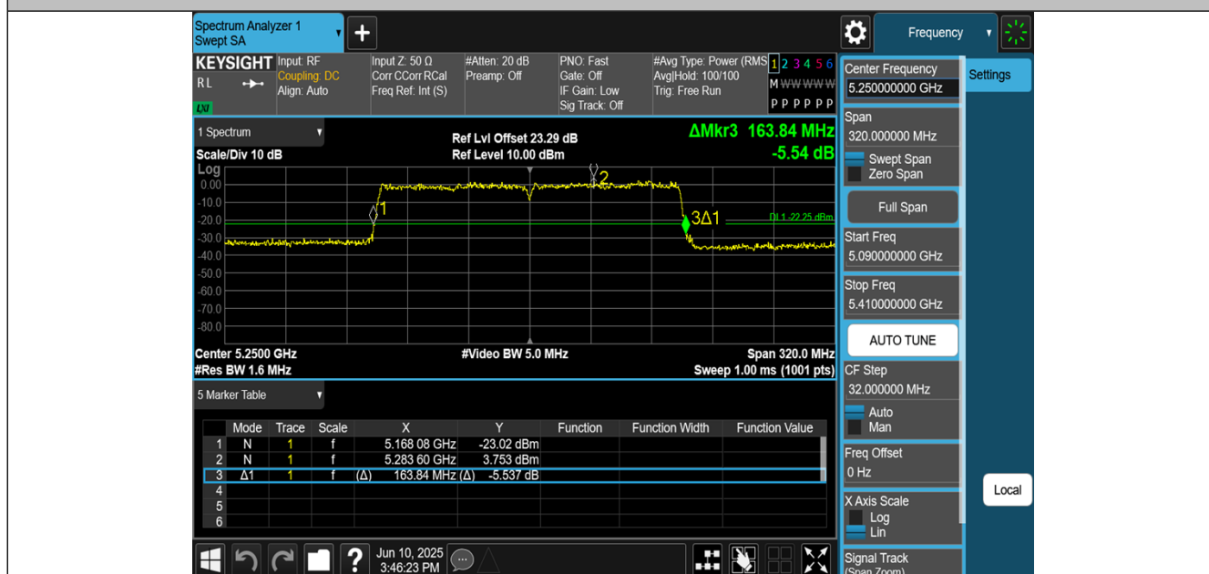
11BE160MIMO-Ant3-5250
