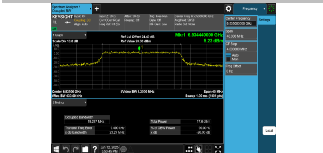
11BE20MIMO-Ant1-6535-PASS
