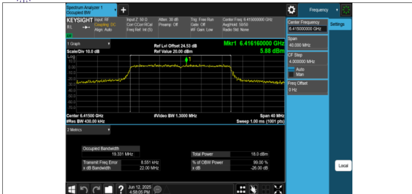
11BE20MIMO-Ant0-6415-PASS
