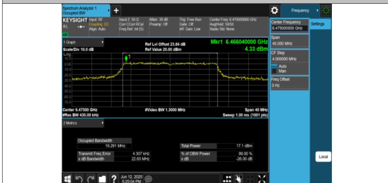
11BE20MIMO-Ant1-6475-PASS
