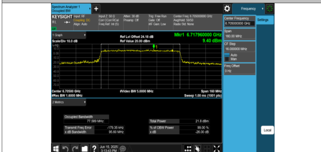
11BE80MIMO-Ant1-6705-PASS
