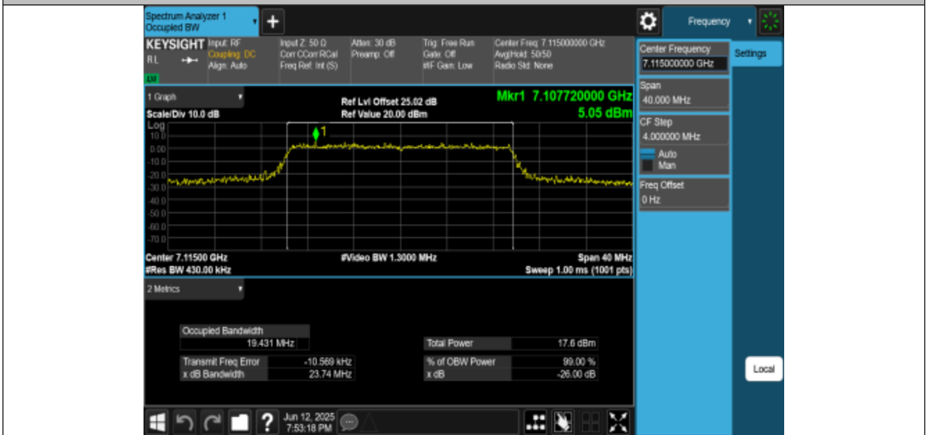
11BE20MIMO-Ant3-7115-PASS
