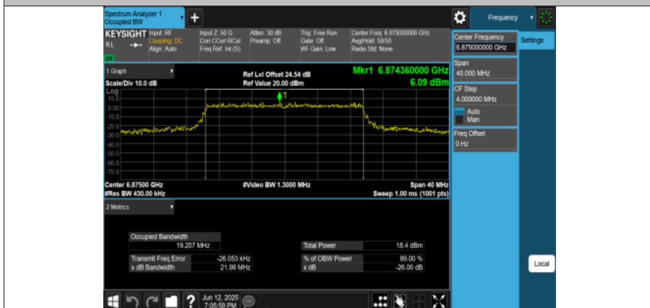
11BE20MIMO-Ant1-6875-PASS
