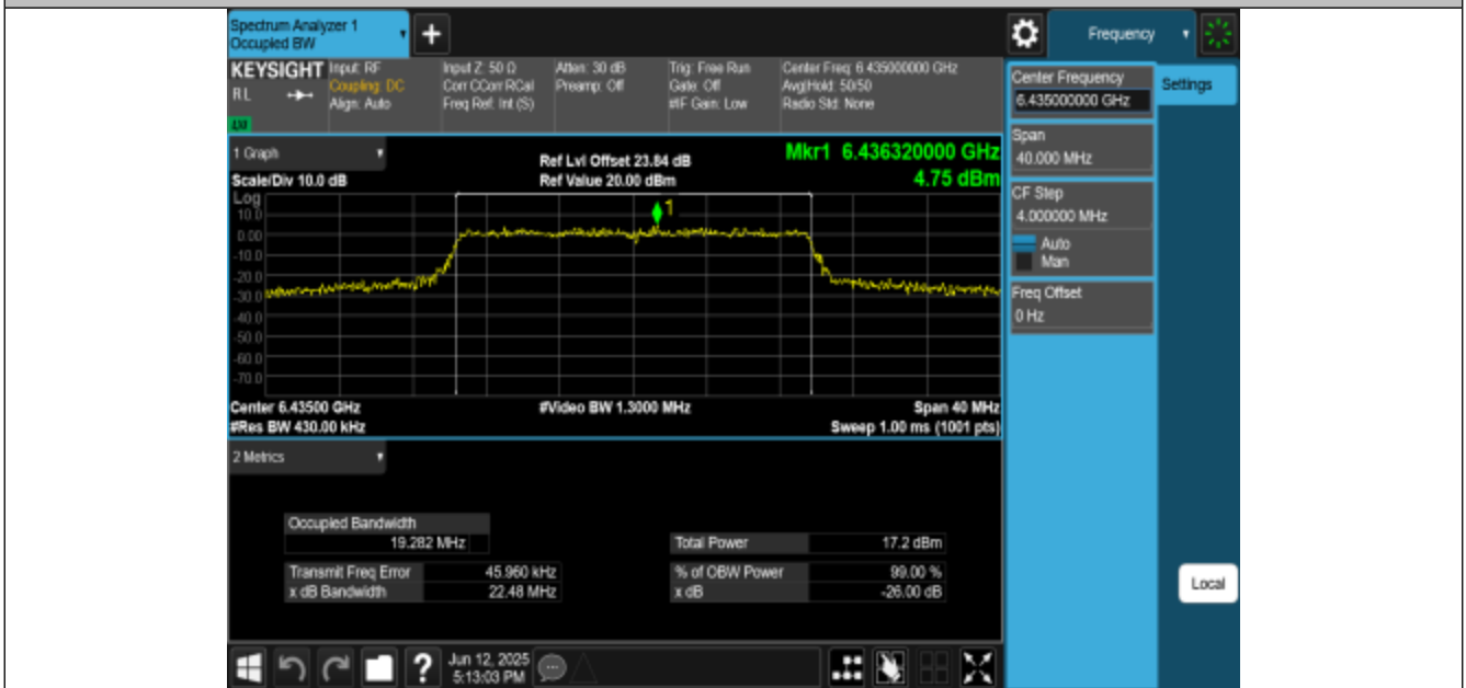
11BE20MIMO-Ant1-6435-PASS
