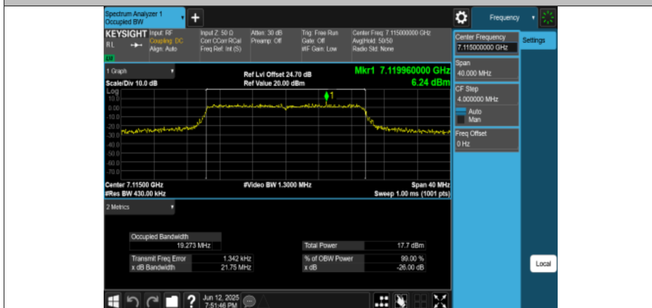
11BE20MIMO-Ant1-7115-PASS
