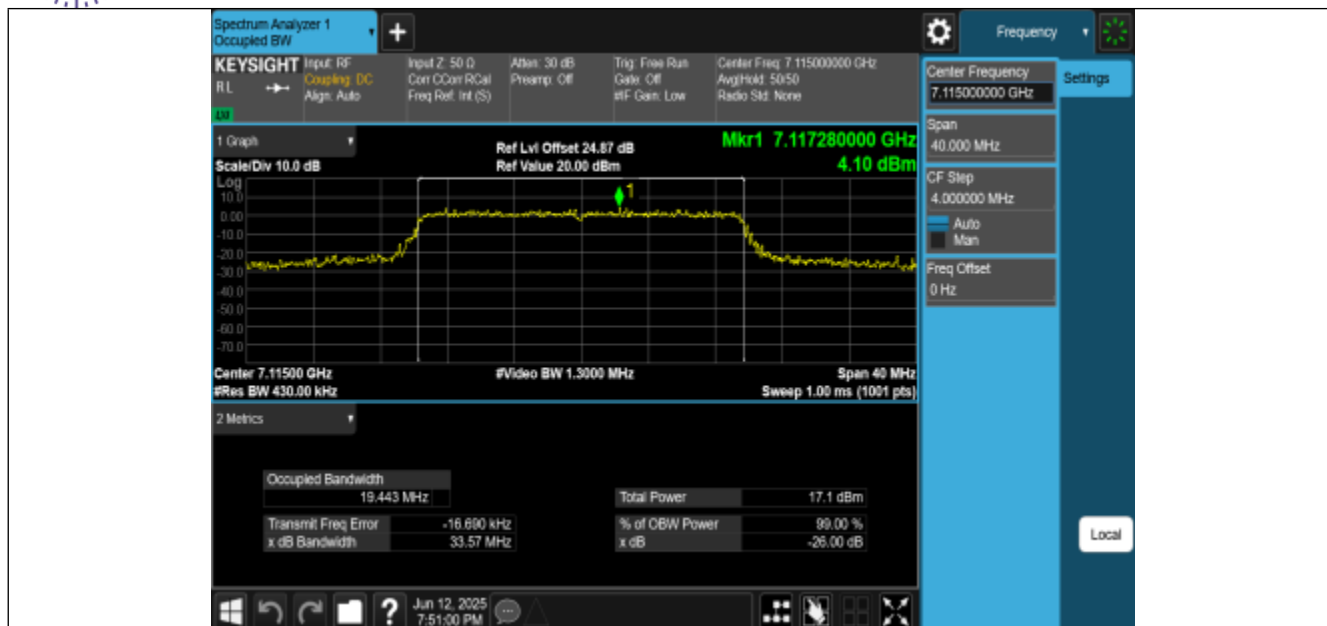
11BE20MIMO-Ant0-7115-PASS
