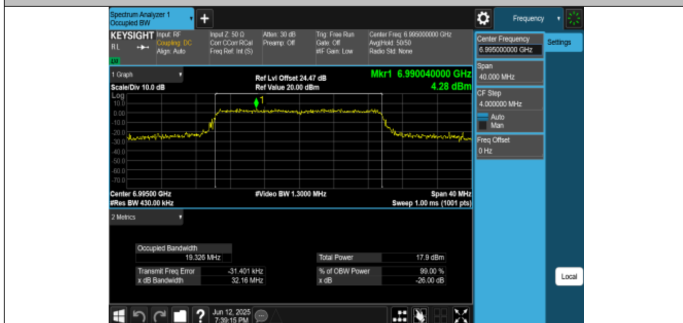
11BE20MIMO-Ant1-6995-PASS
