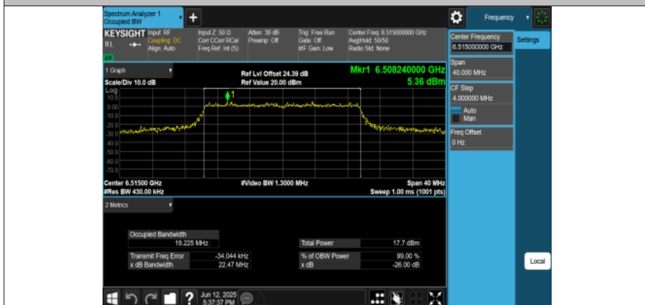
11BE20MIMO-Ant1-6515-PASS
