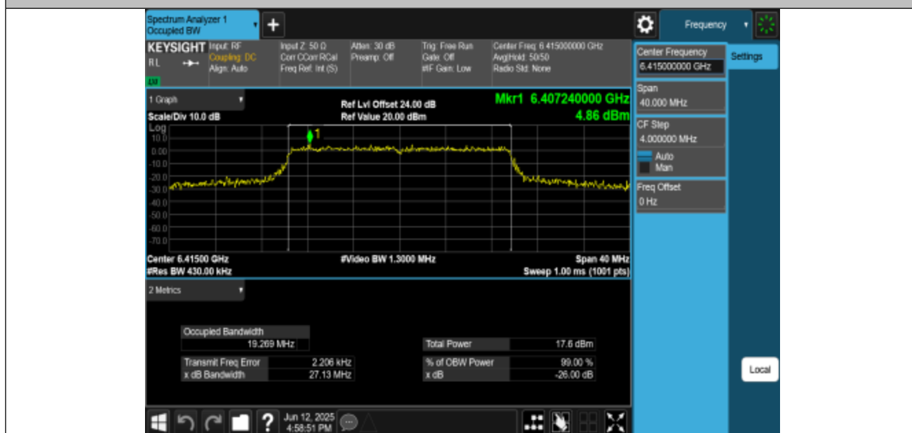
11BE20MIMO-Ant1-6415-PASS
