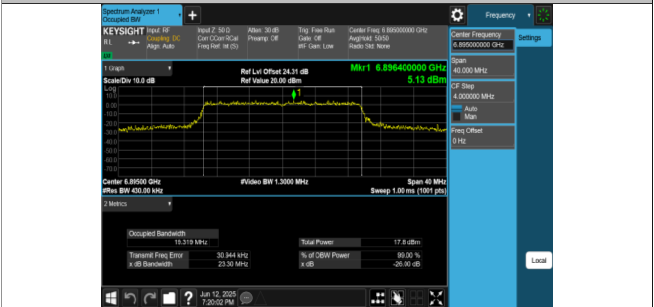
11BE20MIMO-Ant1-6895-PASS
