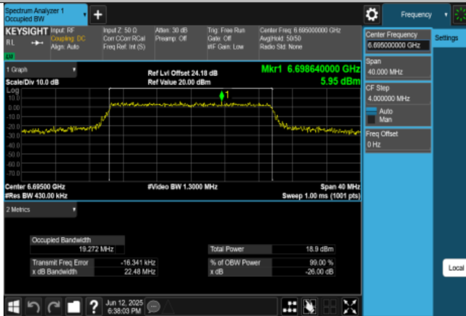
11BE20MIMO-Ant1-6695-PASS
