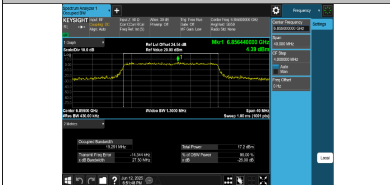
11BE20MIMO-Ant1-6855-PASS
