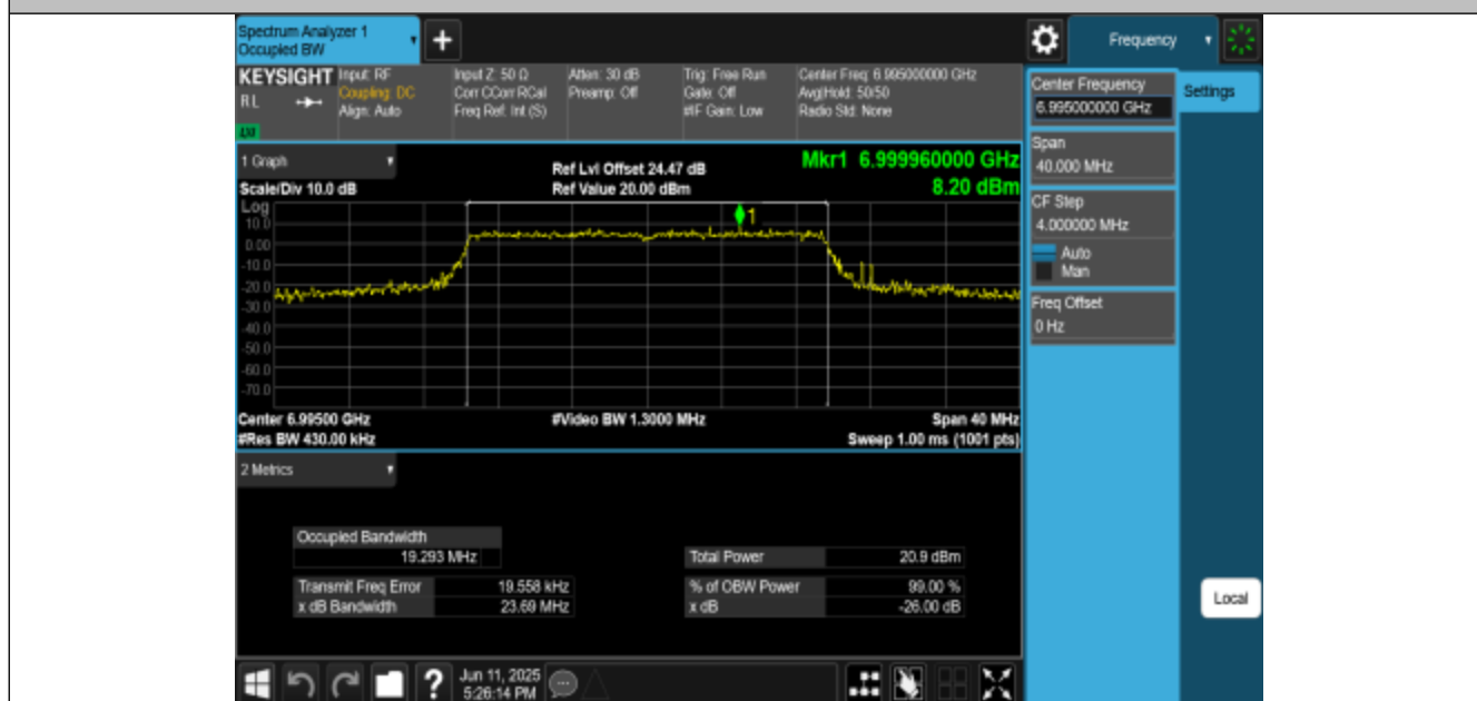
11AX20MIMO-Ant1-6995-PASS
