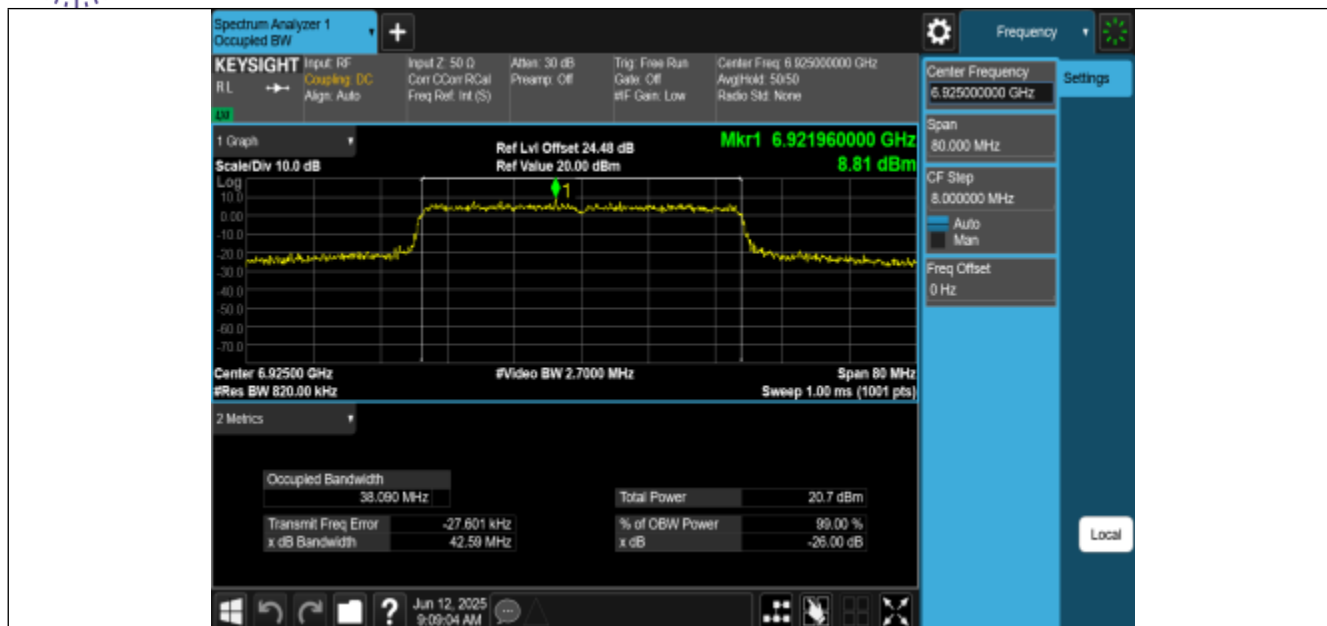
11AX40MIMO-Ant0-6925-PASS
