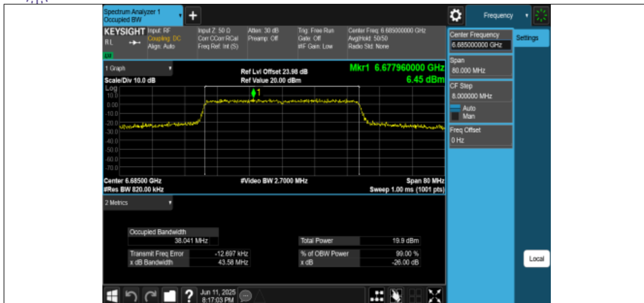
11AX40MIMO-Ant0-6685-PASS
