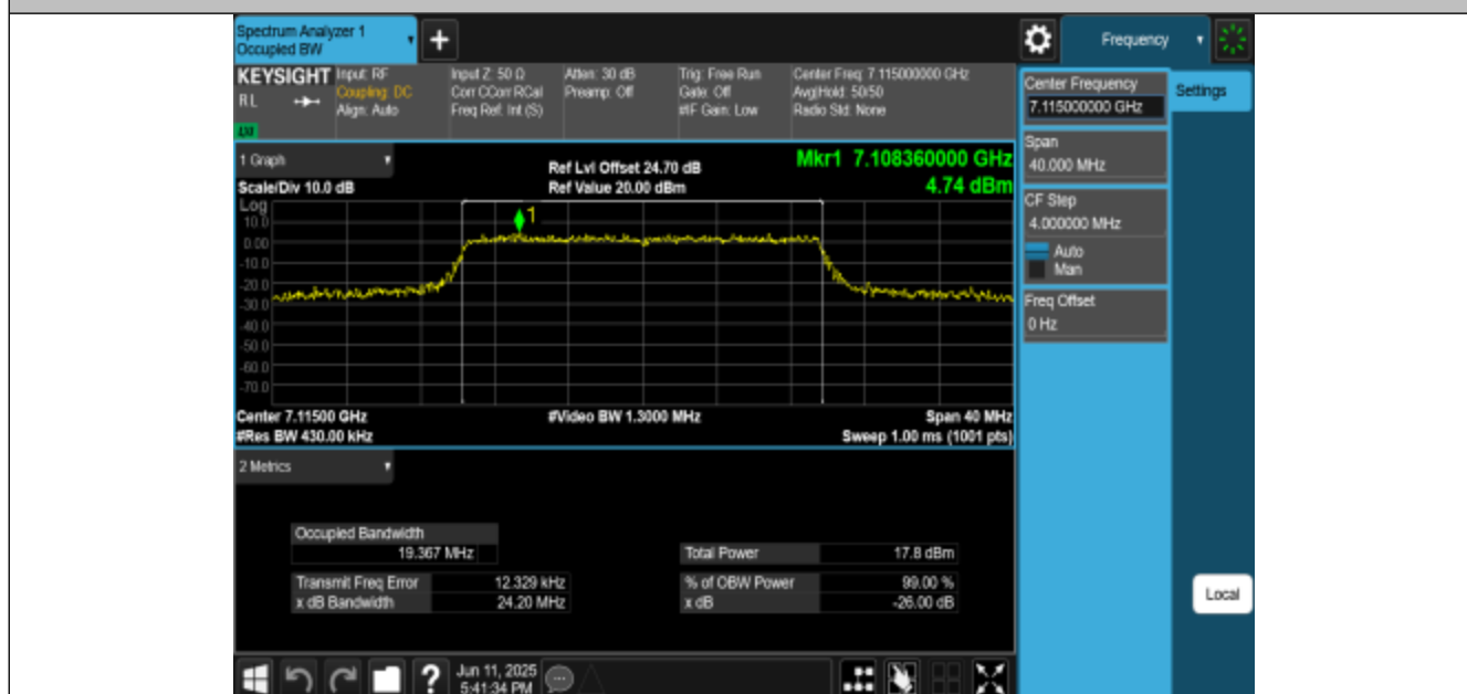
11AX20MIMO-Ant1-7115-PASS
