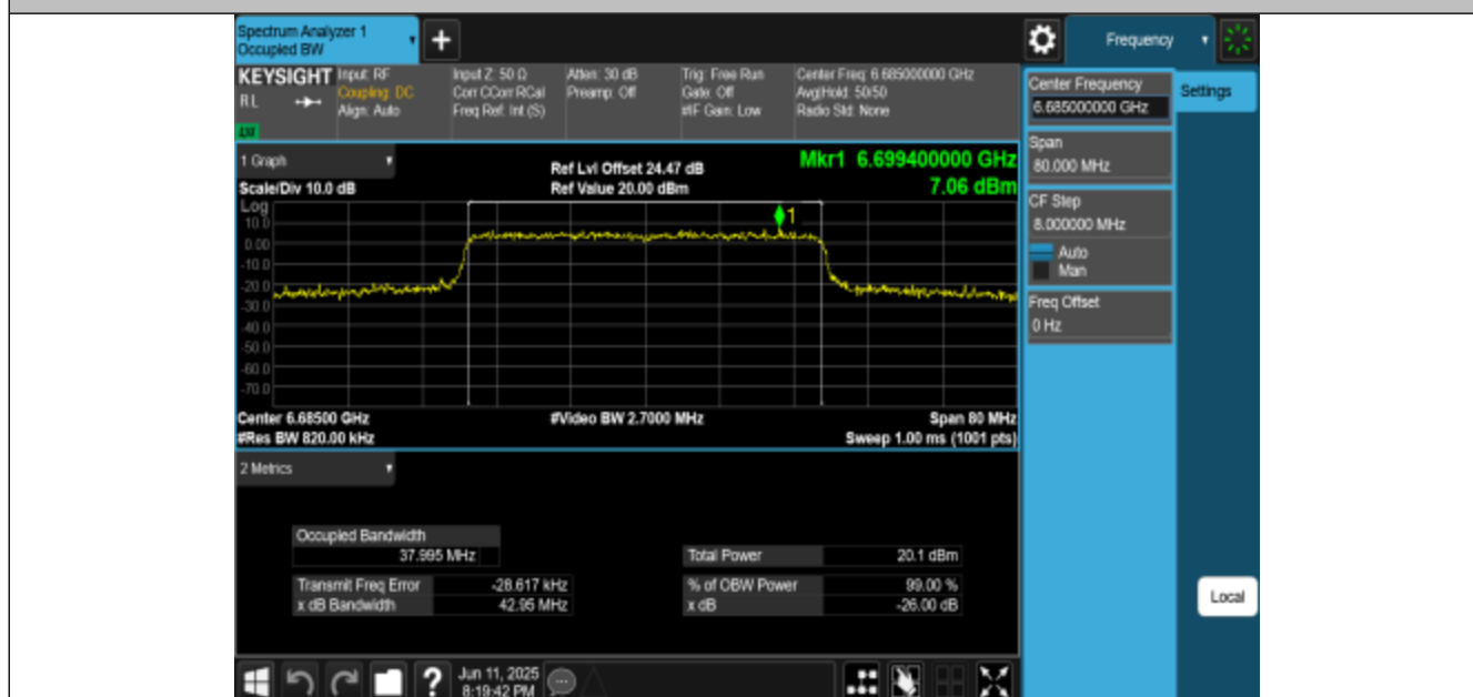
11AX40MIMO-Ant3-6685-PASS
