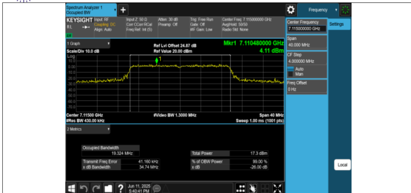
11AX20MIMO-Ant0-7115-PASS
