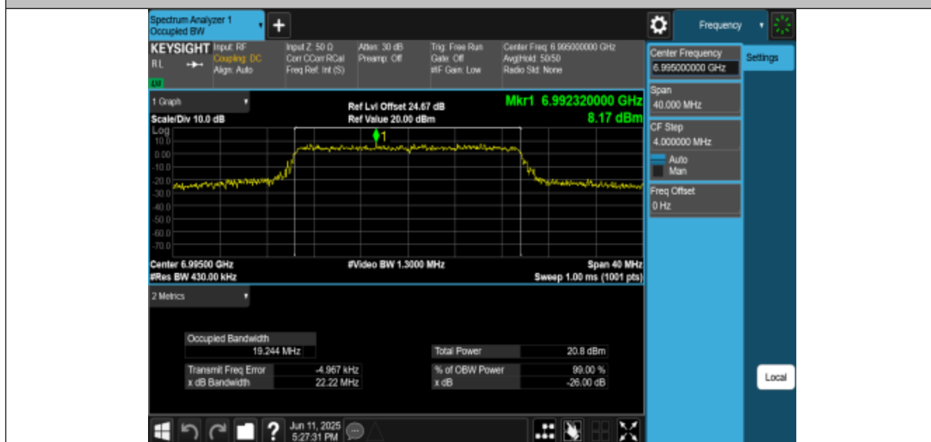
11AX20MIMO-Ant3-6995-PASS
