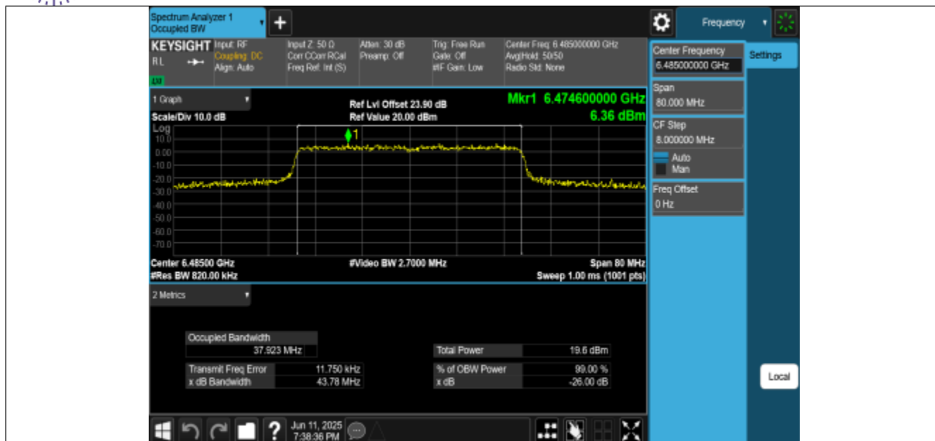
11AX40MIMO-Ant0-6485-PASS
