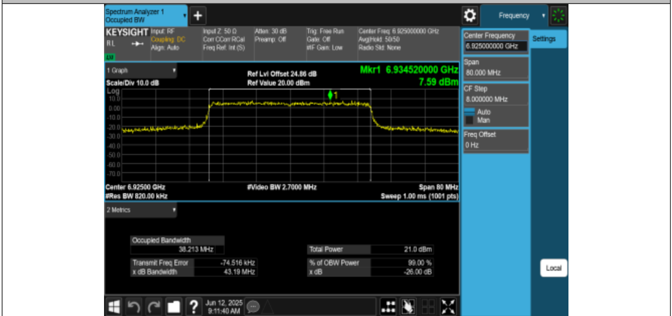
11AX40MIMO-Ant3-6925-PASS
