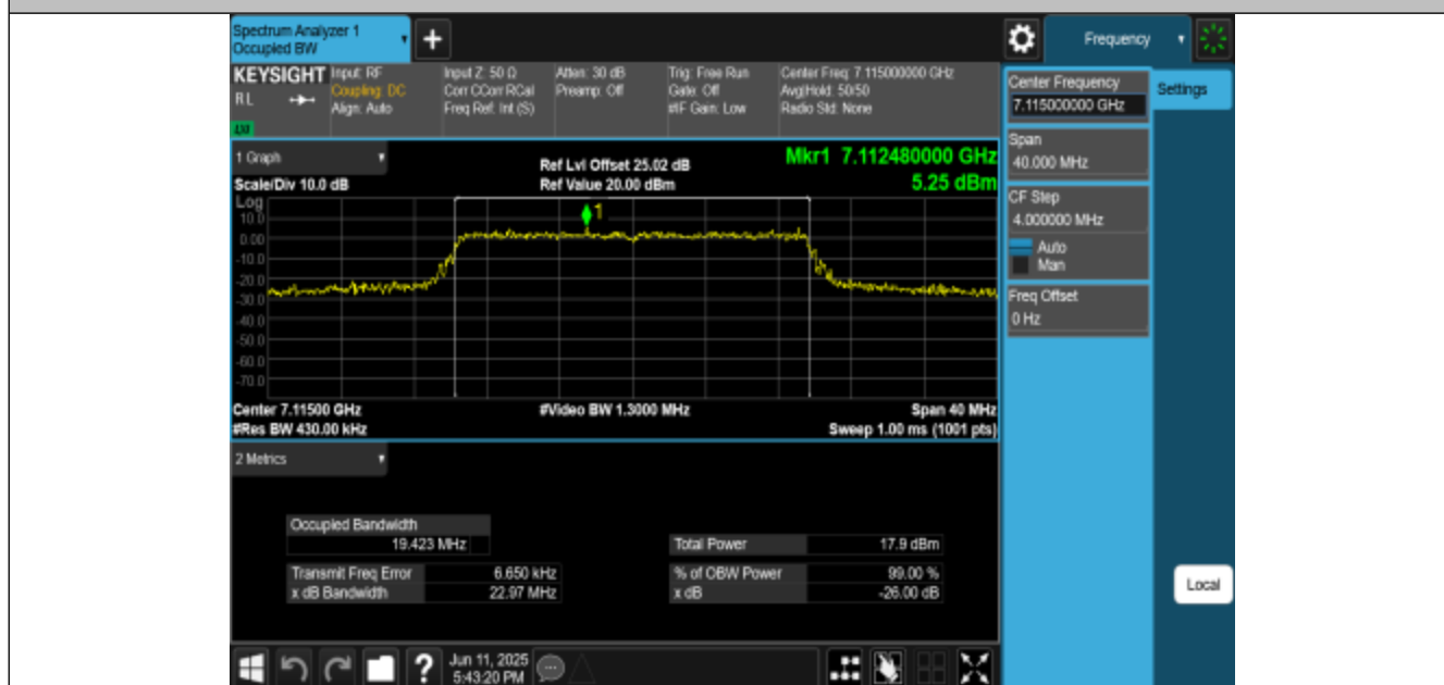
11AX20MIMO-Ant3-7115-PASS
