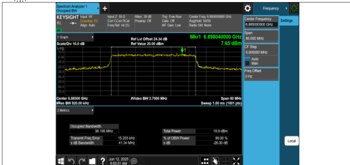
11AX40MIMO-Ant0-6885-PASS
