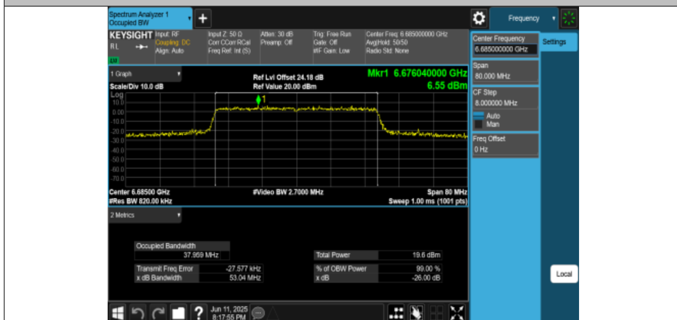
11AX40MIMO-Ant1-6685-PASS
