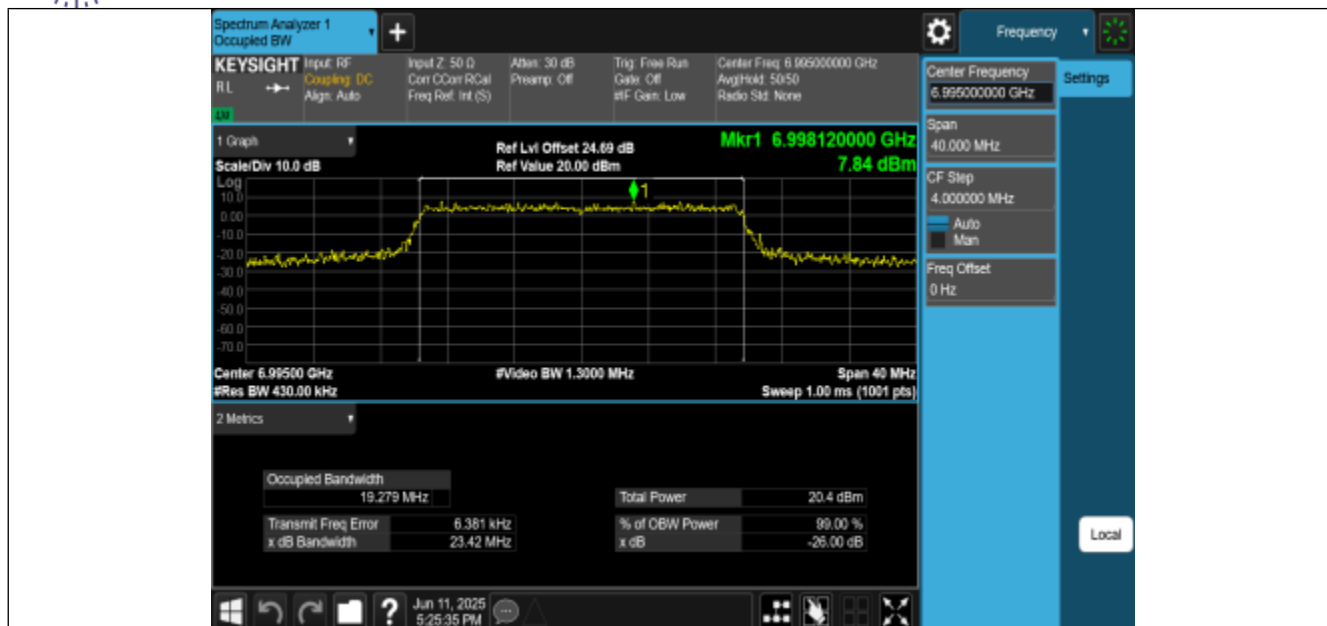
11AX20MIMO-Ant0-6995-PASS
