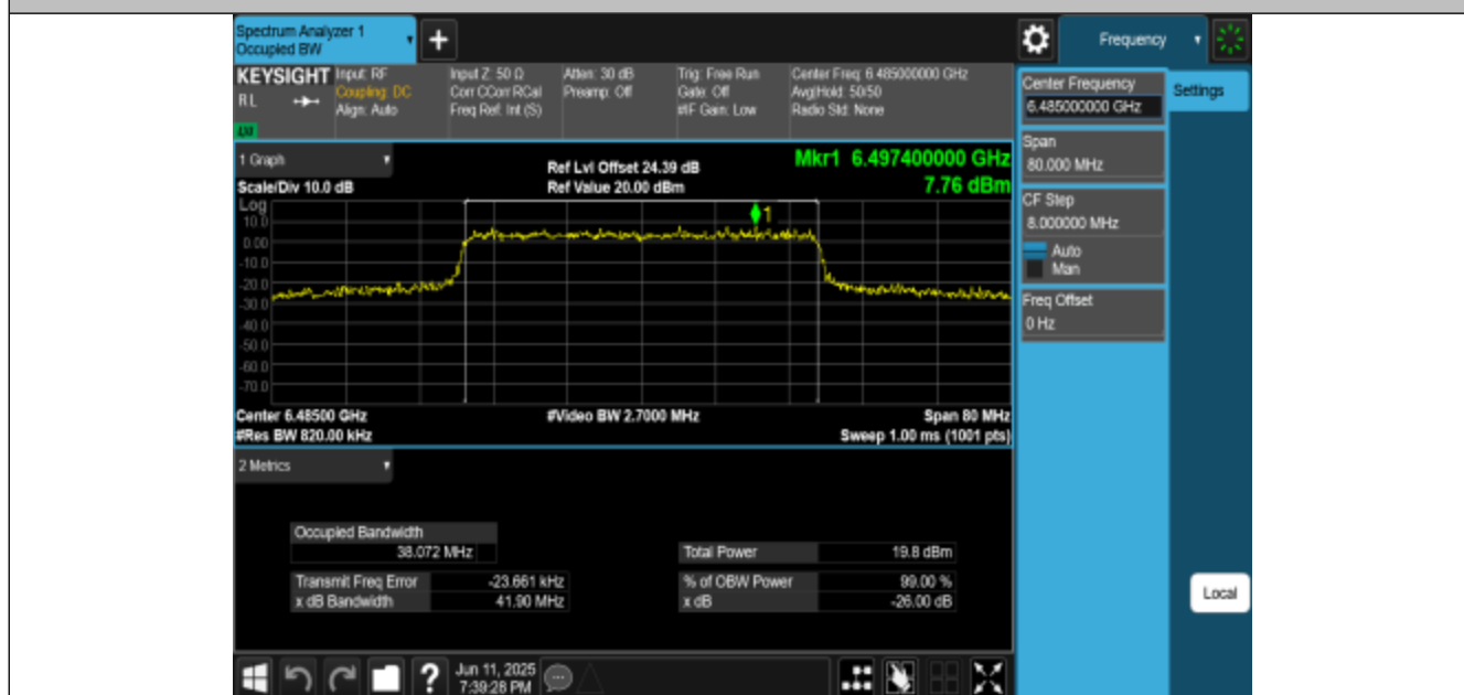
11AX40MIMO-Ant1-6485-PASS
