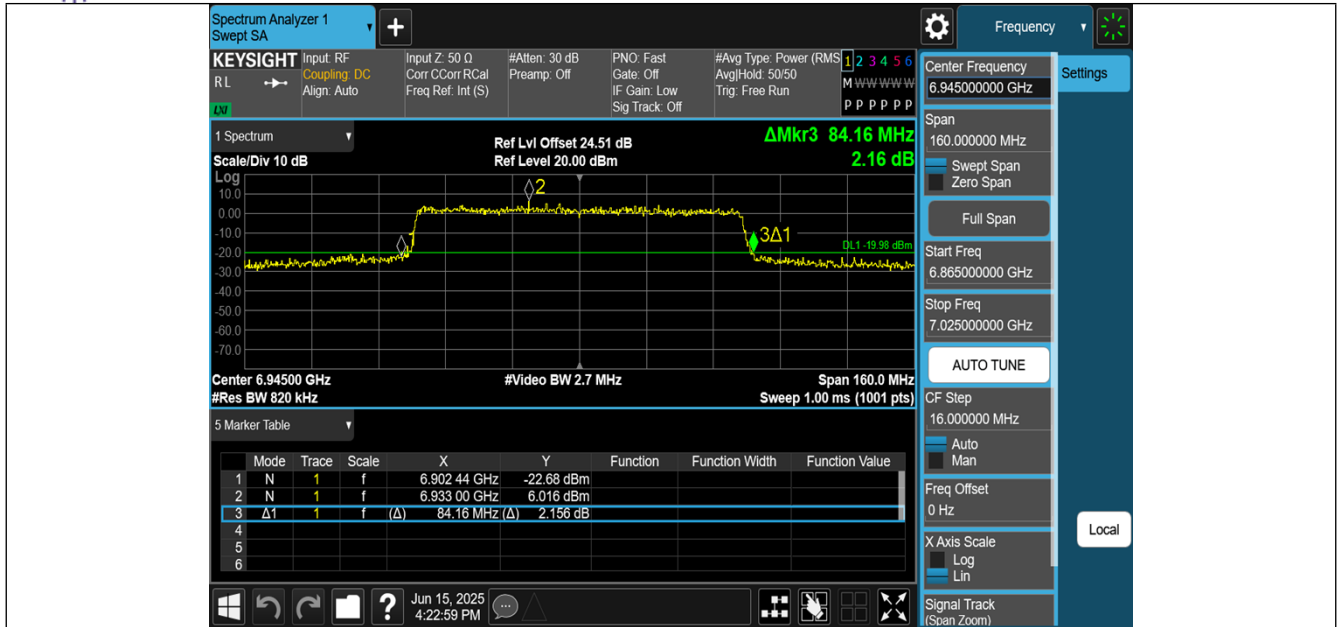
11BE80MIMO-Ant0-6945
