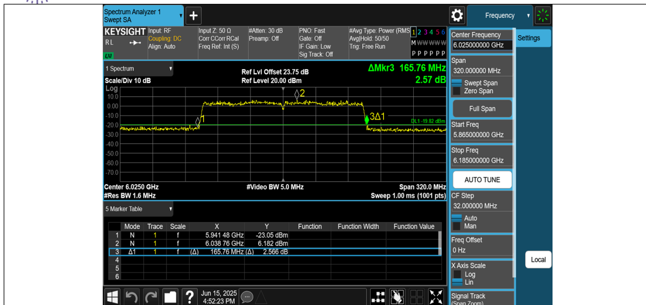
11BE160MIMO-Ant3-6025
