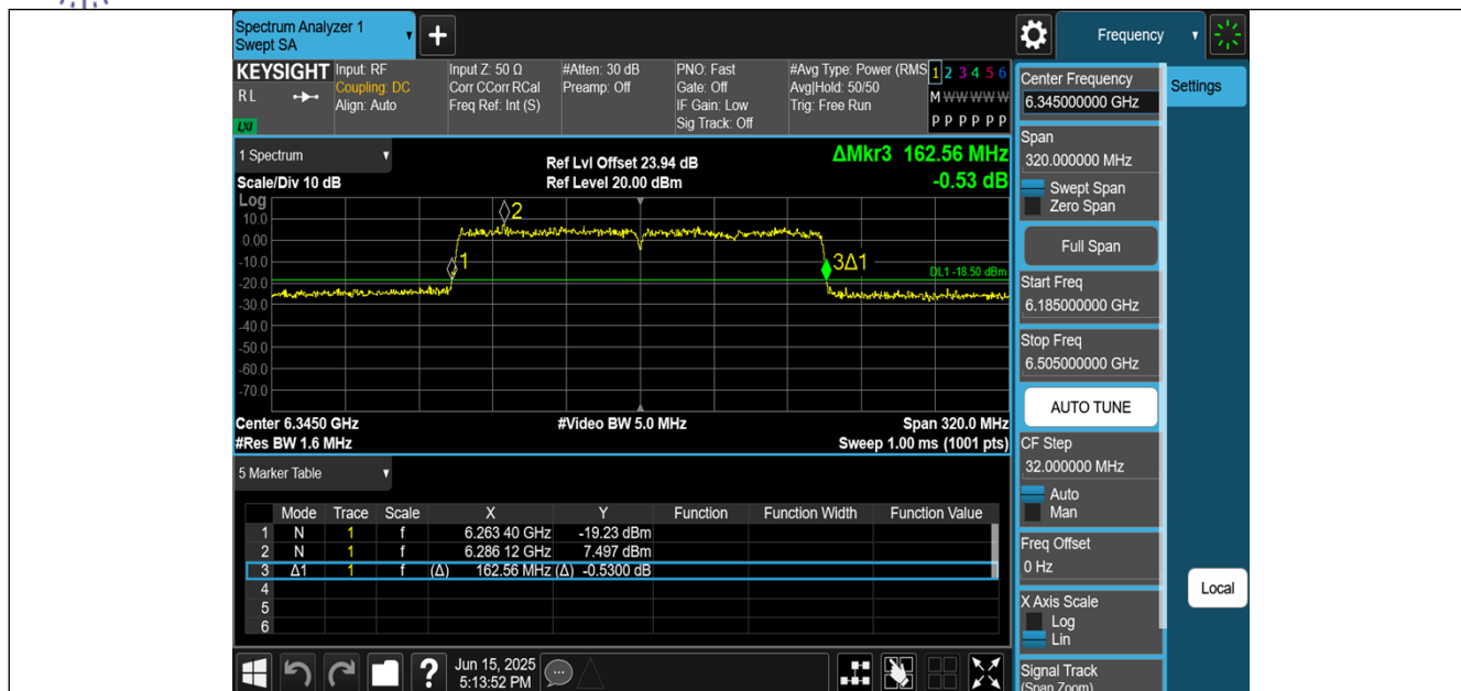
11BE160MIMO-Ant0-6345
