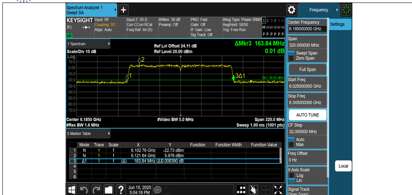
11BE160MIMO-Ant0-6185
