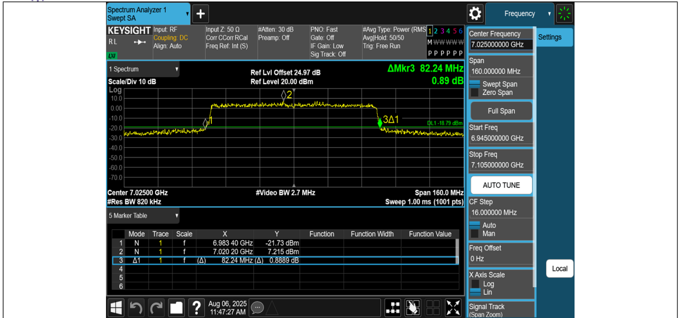
11BE80MIMO-Ant1-7025
