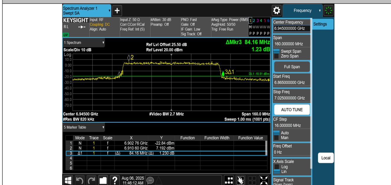
11BE80MIMO-Ant3-6945
