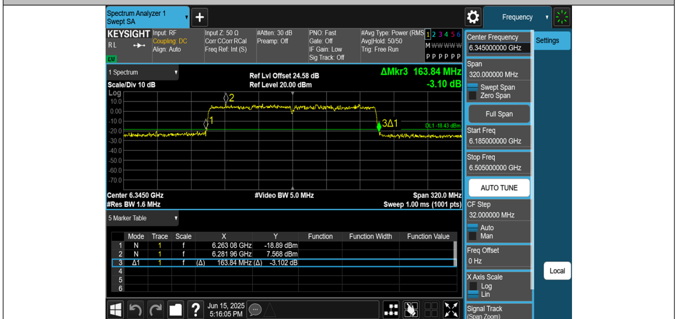
11BE160MIMO-Ant3-6345
