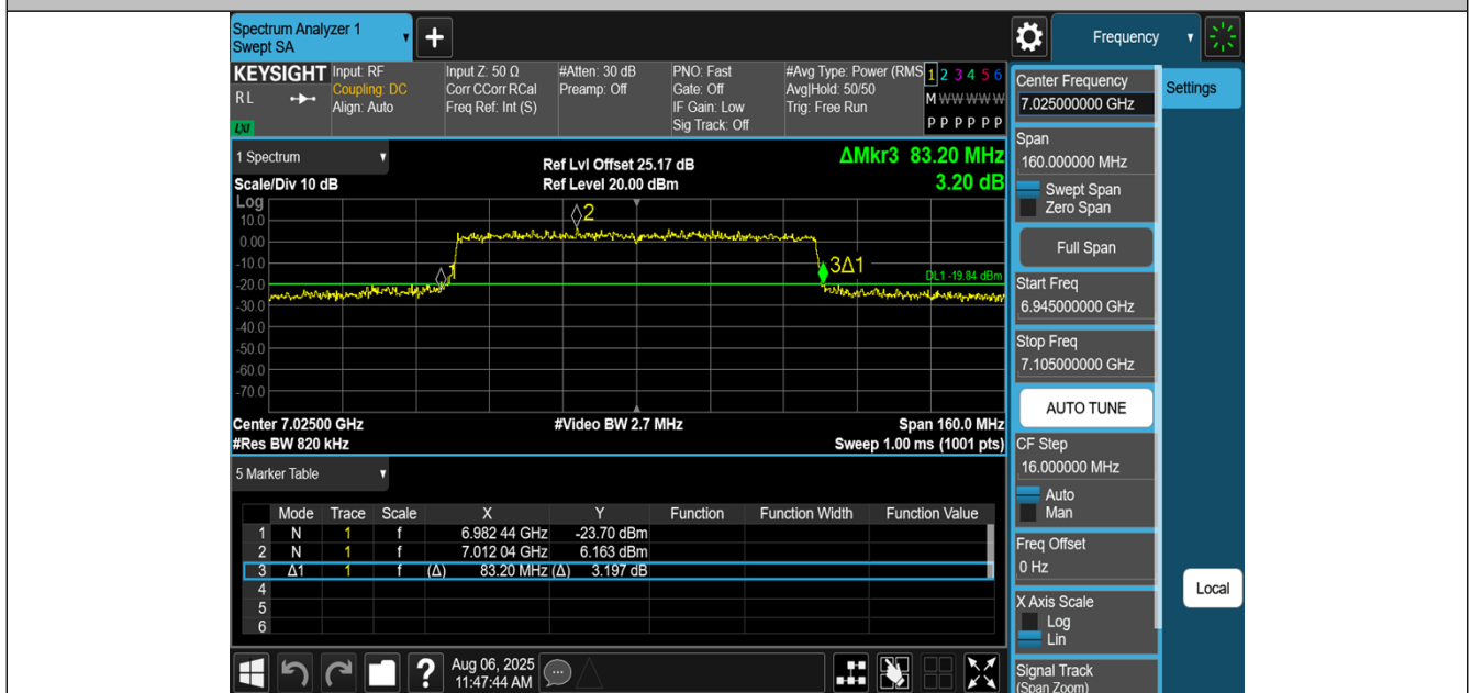
11BE80MIMO-Ant3-7025
