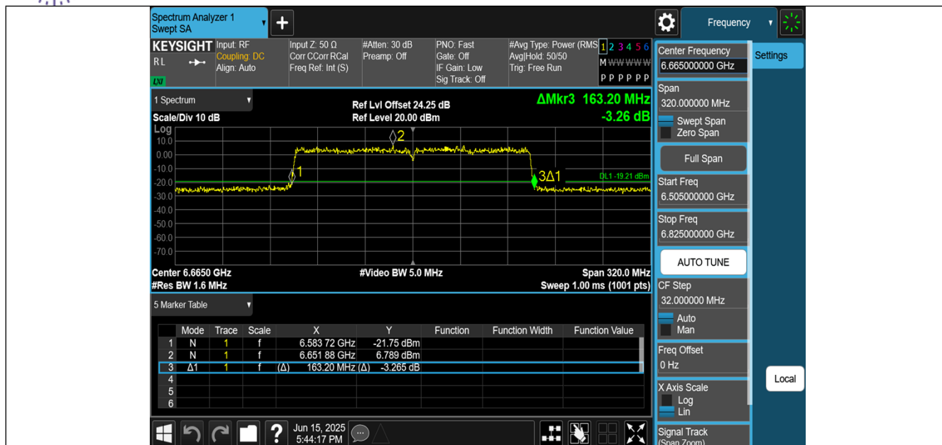
11BE160MIMO-Ant1-6665
