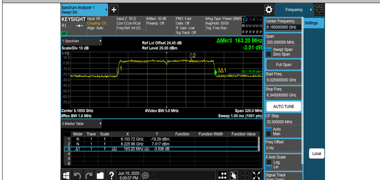
11BE160MIMO-Ant3-6185
