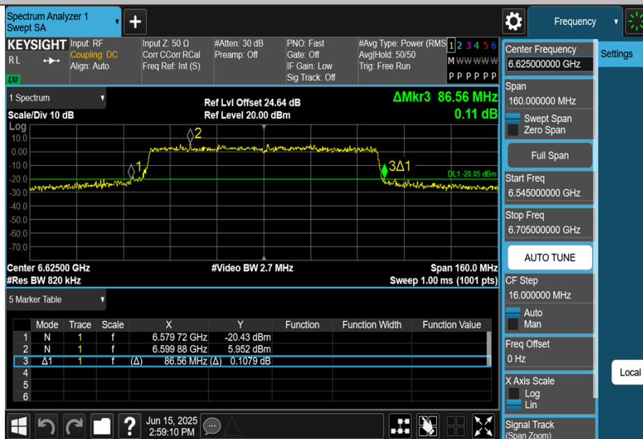
11BE80MIMO-Ant3-6625
