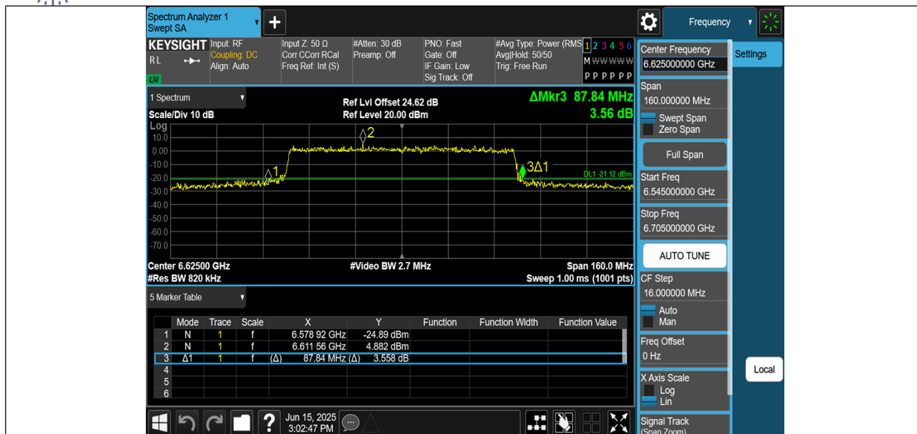
11BE80MIMO-Ant0-6625
