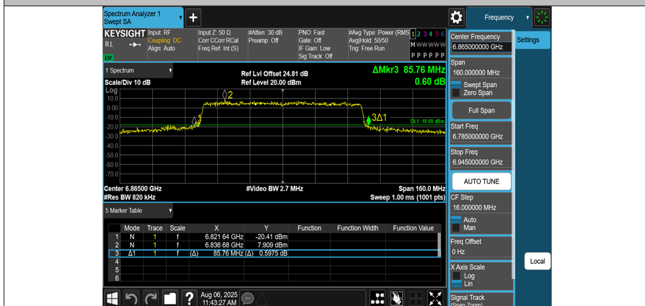
11BE80MIMO-Ant0-6865
