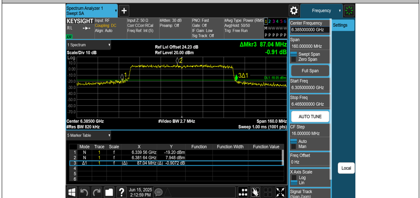
11BE80MIMO-Ant0-6385
