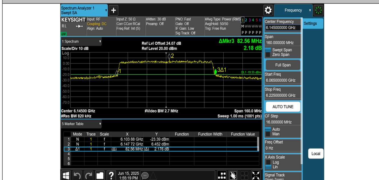
11BE80MIMO-Ant3-6145
