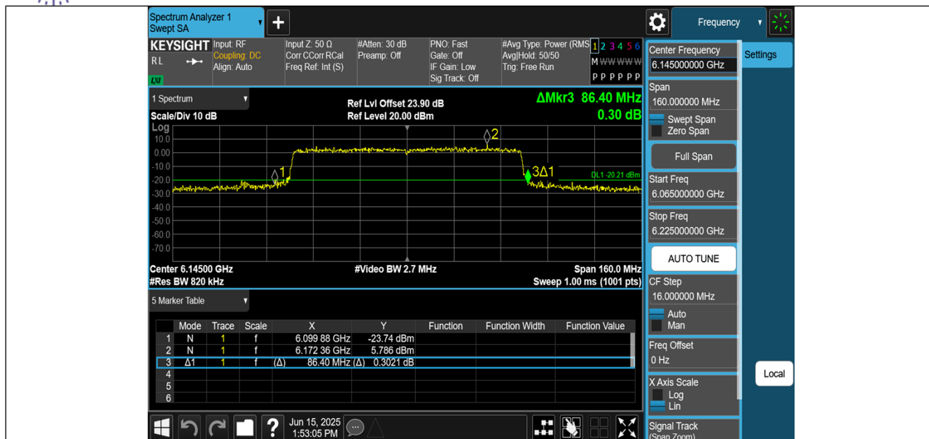
11BE80MIMO-Ant0-6145
