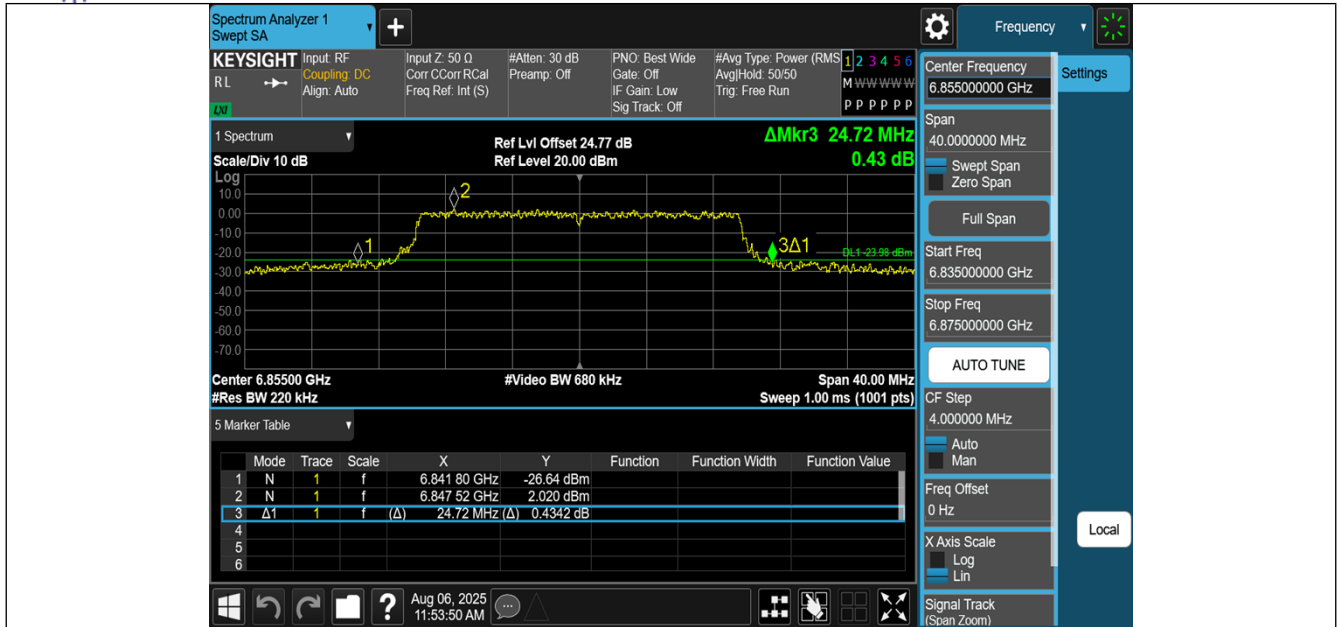
11BE20MIMO-Ant0-6855
