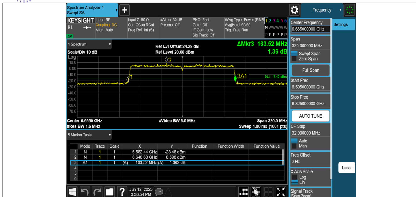
11AX160MIMO-Ant0-6665
