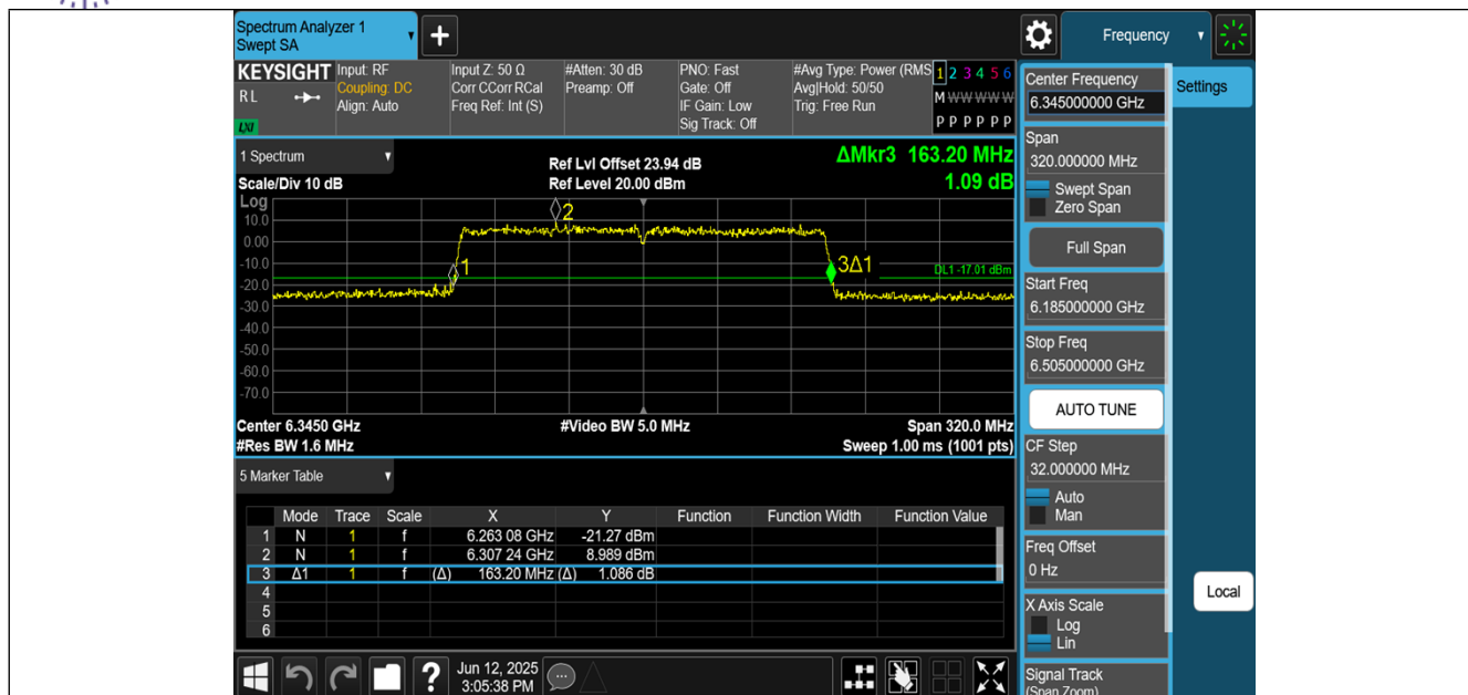
11AX160MIMO-Ant0-6345
