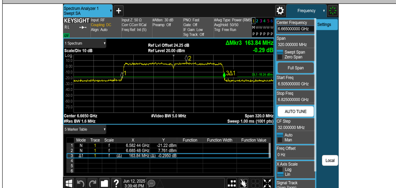
11AX160MIMO-Ant1-6665
