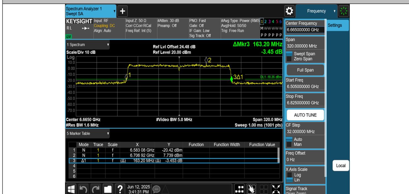
11AX160MIMO-Ant3-6665
