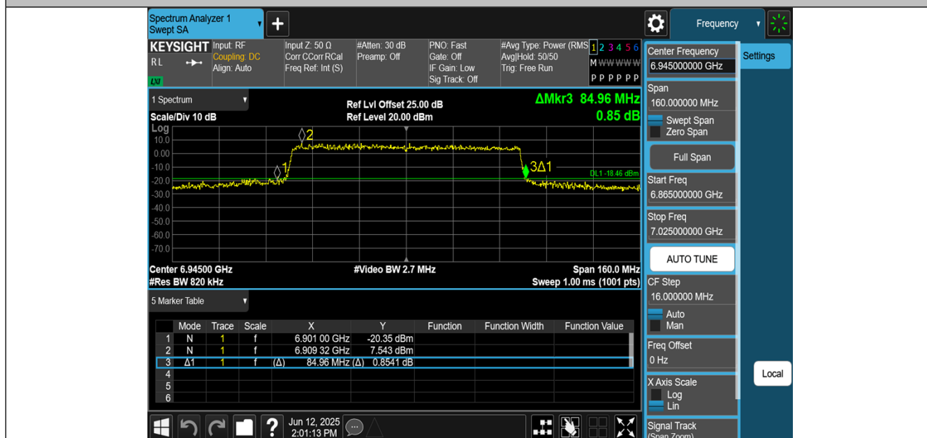
11AX80MIMO-Ant3-6945
