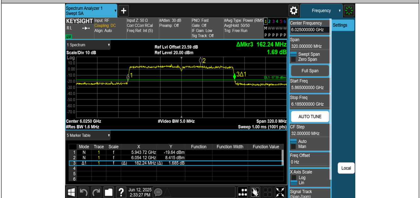
11AX160MIMO-Ant1-6025
