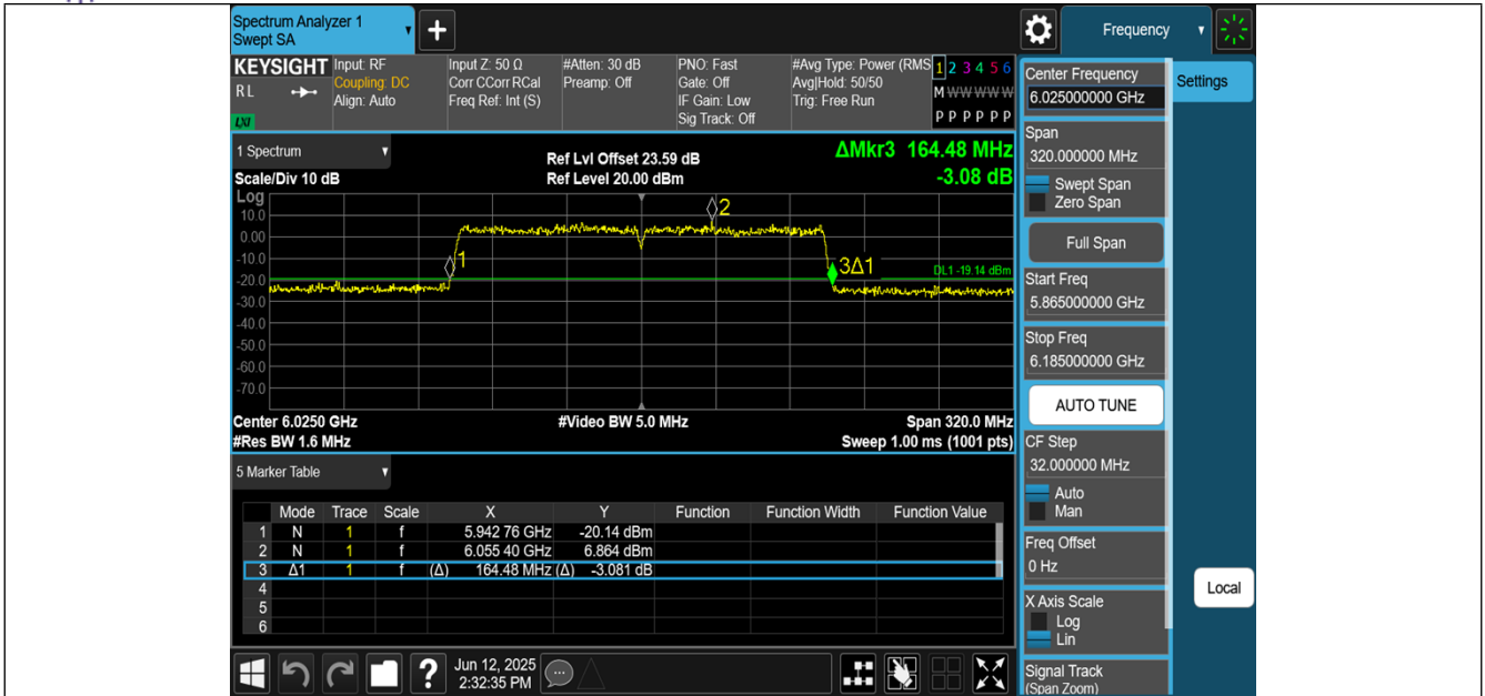
11AX160MIMO-Ant0-6025
