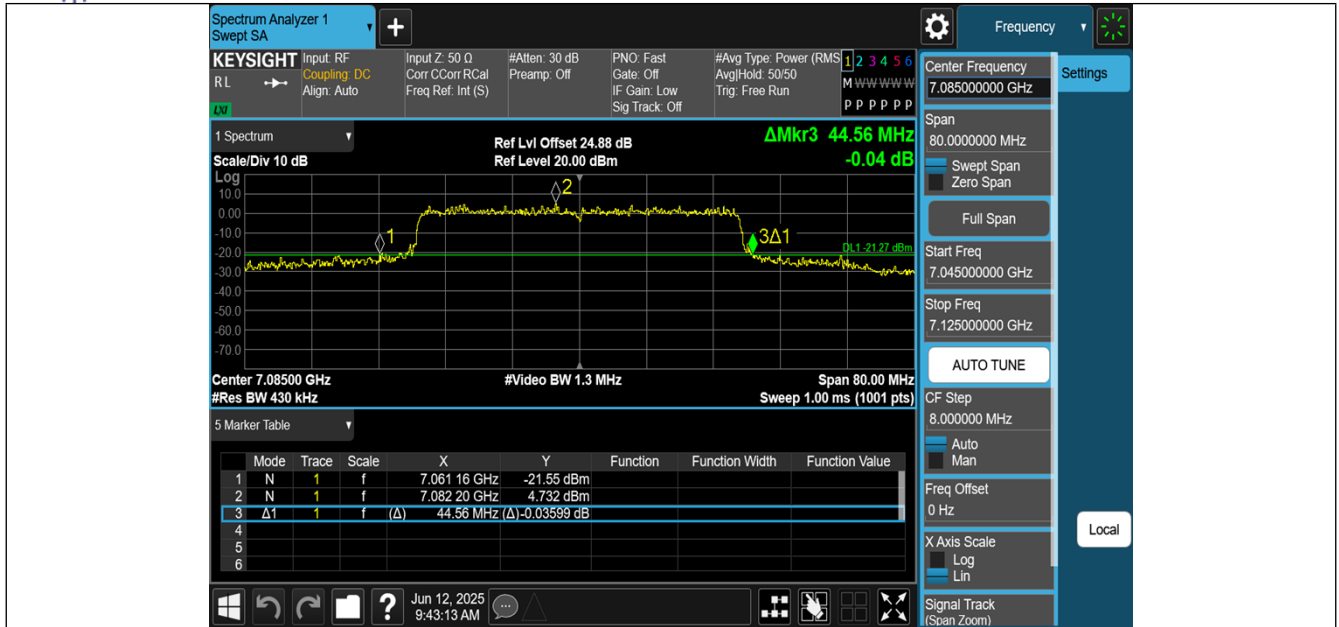
11AX40MIMO-Ant2-7085
