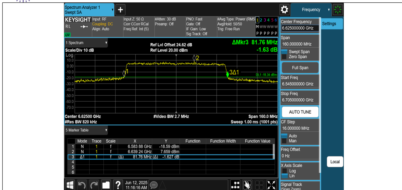
11AX80MIMO-Ant0-6625
