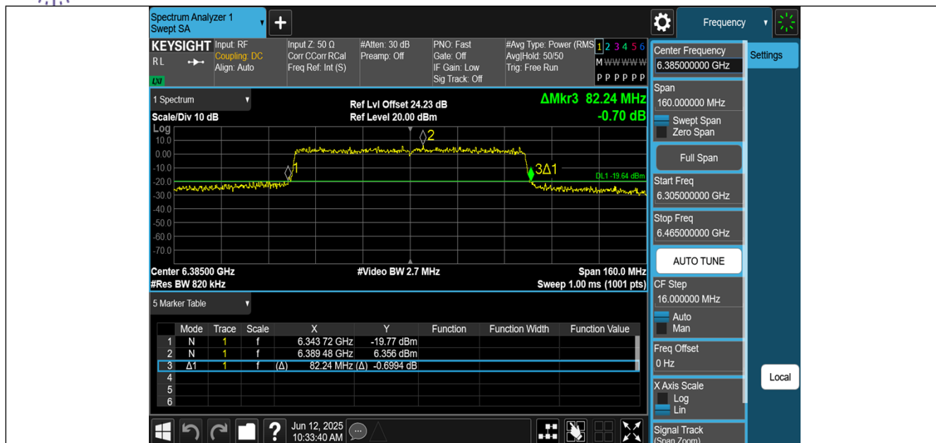
11AX80MIMO-Ant0-6385
