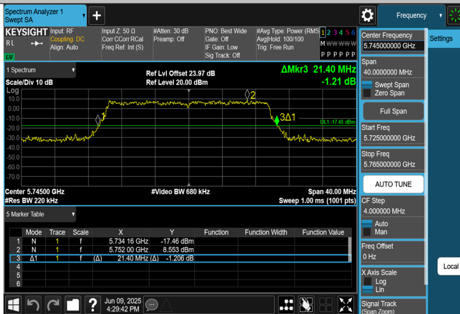
11BE20MIMO-Ant1-5745
