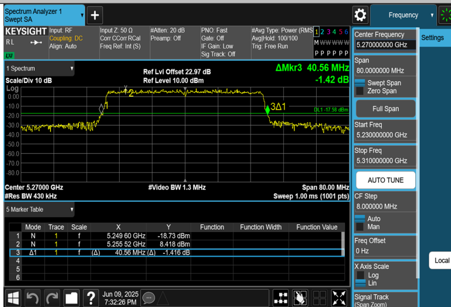
11BE40MIMO-Ant1-5270
