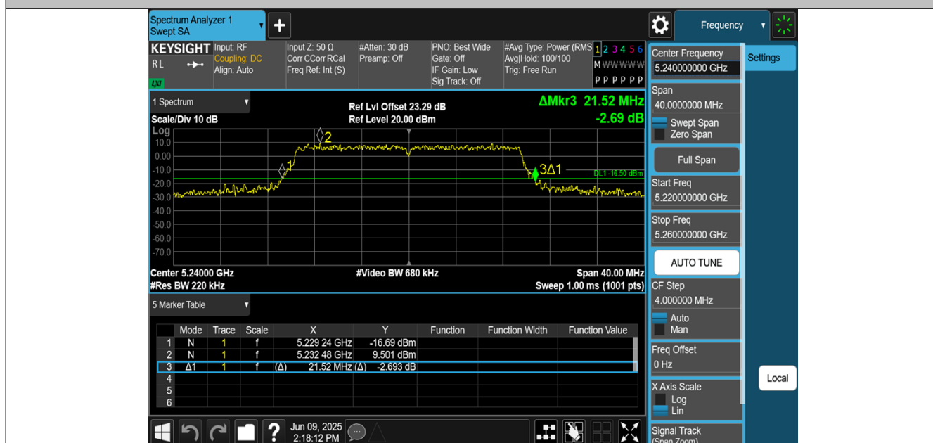
11BE20MIMO-Ant3-5240
