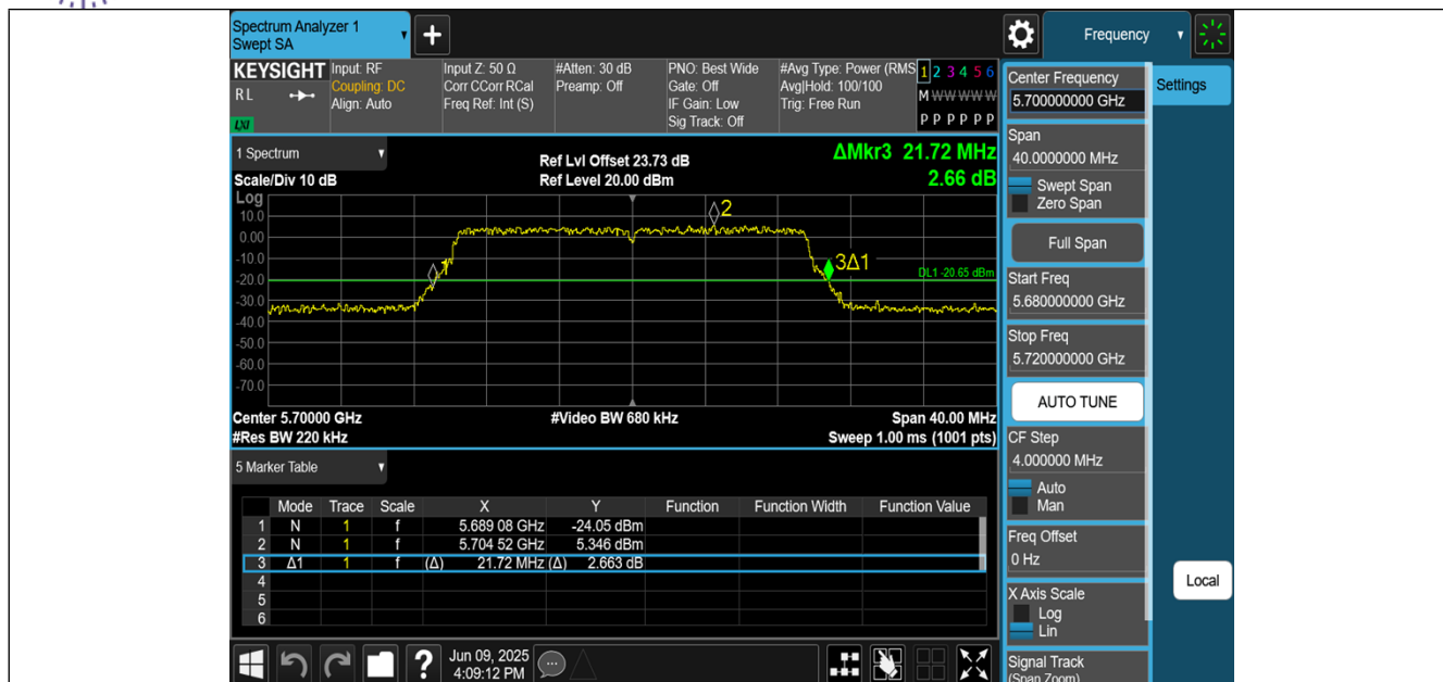
11BE20MIMO-Ant2-5700
