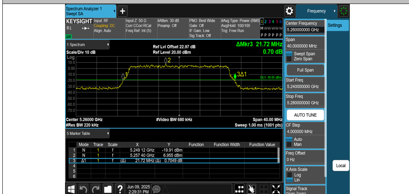
11BE20MIMO-Ant1-5260
