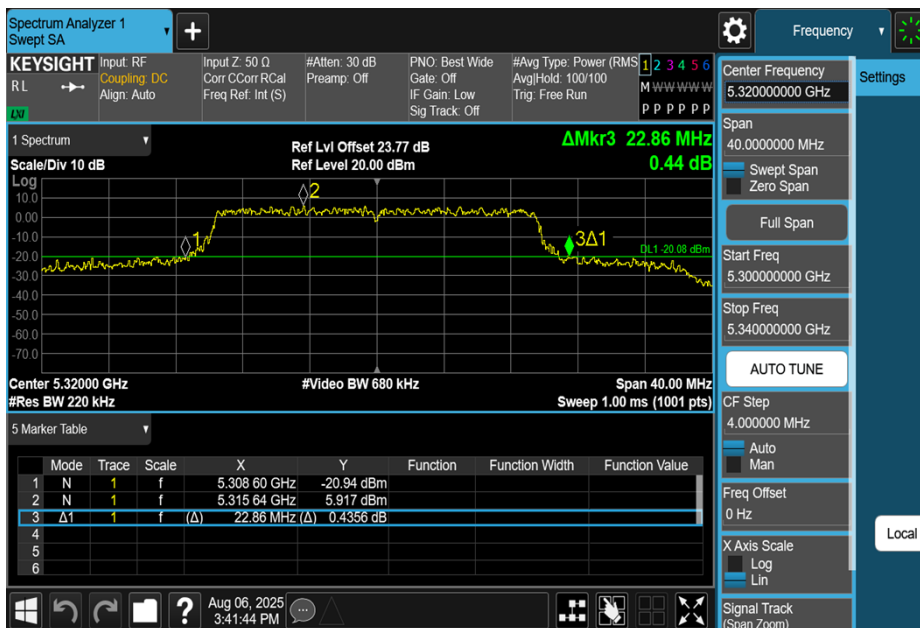
11BE20MIMO-Ant0-5320
