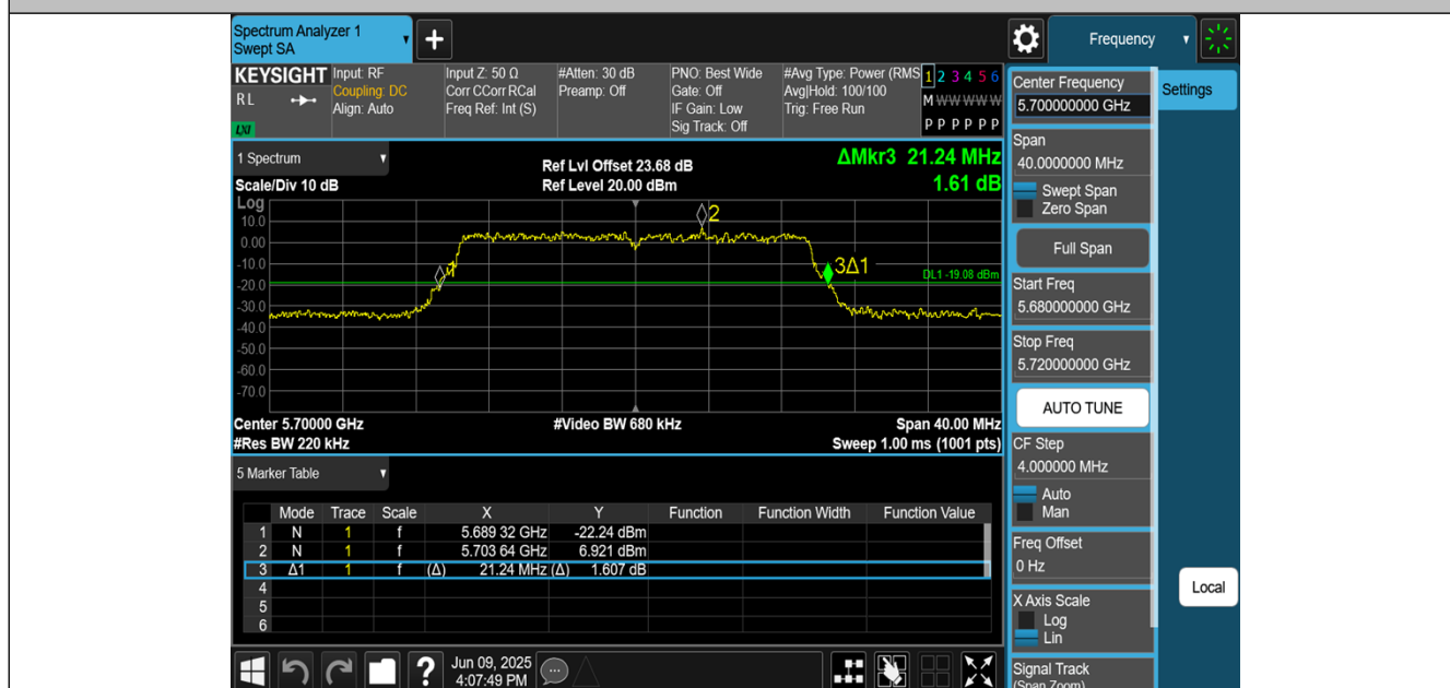
11BE20MIMO-Ant1-5700
