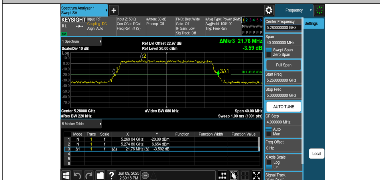
11BE20MIMO-Ant1-5280
