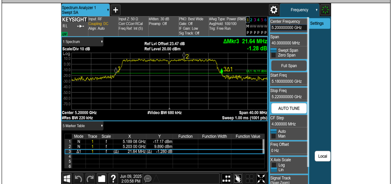
11BE20MIMO-Ant2-5200
