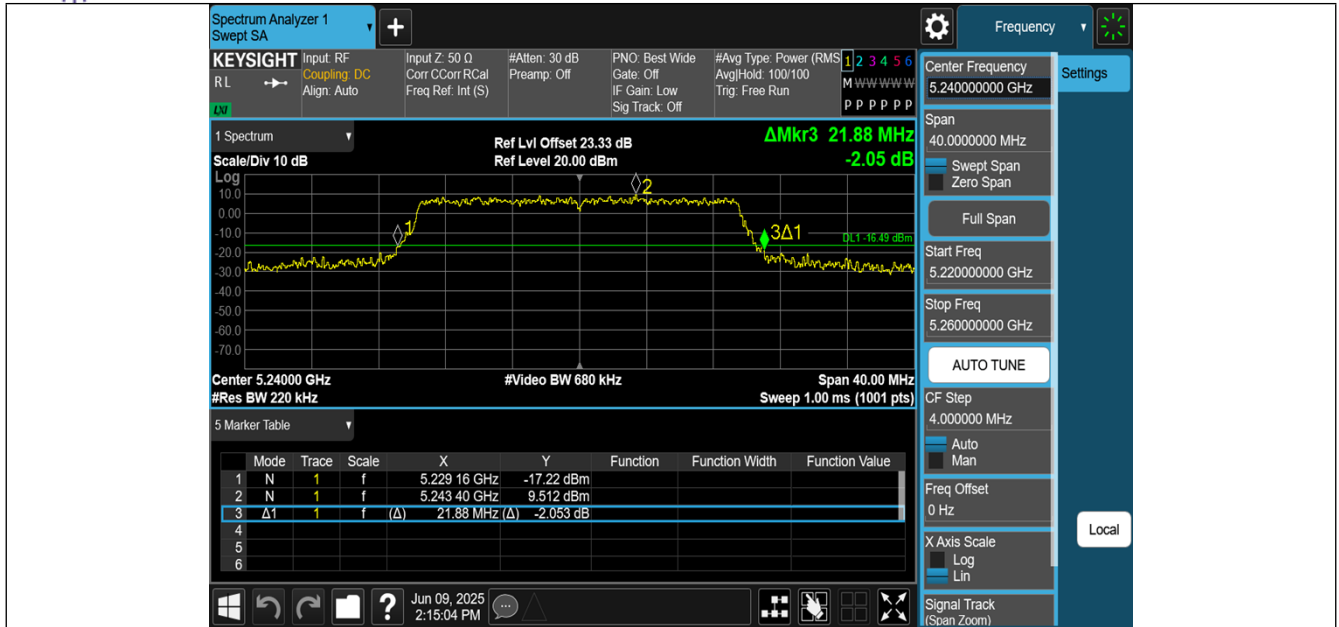
11BE20MIMO-Ant0-5240
