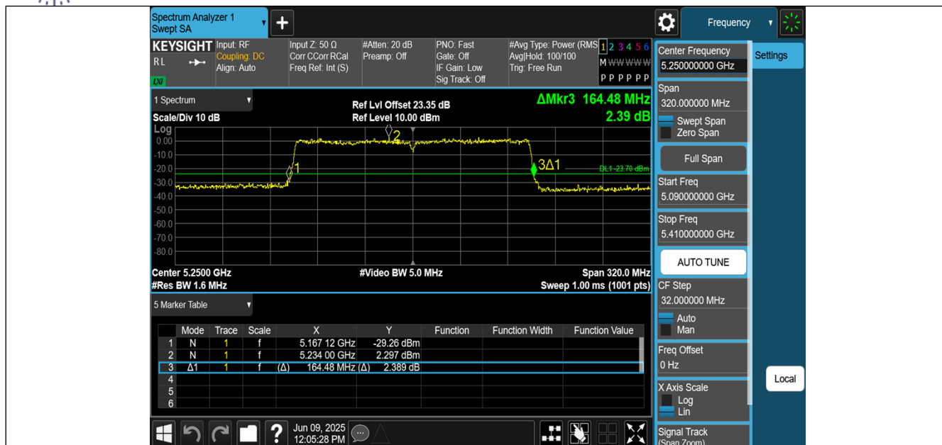
11AX160MIMO-Ant0-5250
