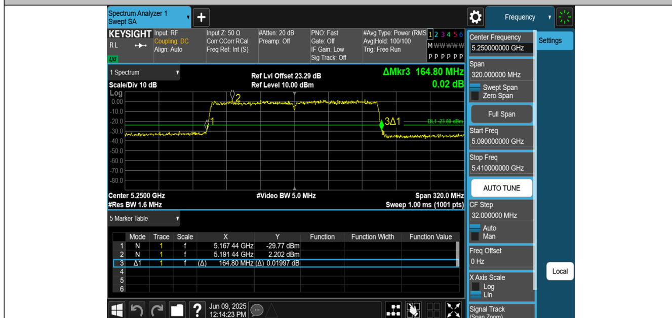
11AX160MIMO-Ant3-5250
