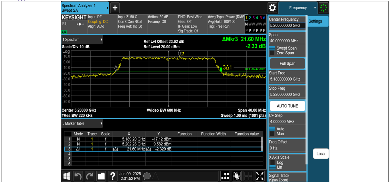
11BE20MIMO-Ant0-5200
