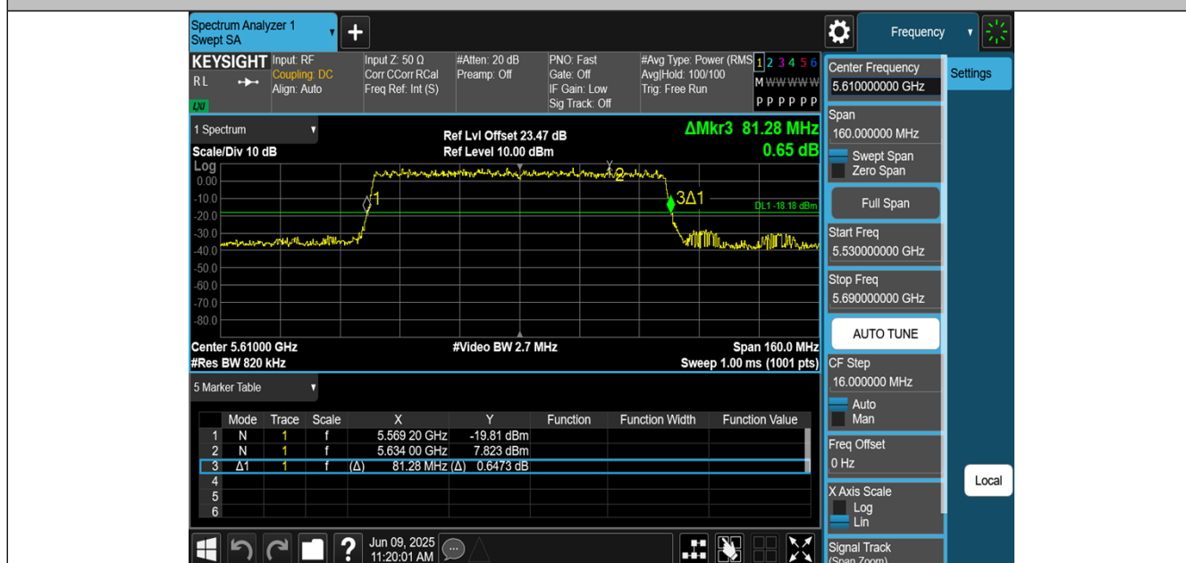
11AX80MIMO-Ant1-5610
