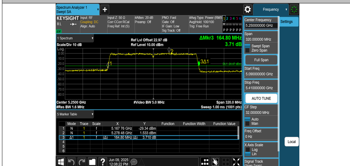
11AX160MIMO-Ant1-5250
