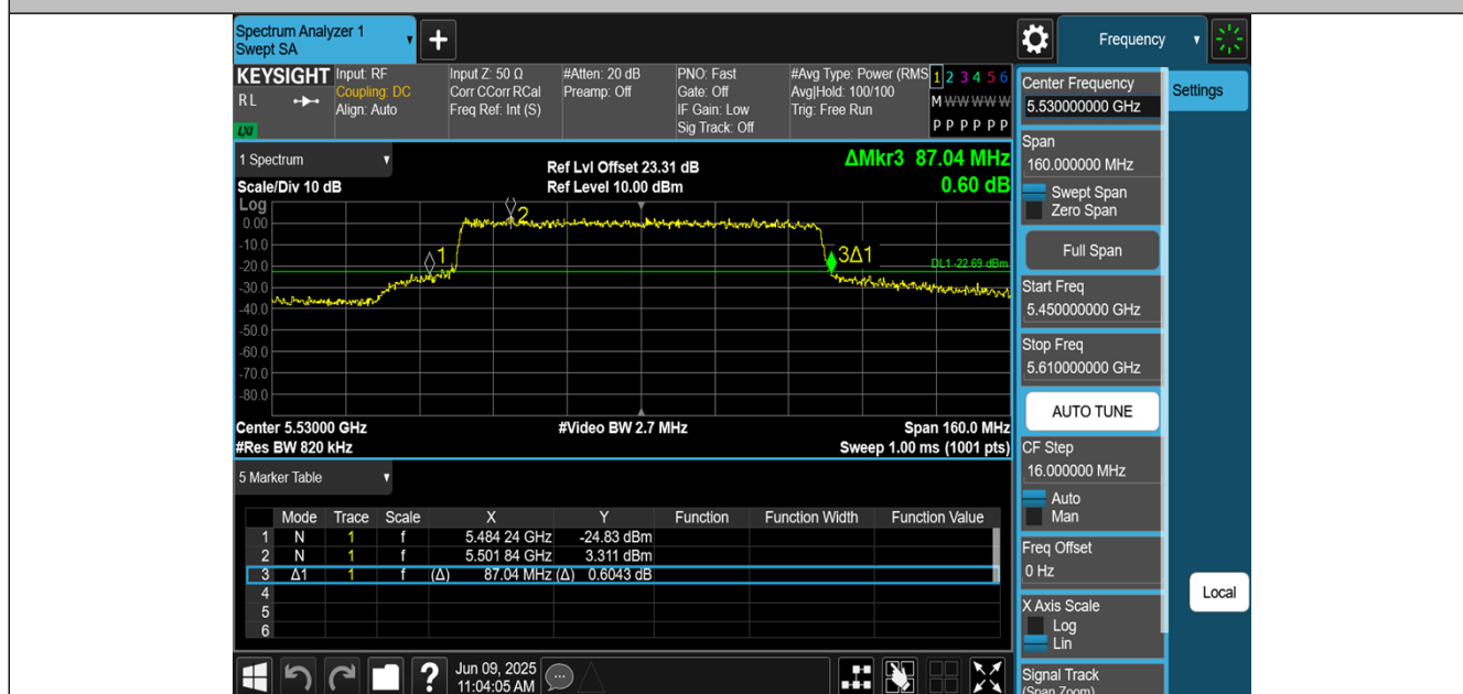
11AX80MIMO-Ant1-5530
