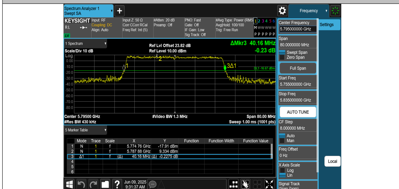
11AX40MIMO-Ant1-5795
