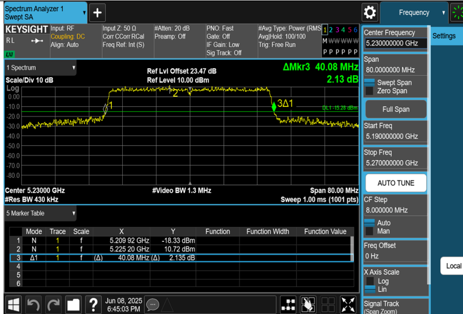
11AX40MIMO-Ant2-5230
