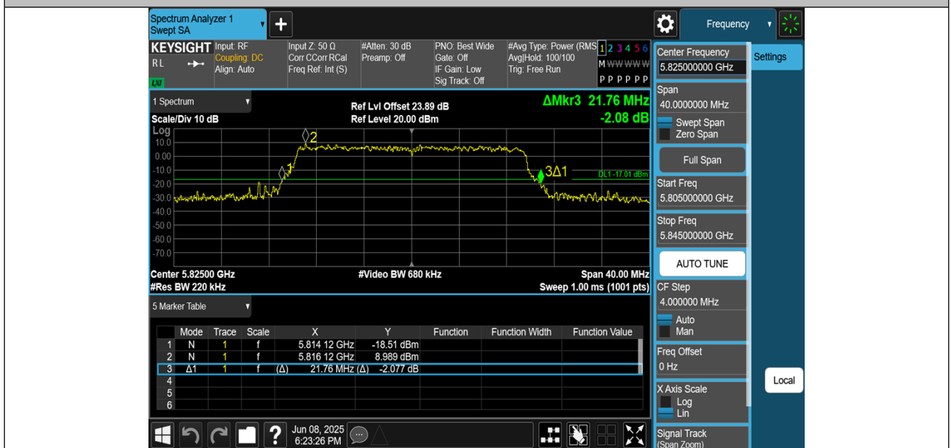
11AX20MIMO-Ant3-5825
