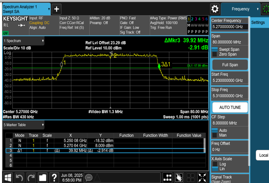
11AX40MIMO-Ant3-5270
