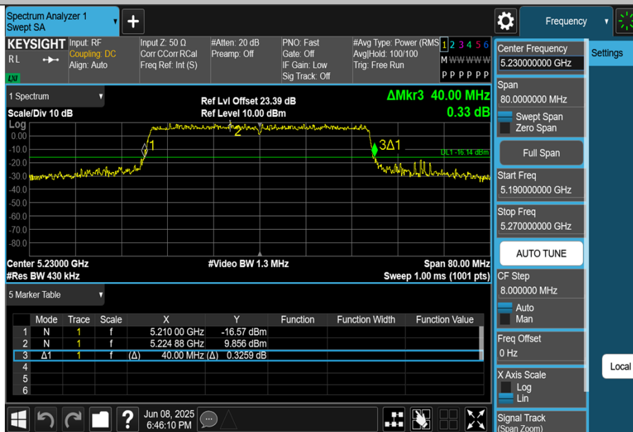
11AX40MIMO-Ant3-5230
