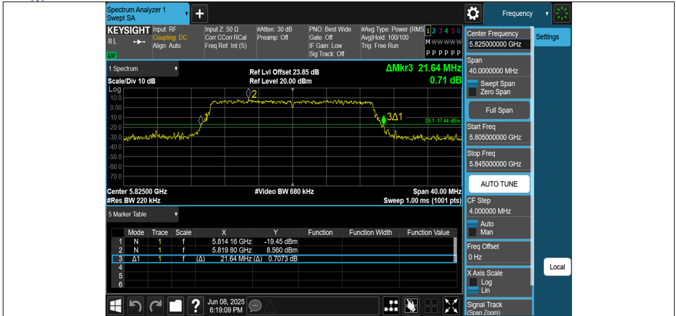
11AX20MIMO-Ant2-5825
