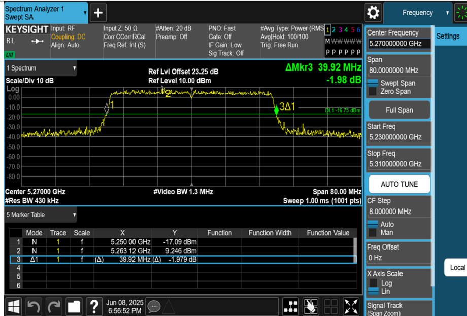
11AX40MIMO-Ant2-5270
