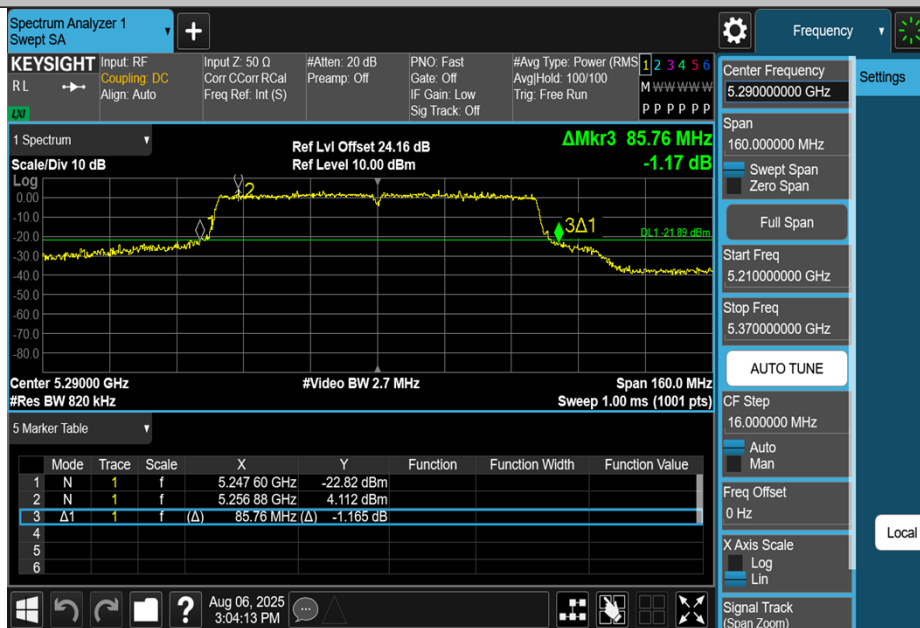
11AC80MIMO-Ant1-5290
