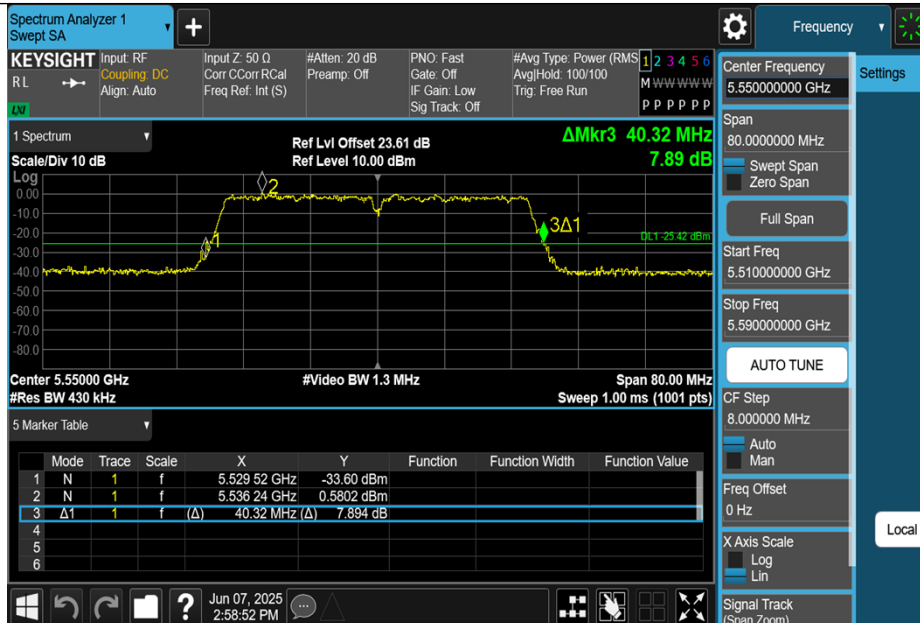
11AC40MIMO-Ant0-5550
