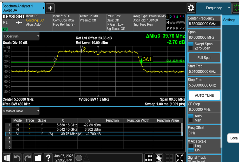
11AC40MIMO-Ant1-5550
