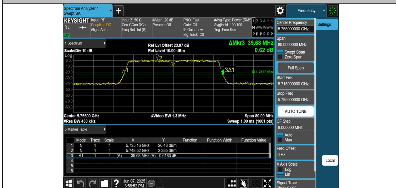
11AC40MIMO-Ant1-5755
