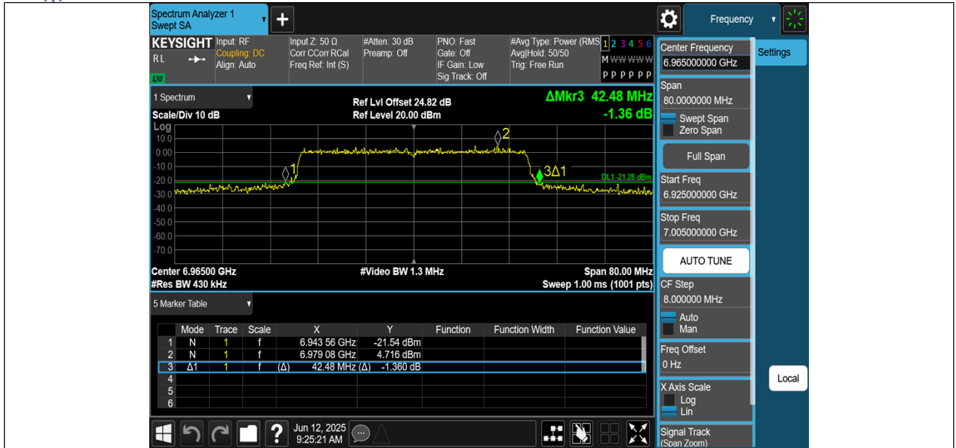
11AX40MIMO-Ant0-6965
