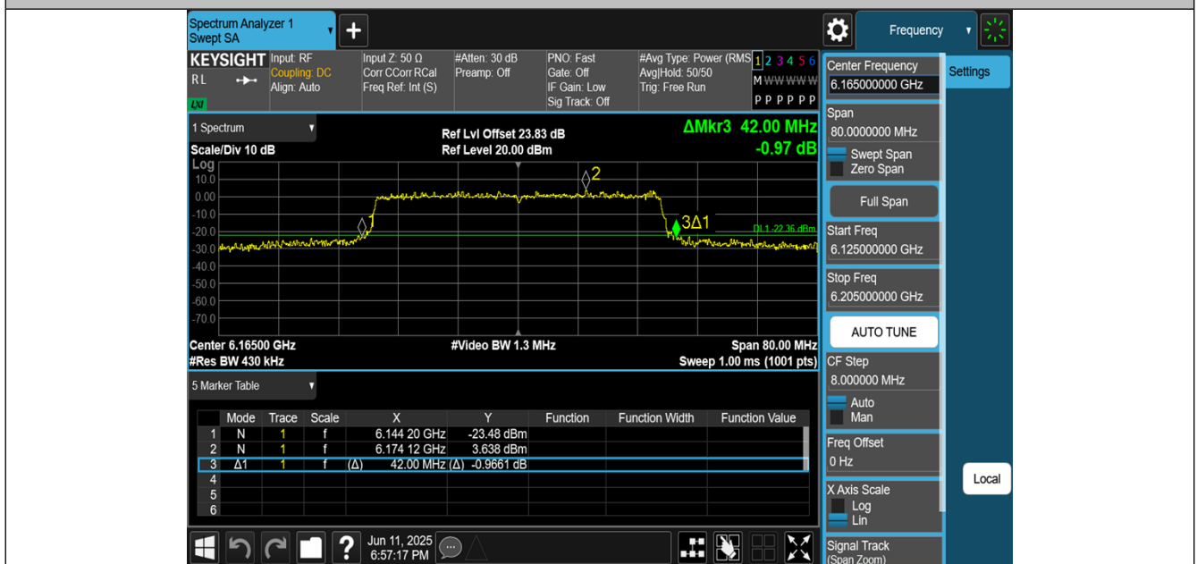
11AX40MIMO-Ant0-6165
