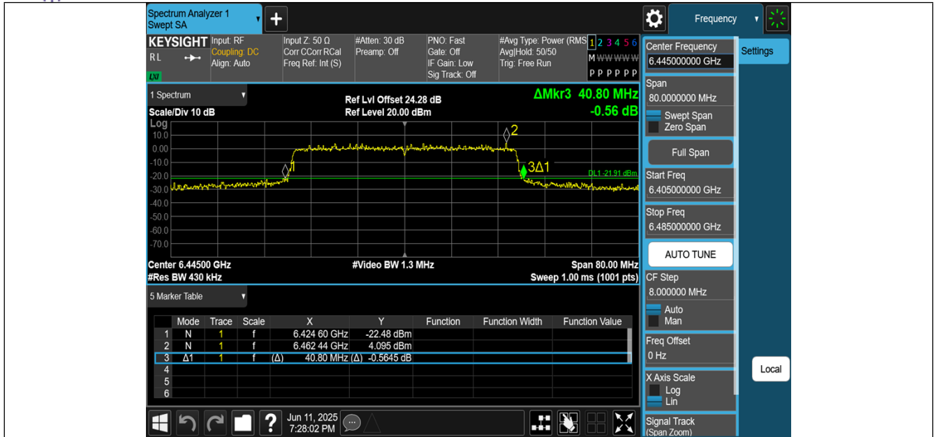
11AX40MIMO-Ant2-6445
