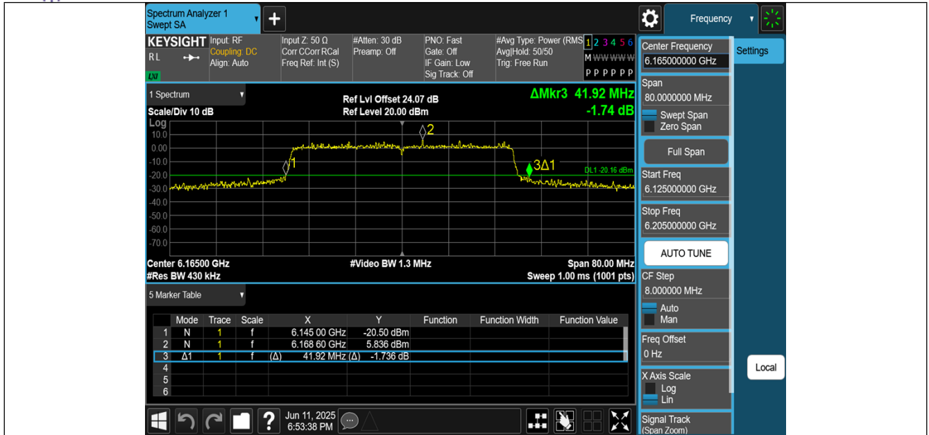
11AX40MIMO-Ant3-6165
