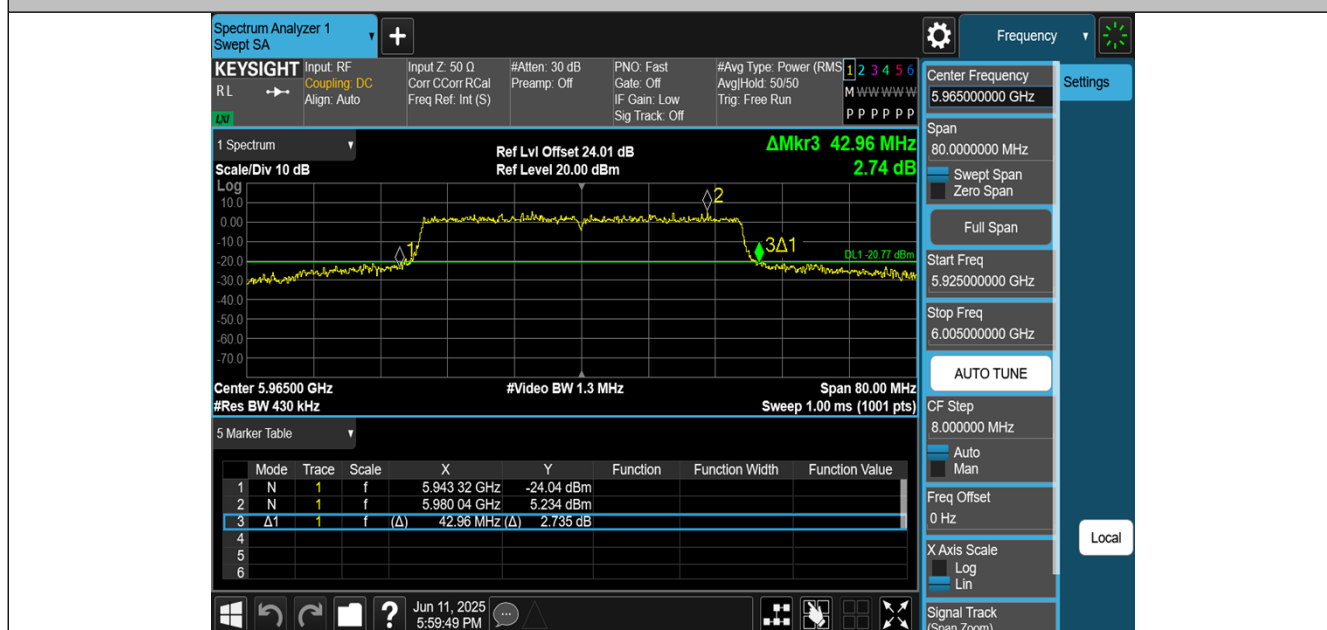
11AX40MIMO-Ant0-5965
