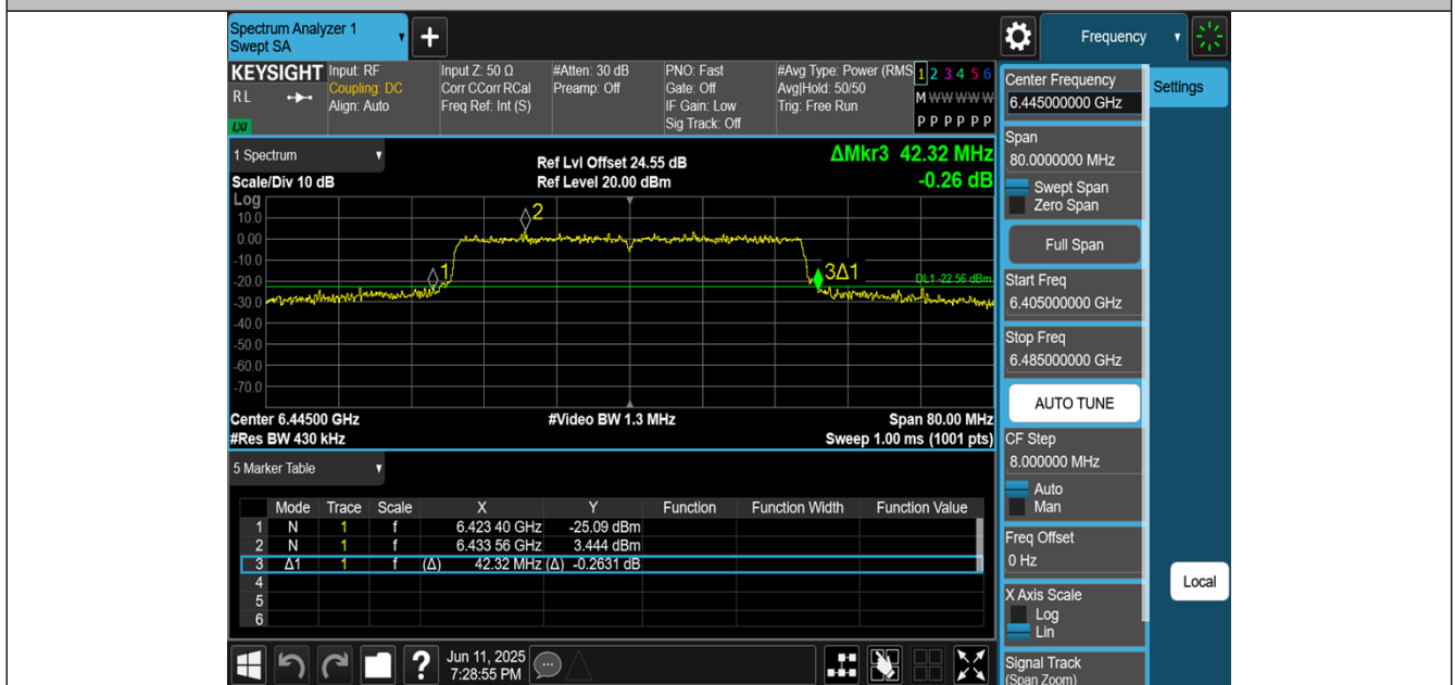
11AX40MIMO-Ant3-6445
