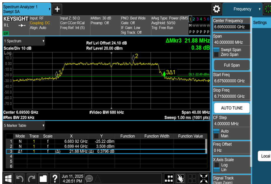
11AX20MIMO-Ant3-6695
