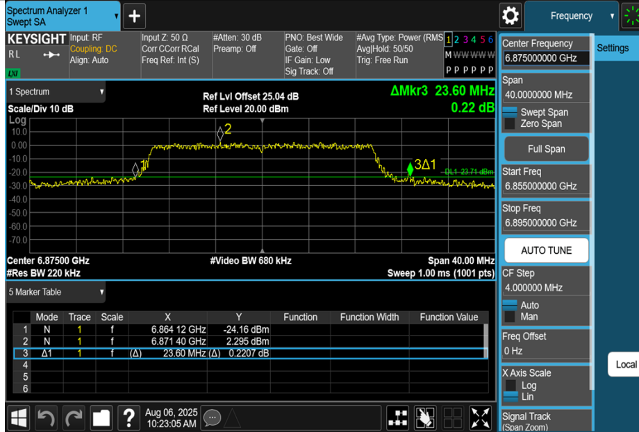
11AX20MIMO-Ant1-6875
