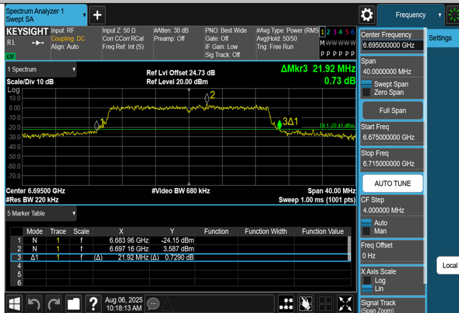
11AX20MIMO-Ant2-6695
