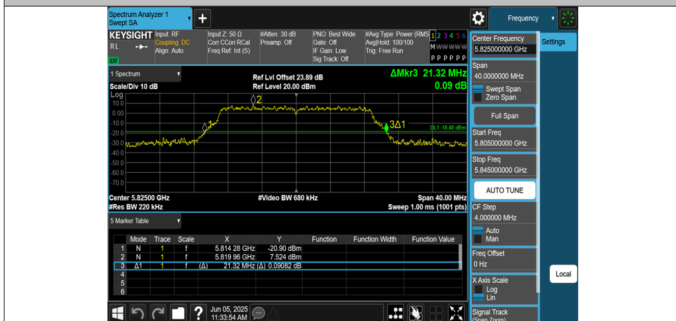
11N20MIMO-Ant3-5825
