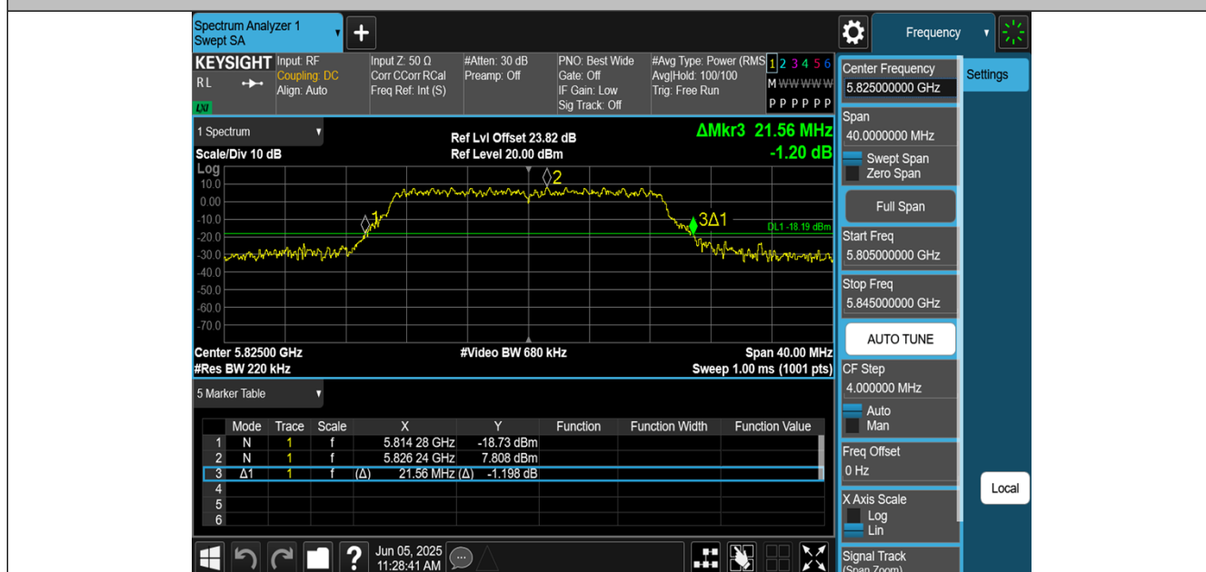
11N20MIMO-Ant1-5825
