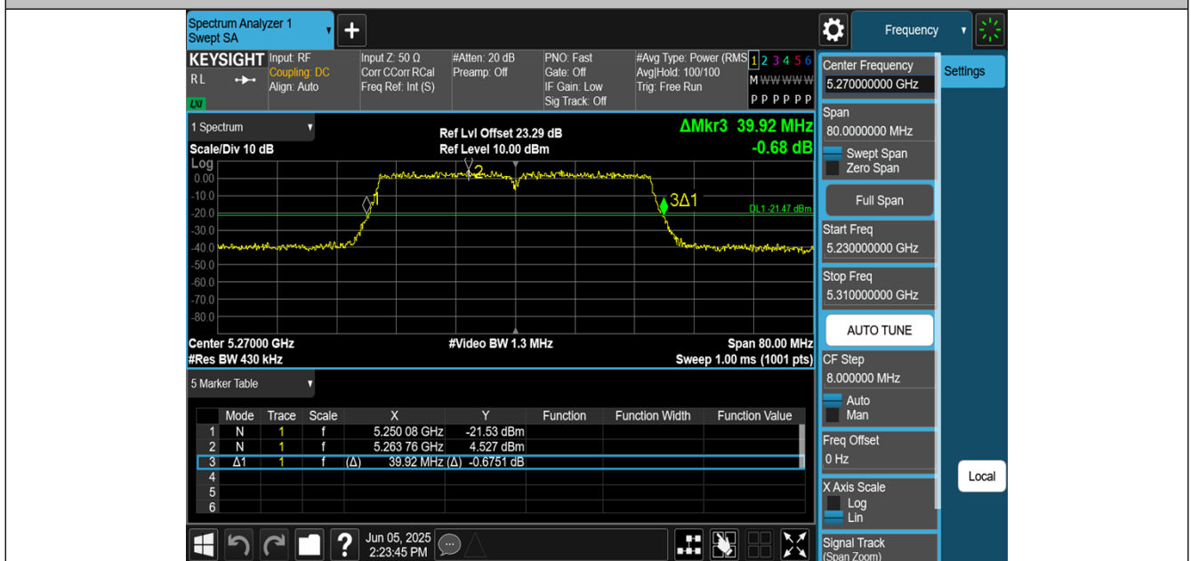
11N40MIMO-Ant3-5270
