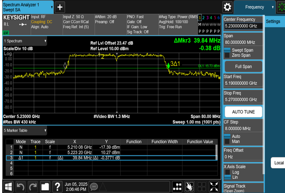
11N40MIMO-Ant2-5230
