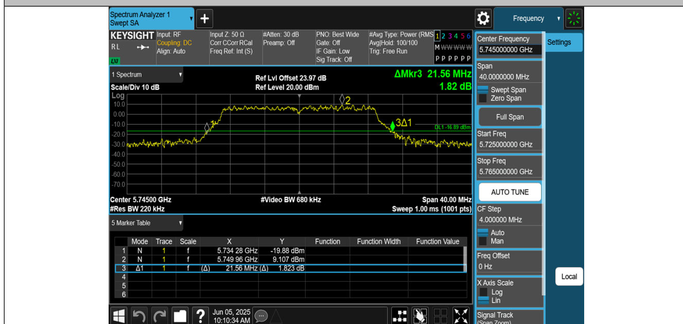
11N20MIMO-Ant1-5745
