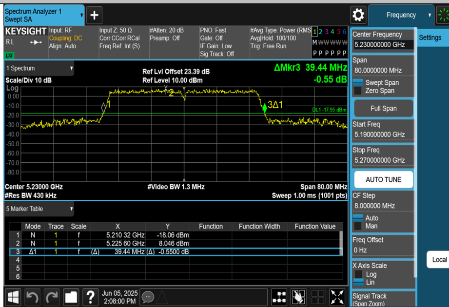
11N40MIMO-Ant3-5230
