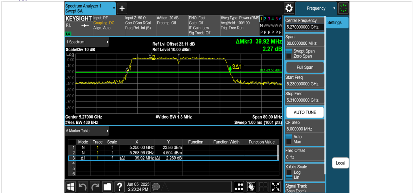
11N40MIMO-Ant0-5270
