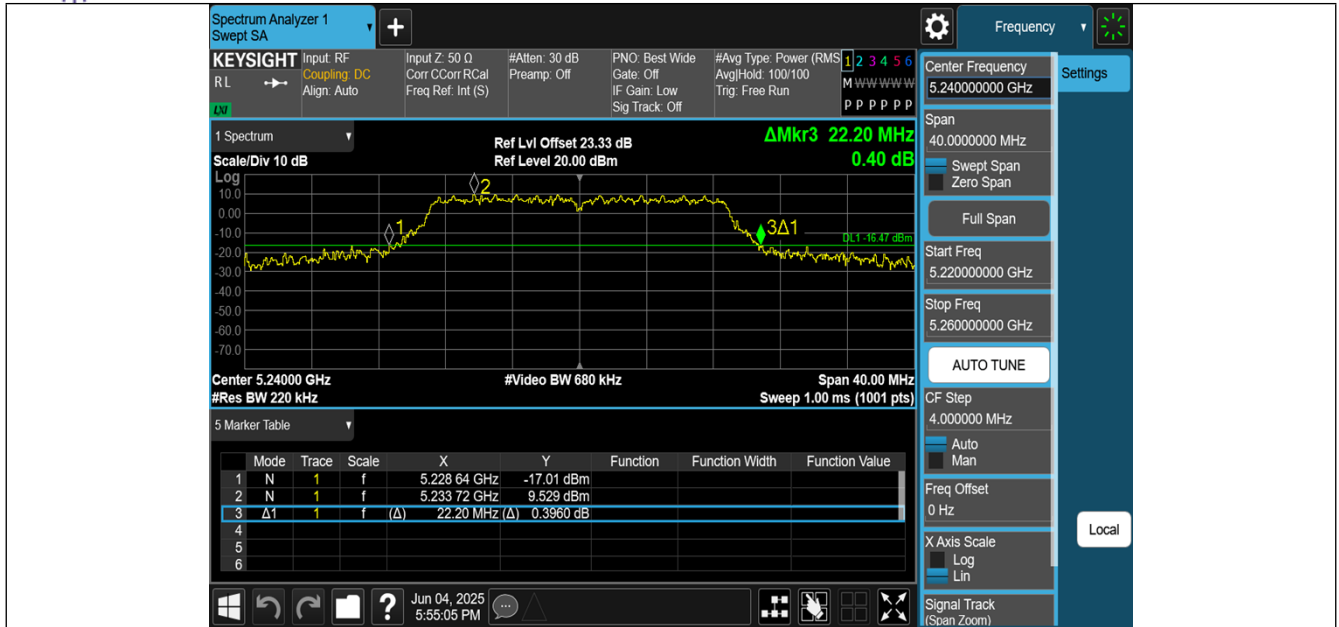
11N20MIMO-Ant0-5240
