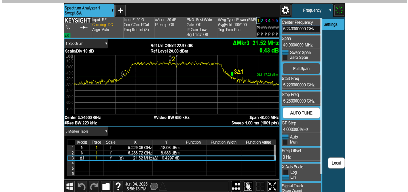
11N20MIMO-Ant1-5240
