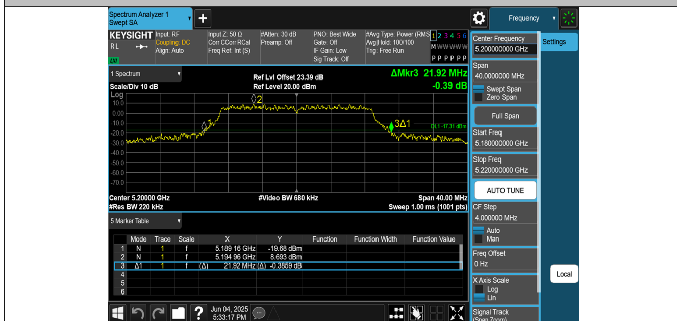
11N20MIMO-Ant3-5200
