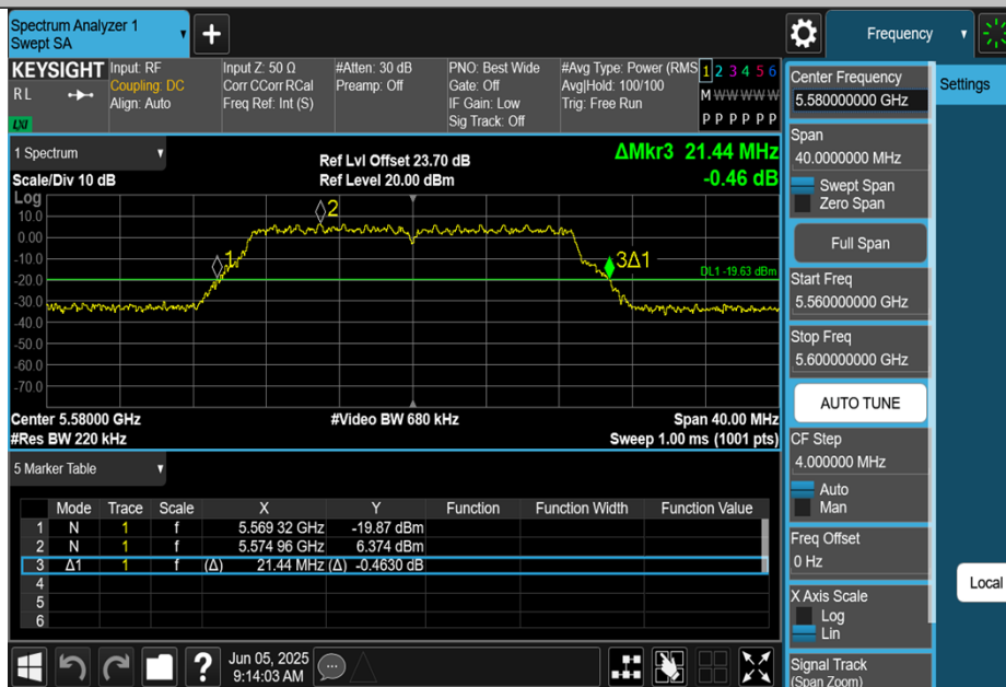
11N20MIMO-Ant3-5580
