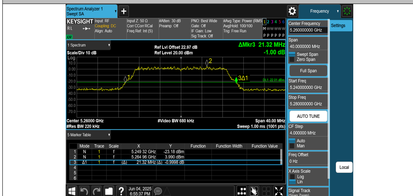
11N20MIMO-Ant1-5260
