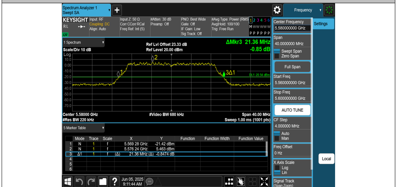
11N20MIMO-Ant1-5580
