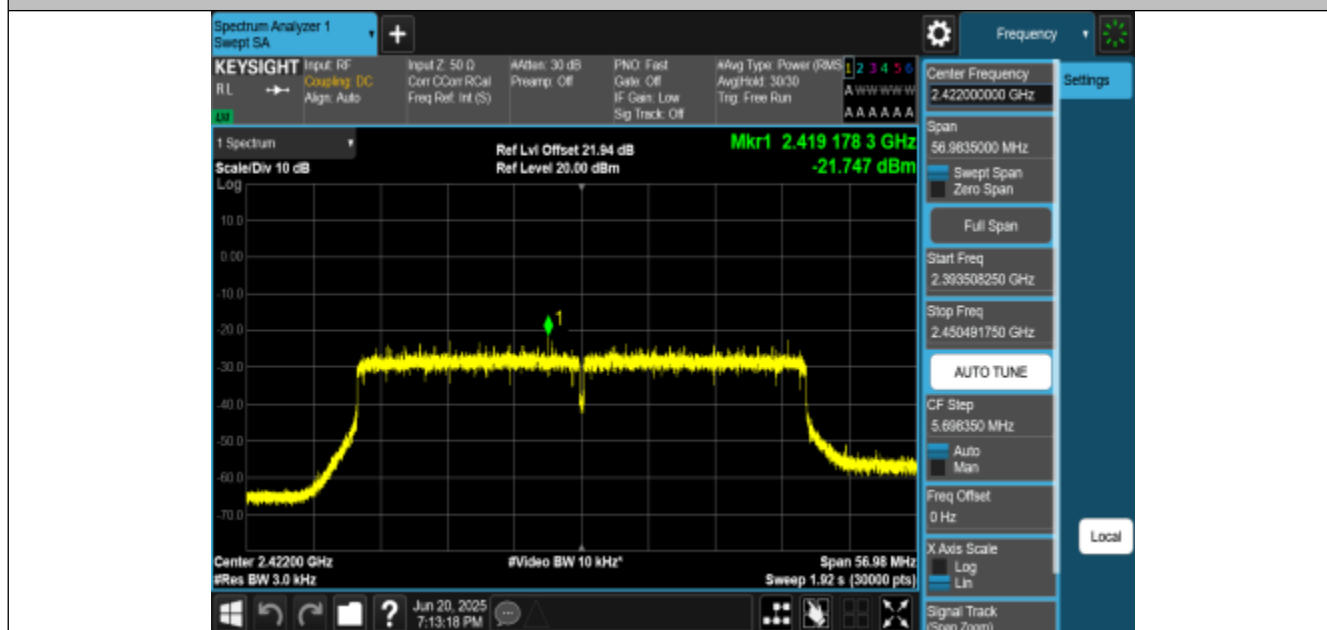
11AX40MIMO-Ant0-2422-PASS
