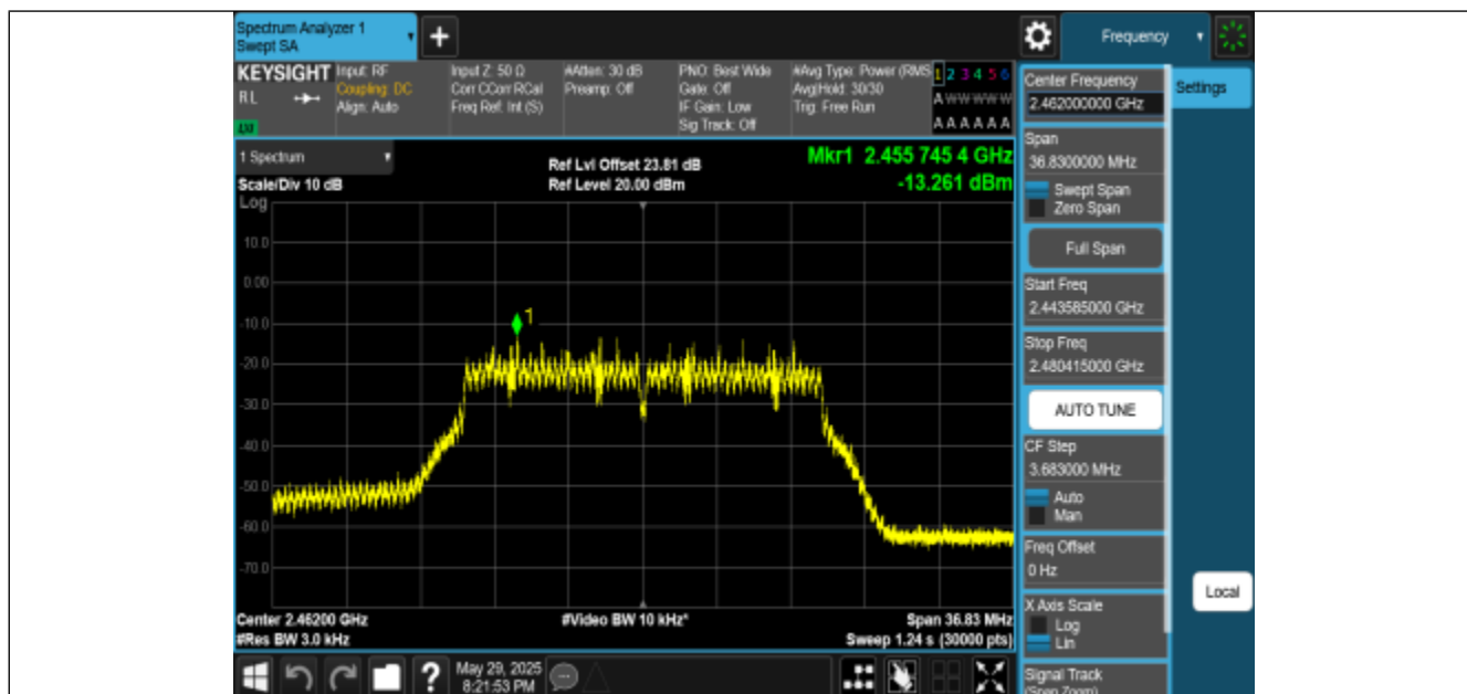
11N20MIMO-Ant0-2462-PASS
