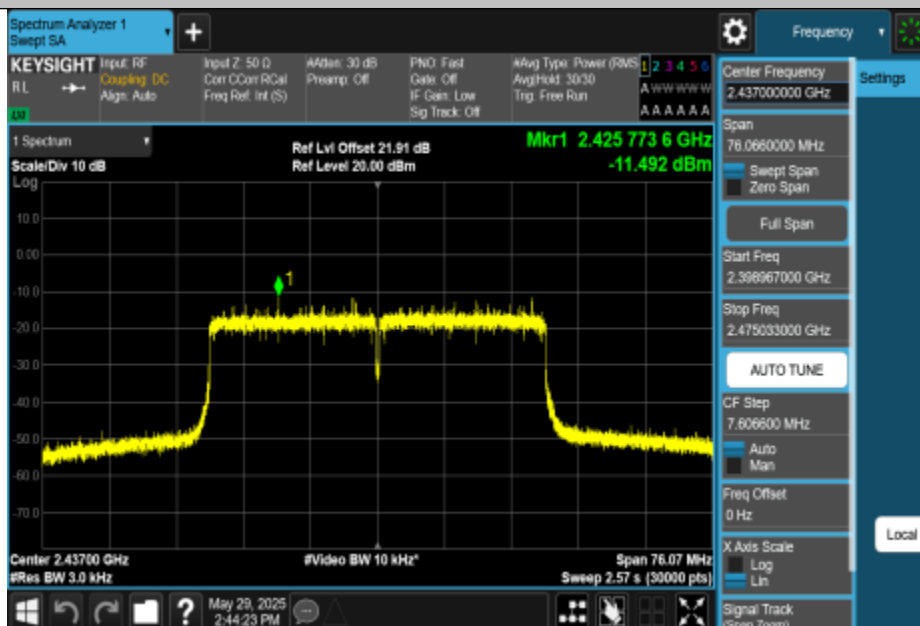
11AX40MIMO-Ant1-2437-PASS
