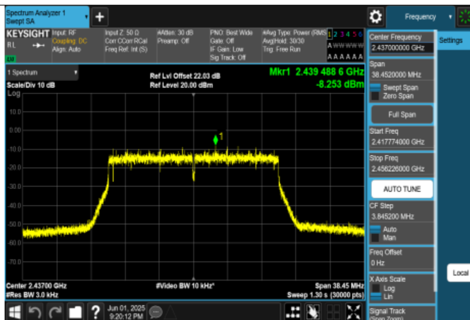
11BE20MIMO-Ant0-2437-PASS
