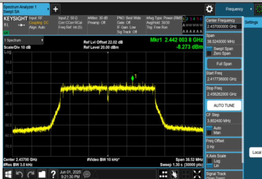
11BE20MIMO-Ant1-2437-PASS
