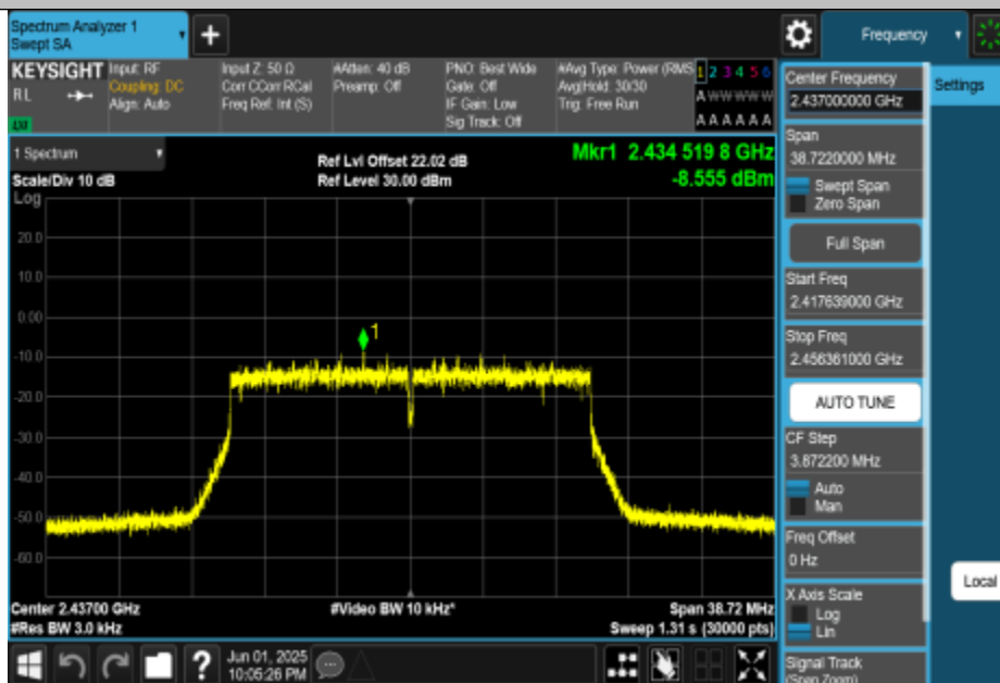
11AX20MIMO-Ant1-2437-PASS
