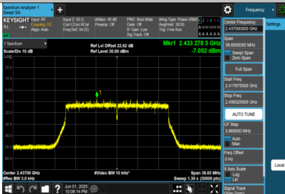
11AX20MIMO-Ant3-2437-PASS
