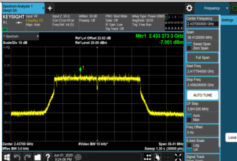
11BE20MIMO-Ant3-2437-PASS
