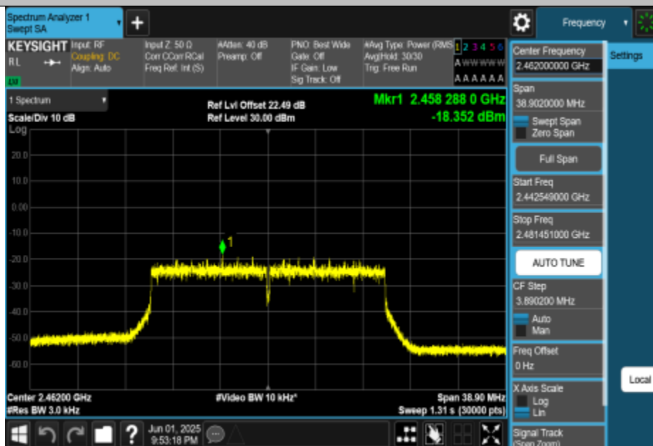
11AX20MIMO-Ant3-2462-PASS
