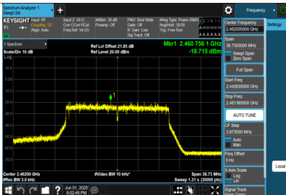
11BE20MIMO-Ant0-2462-PASS
