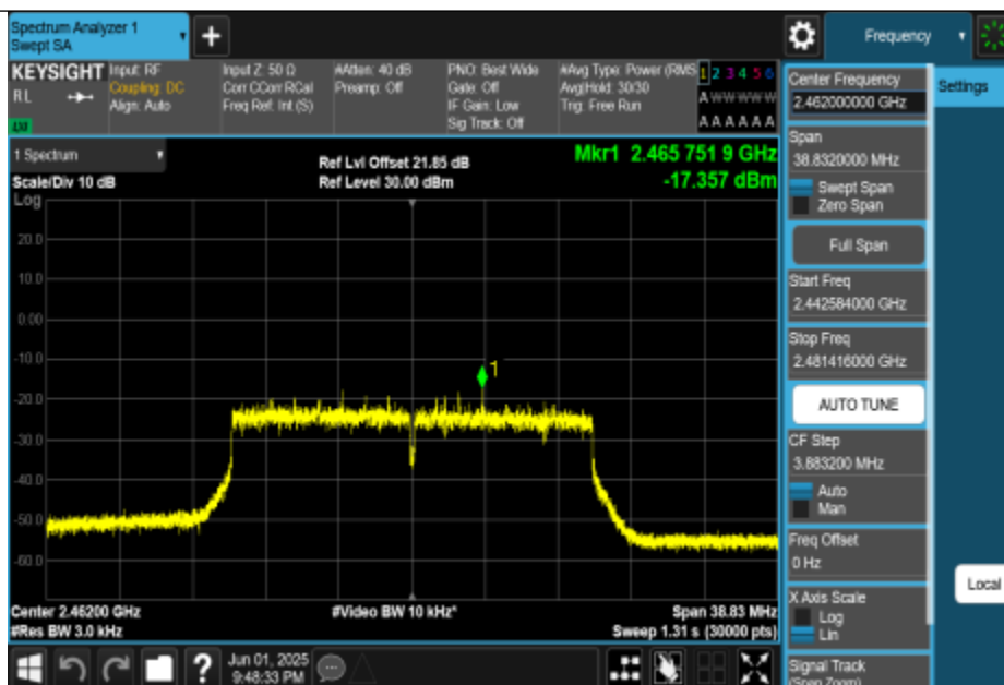
11AX20MIMO-Ant0-2462-PASS
