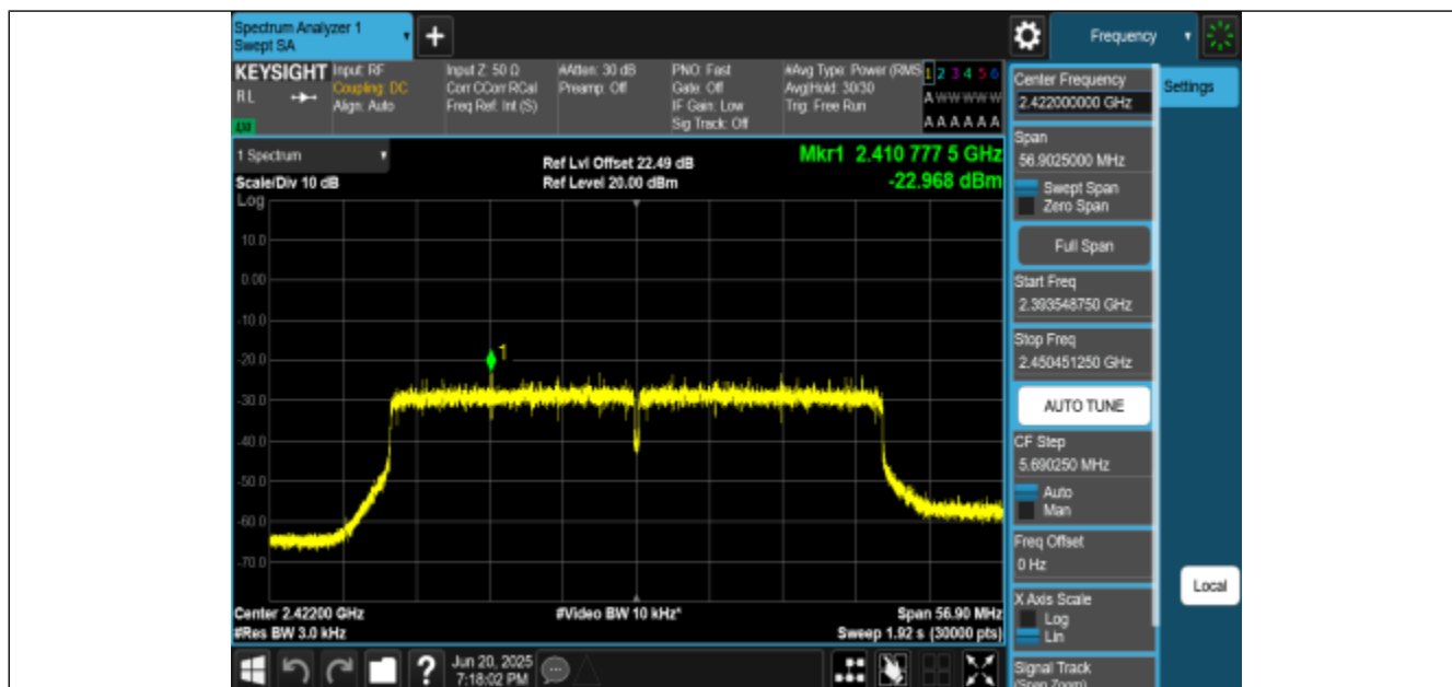
11AX40MIMO-Ant3-2422-PASS
