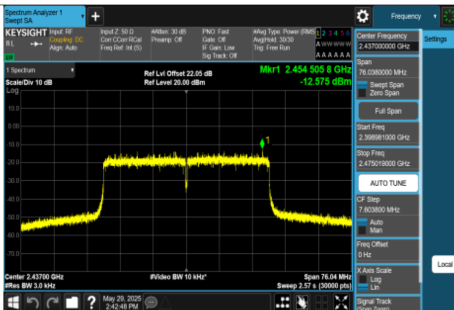
11AX40MIMO-Ant0-2437-PASS
