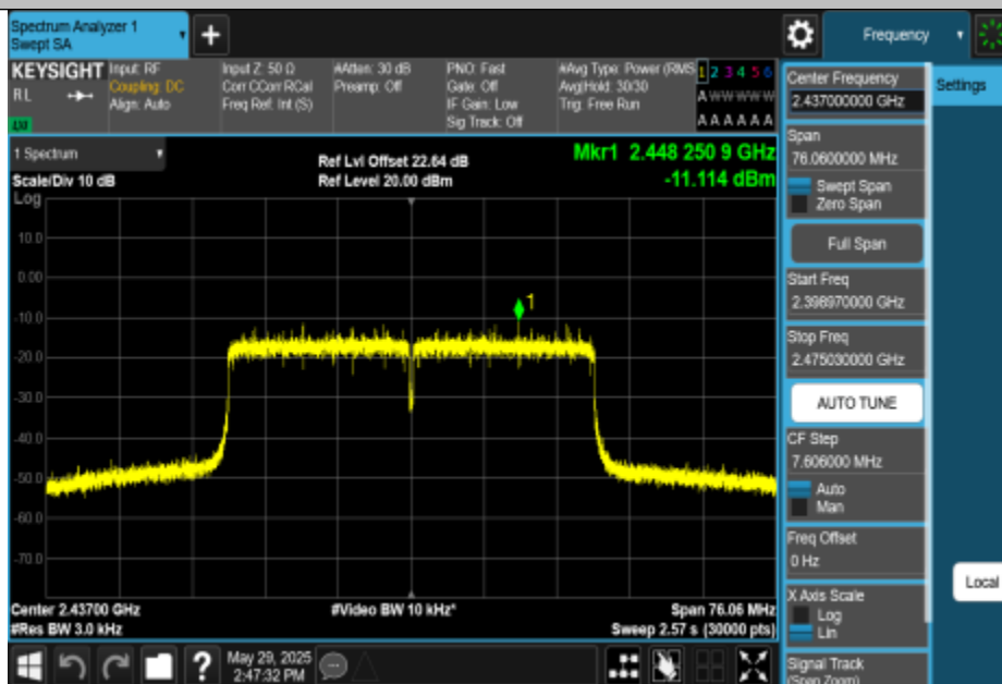
11AX40MIMO-Ant3-2437-PASS
