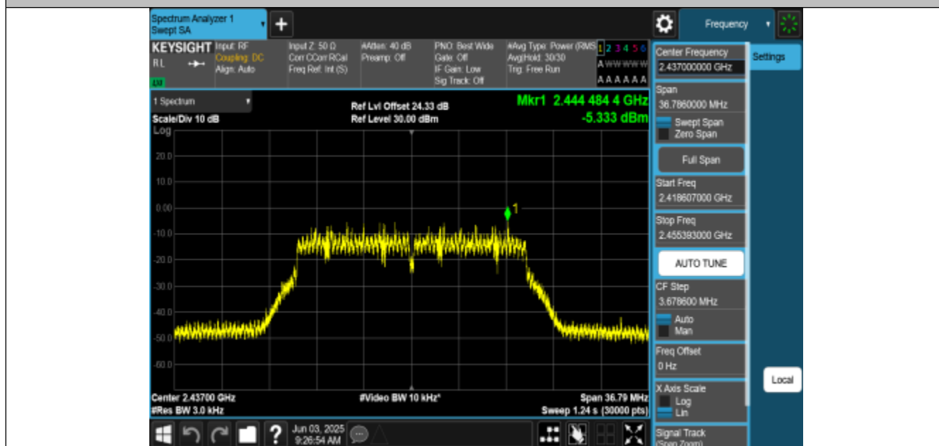
11N20MIMO-Ant3-2437-PASS
