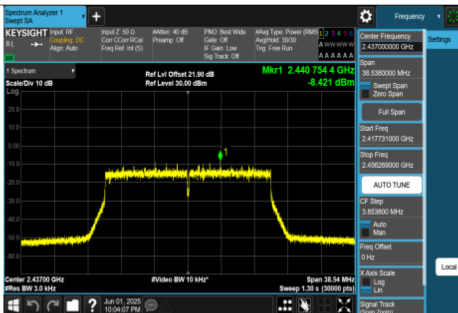
11AX20MIMO-Ant0-2437-PASS
