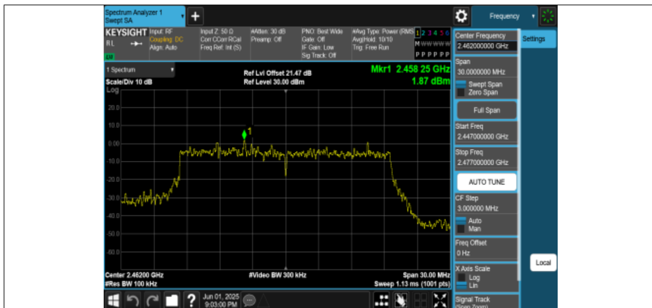
11BE20MIMO-Ant0-2462-0~Reference-PASS
