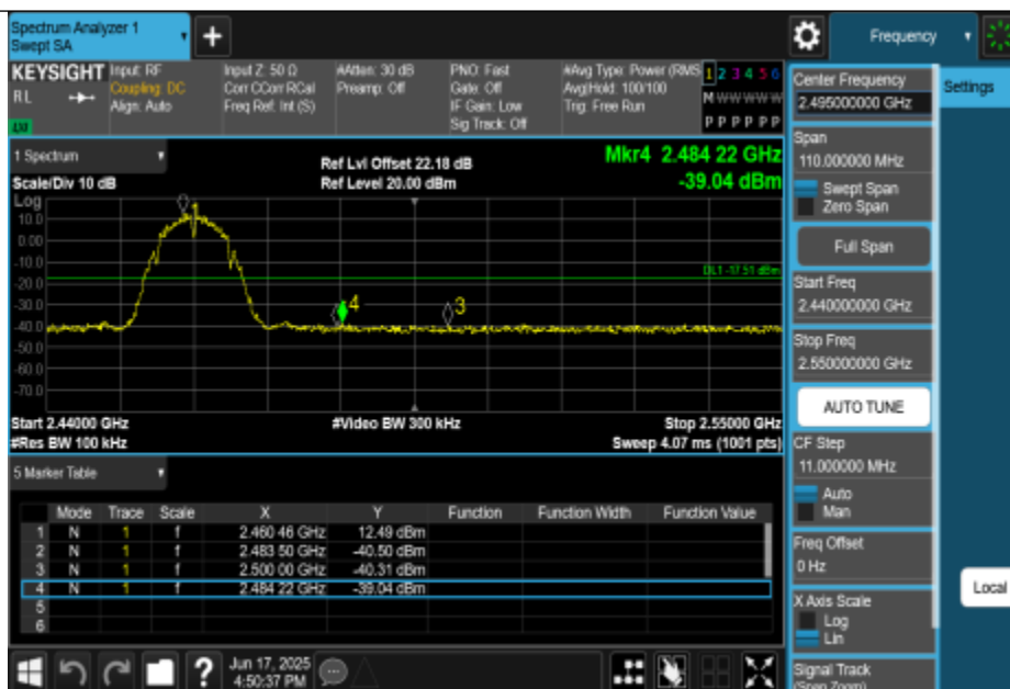
11B-CDD-Ant2-2462-PASS
