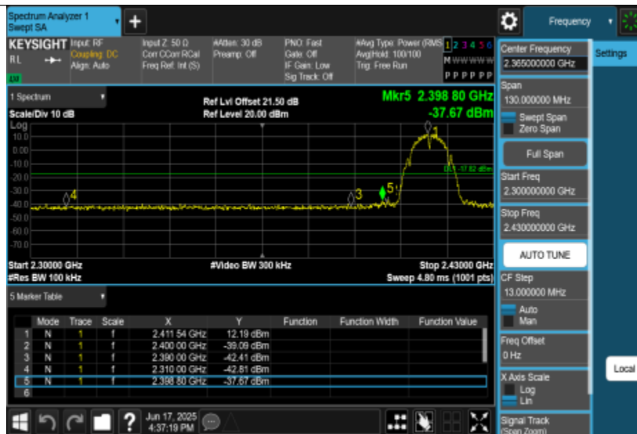
11B-CDD-Ant0-2412-PASS
