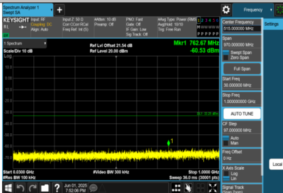
11AX40MIMO-Ant0-2422-30~1000-PASS
