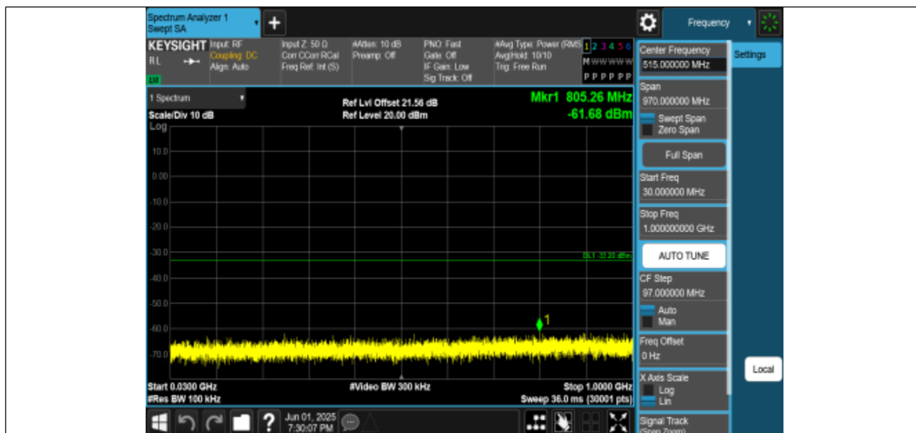
11AX40MIMO-Ant0-2452-30~1000-PASS
