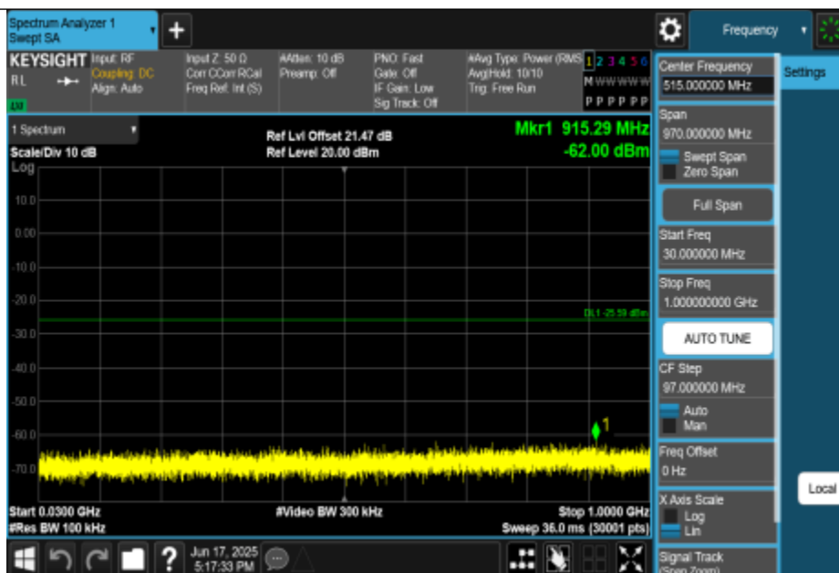
11N20MIMO-Ant0-2462-30~1000-PASS
