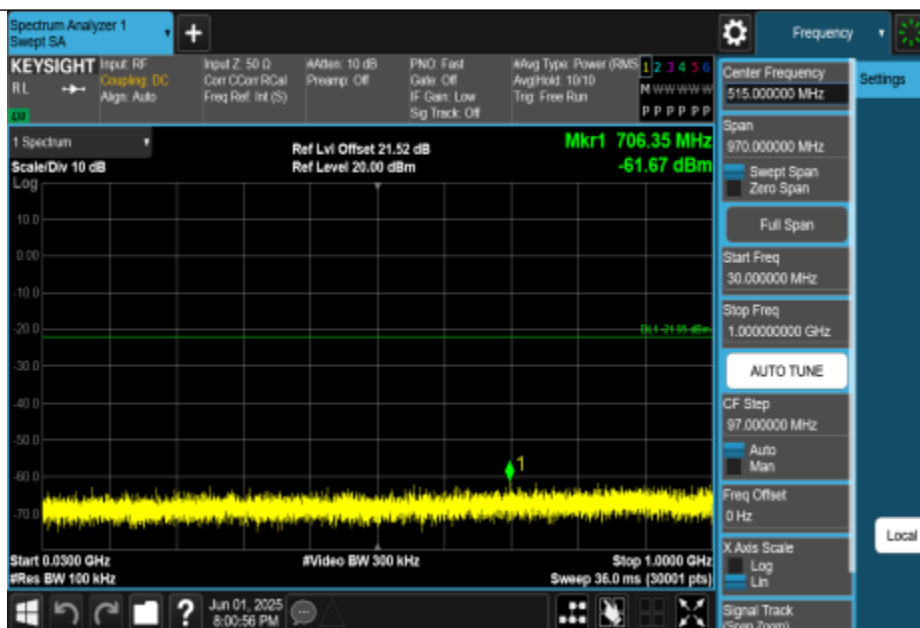
11AX40MIMO-Ant0-2437-30~1000-PASS
