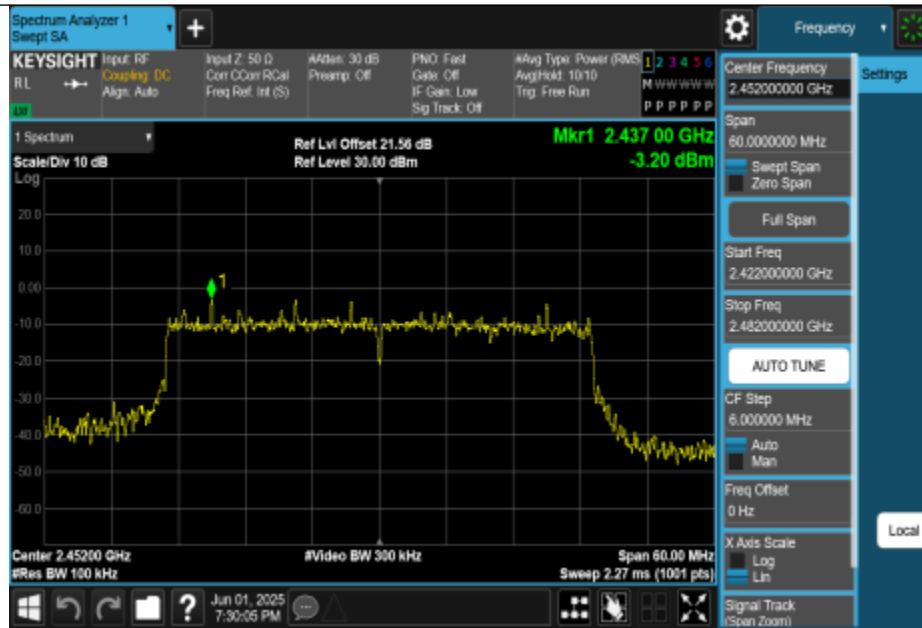
11AX40MIMO-Ant0-2452-0~Reference-PASS
