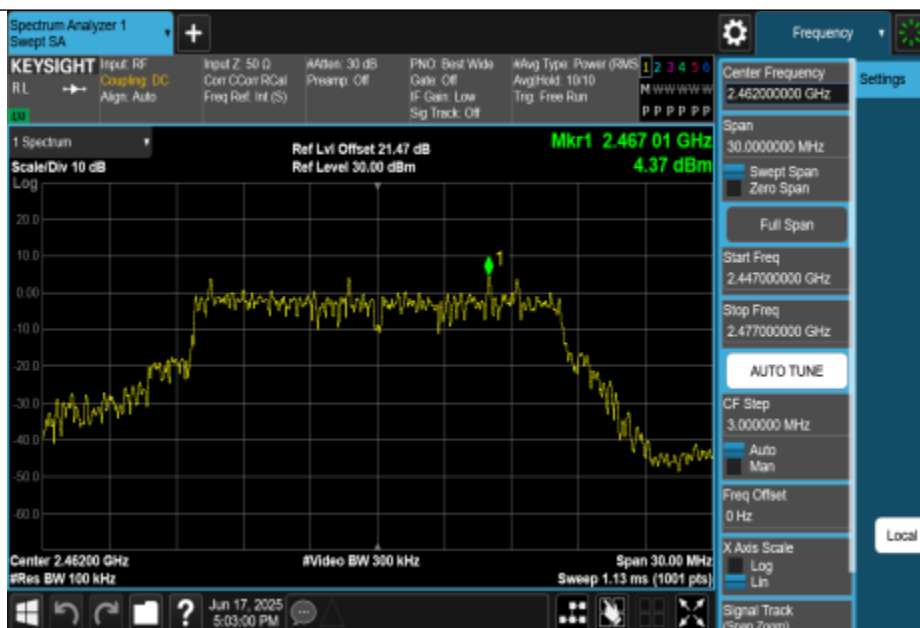
11G-CDD-Ant0-2462-0~Reference-PASS
