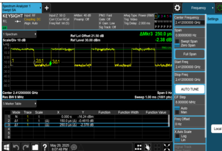
NTNV-11N20MIMO-Ant0-2412
