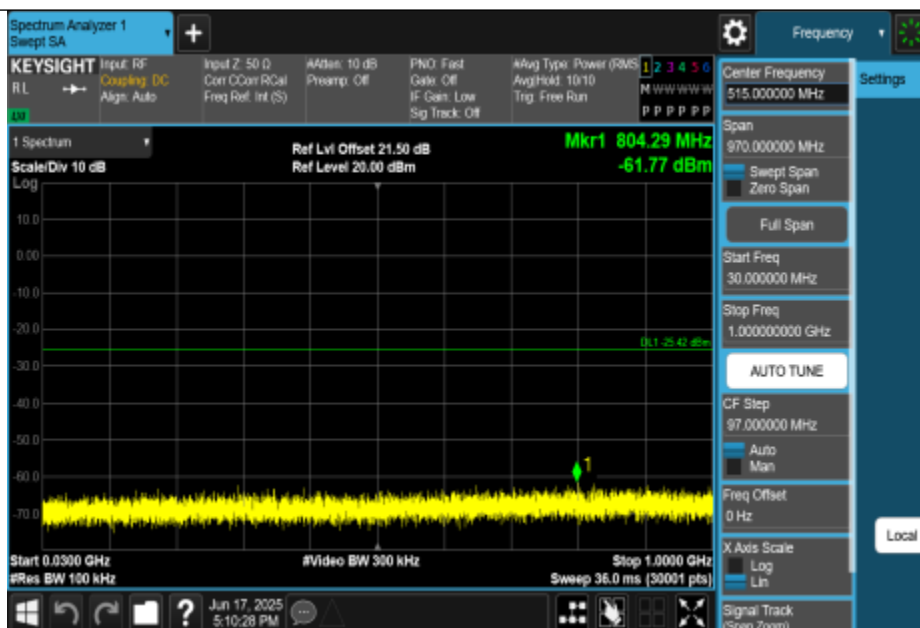
11N20MIMO-Ant0-2412-30~1000-PASS
