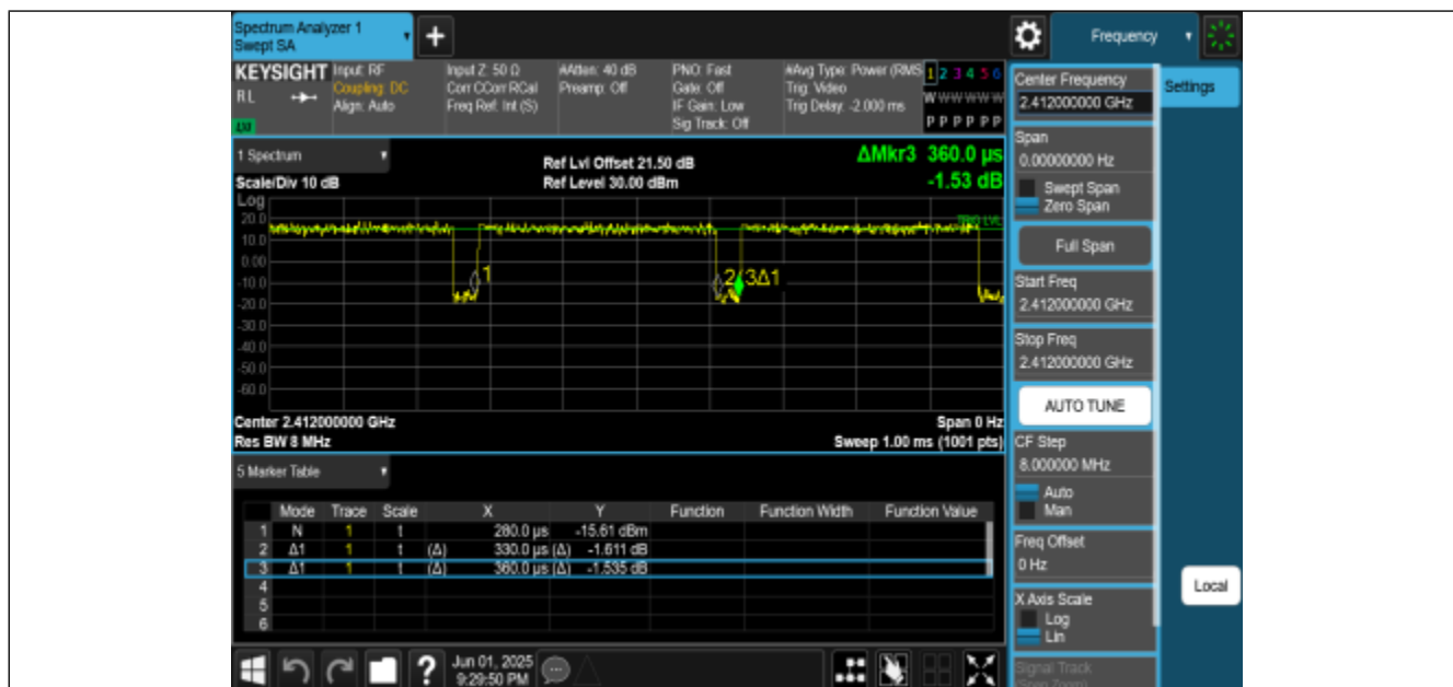
NTNV-11AX20MIMO-Ant0-2412
