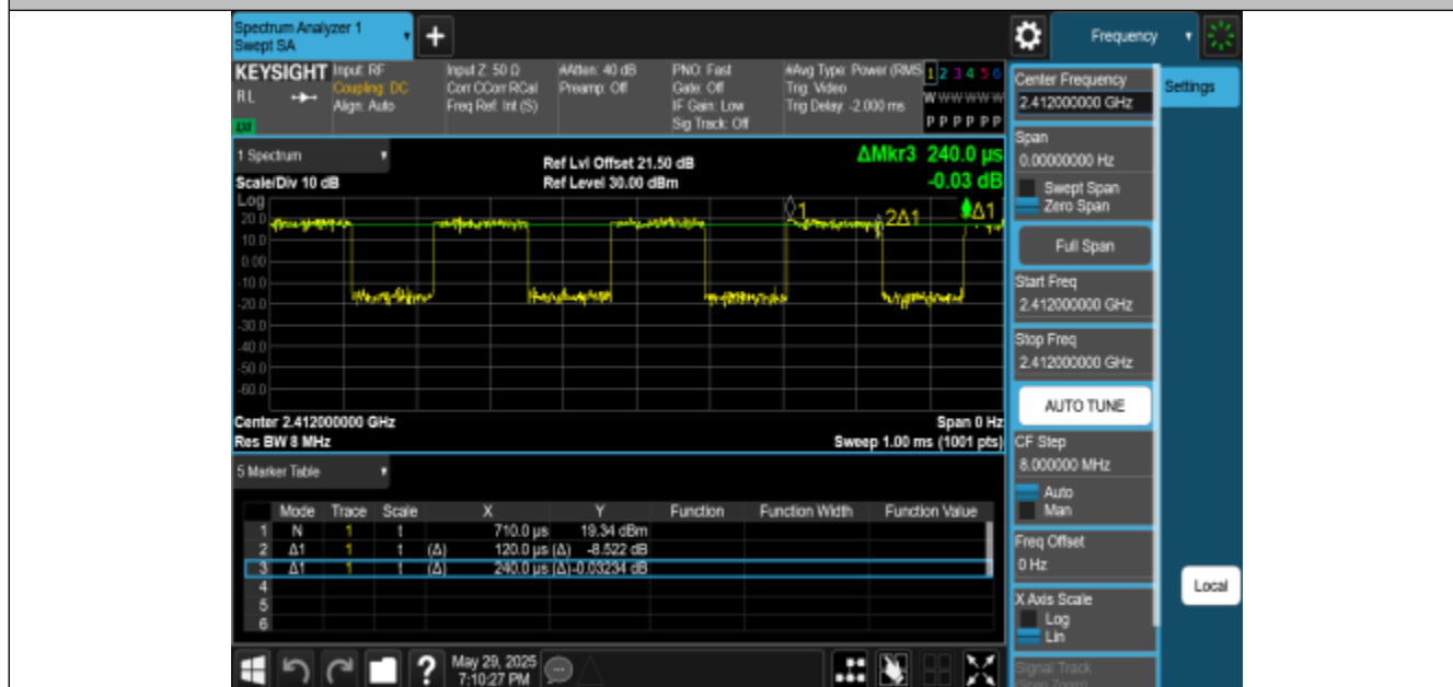
NTNV-11G-CDD-Ant0-2412
