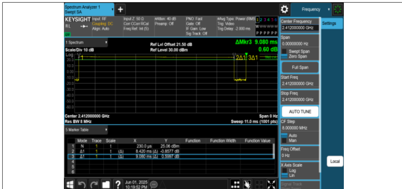
NTNV-11B-CDD-Ant0-2412
