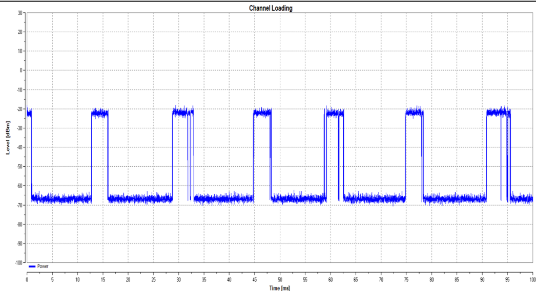
11BE160MIMO_5250
