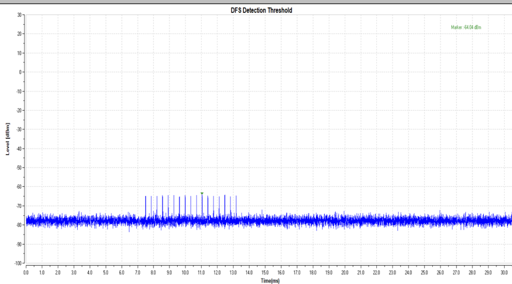
11BE160MIMO_5250_Type4
