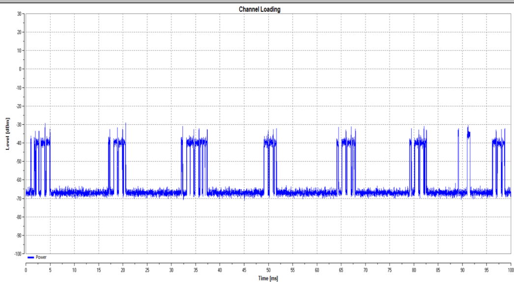
11BE160MIMO_5250
