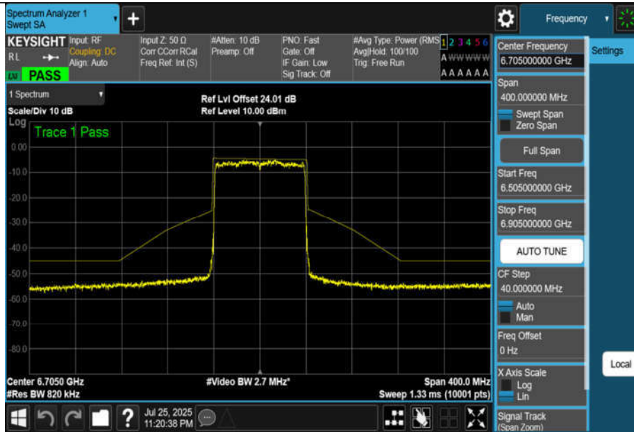
NTNV-11BE80MIMO-Ant1-6705-PASS
