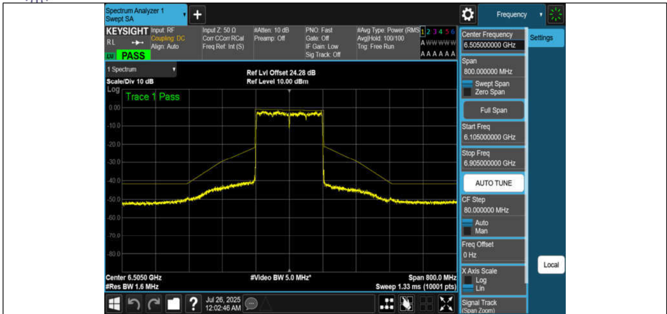
NTNV-11BE160MIMO-Ant1-6505-PASS
