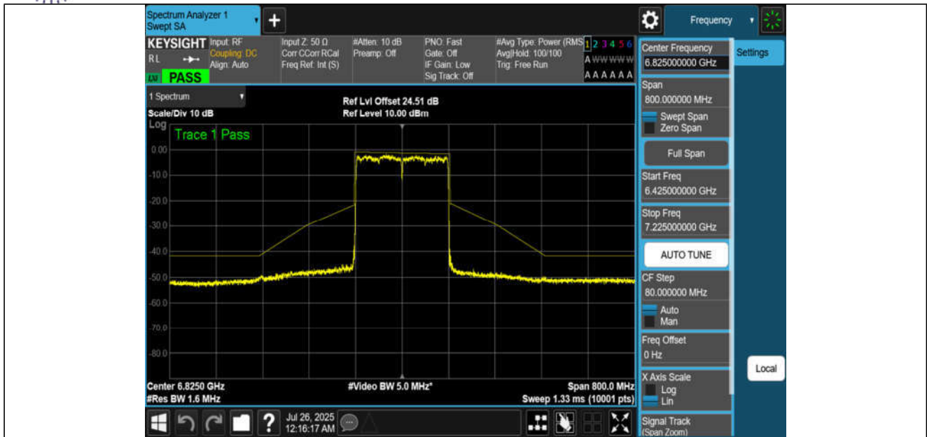
NTNV-11BE160MIMO-Ant1-6825-PASS
