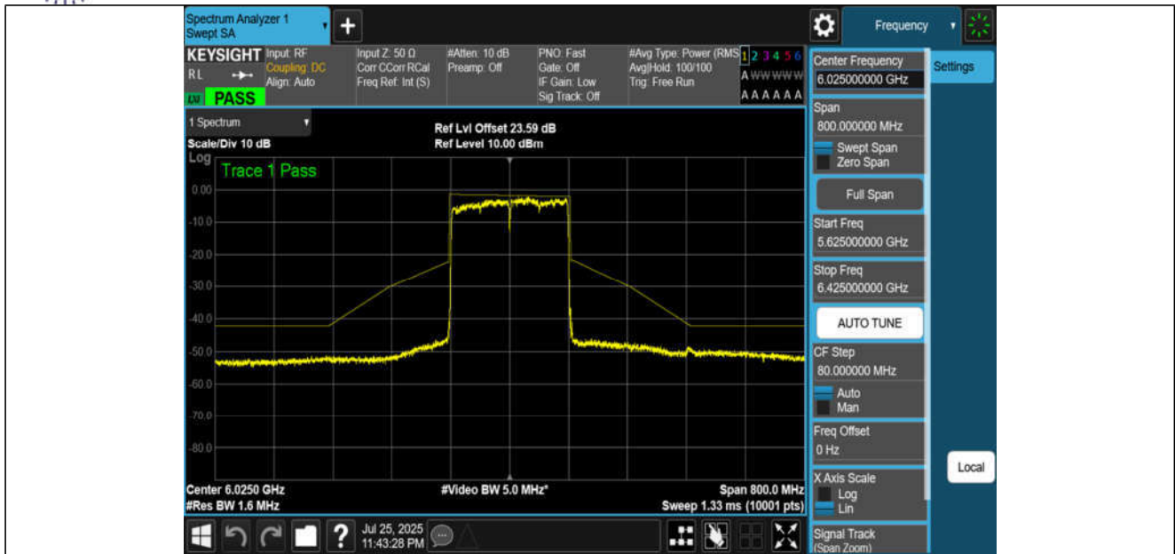
NTNV-11BE160MIMO-Ant1-6025-PASS
