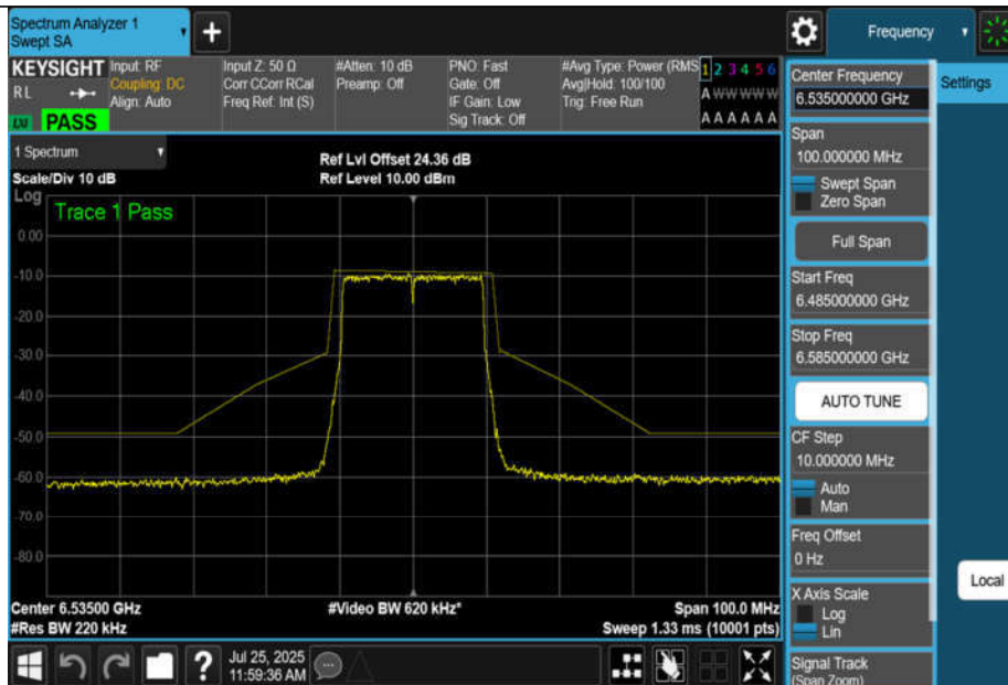
NTNV-11BE20MIMO-Ant1-6535-PASS
