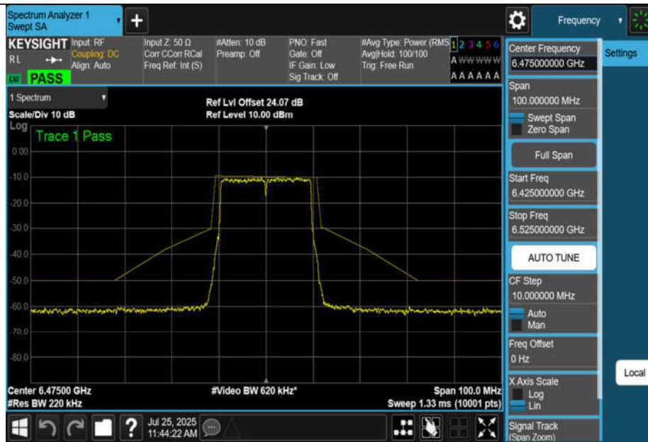
NTNV-11BE20MIMO-Ant1-6475-PASS
