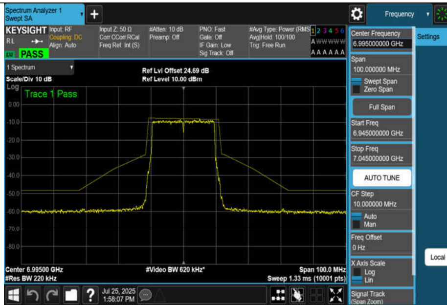
NTNV-11BE20MIMO-Ant1-6995-PASS
