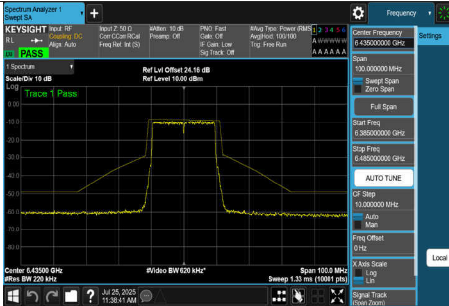
NTNV-11BE20MIMO-Ant1-6435-PASS
