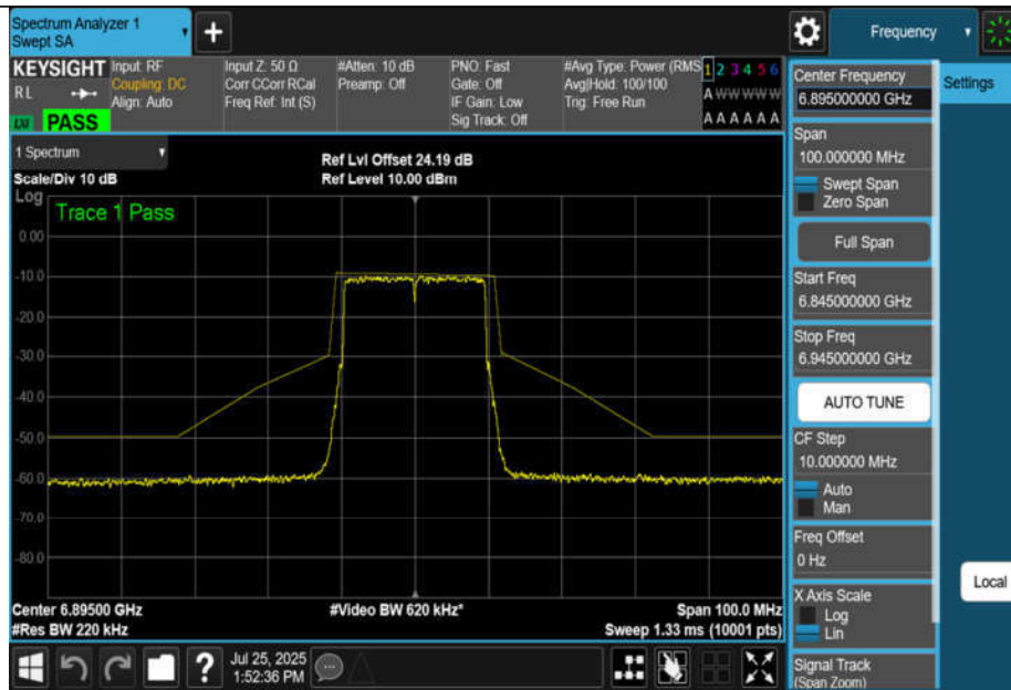
NTNV-11BE20MIMO-Ant1-6895-PASS
