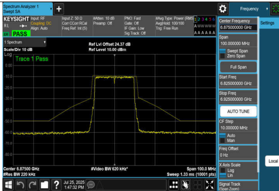
NTNV-11BE20MIMO-Ant1-6875-PASS
