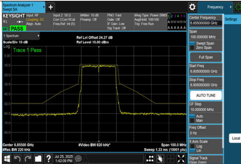
NTNV-11BE20MIMO-Ant1-6855-PASS
