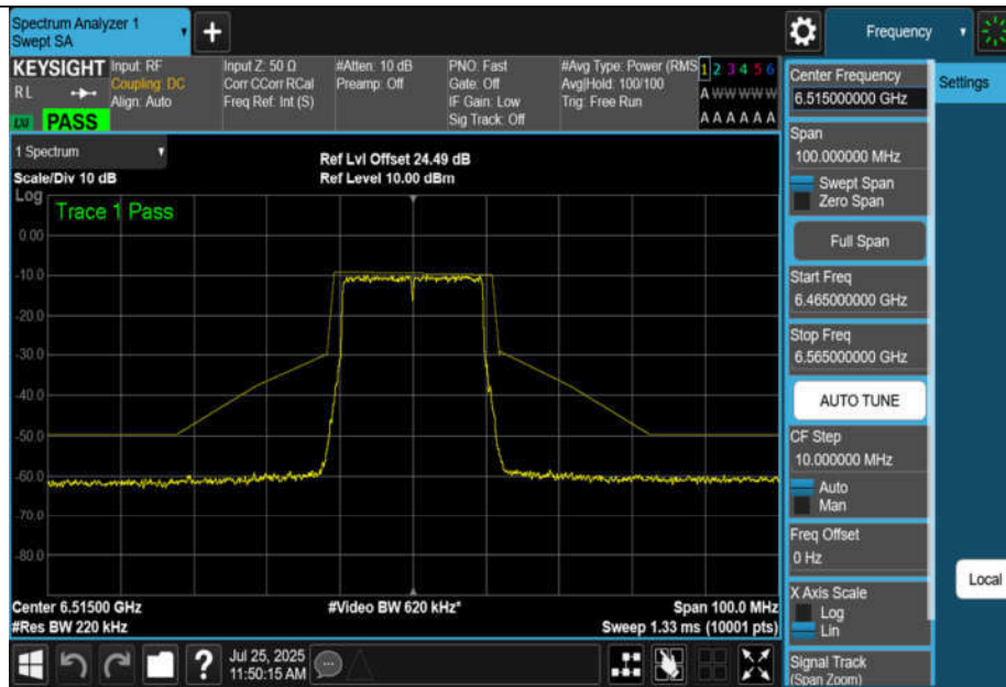
NTNV-11BE20MIMO-Ant1-6515-PASS
