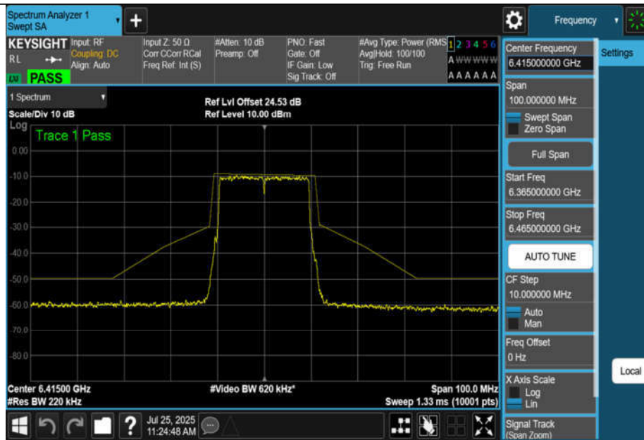
NTNV-11BE20MIMO-Ant1-6415-PASS
