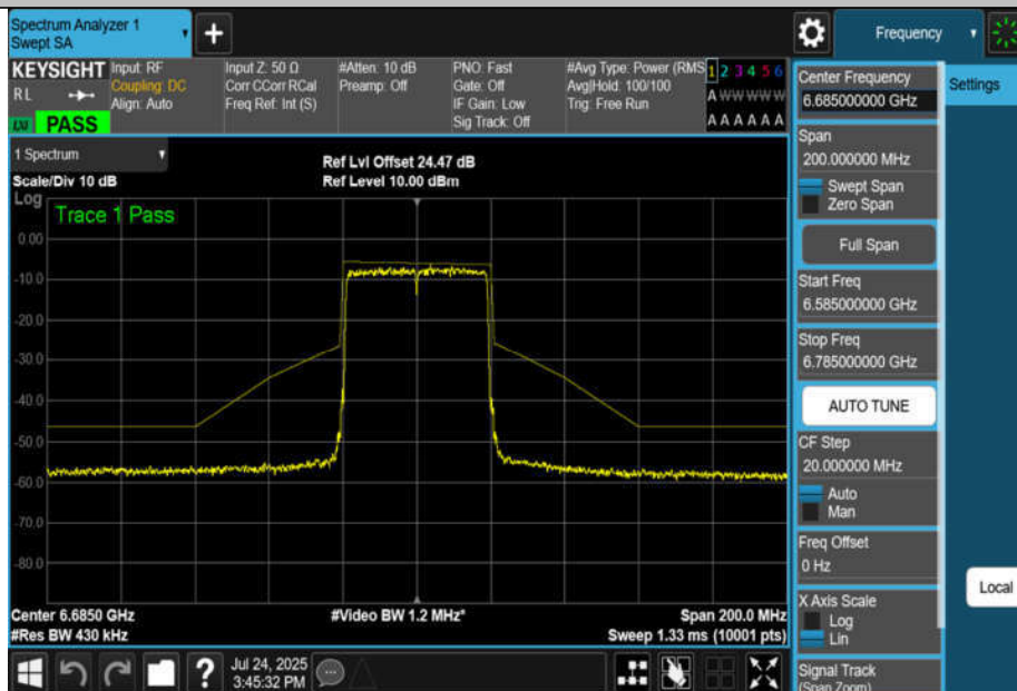
NTNV-11AX40MIMO-Ant4-6685-PASS
