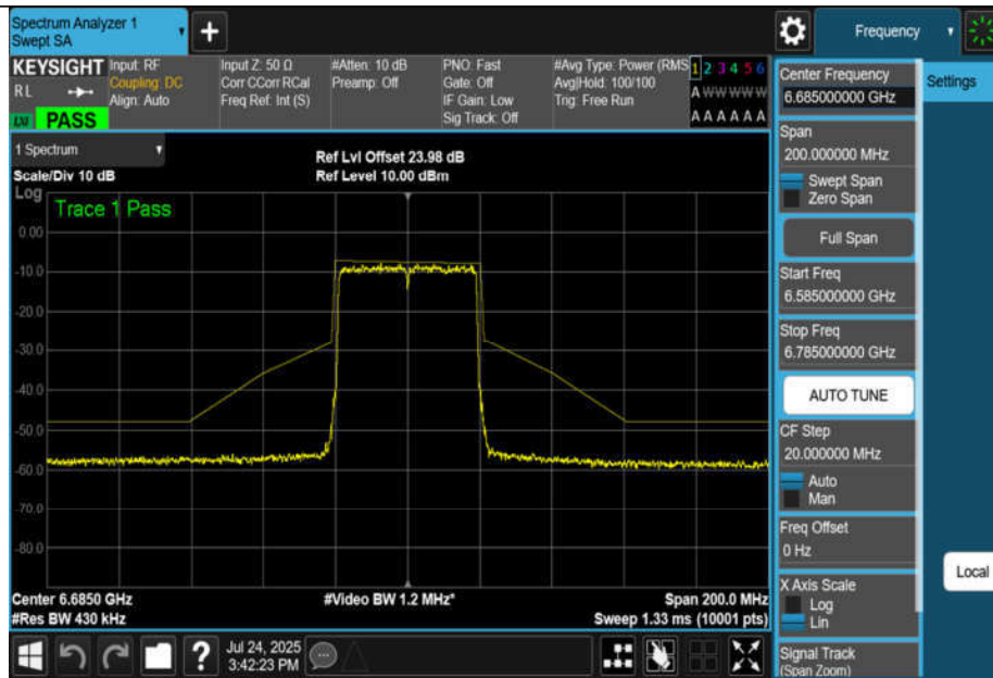
NTNV-11AX40MIMO-Ant1-6685-PASS
