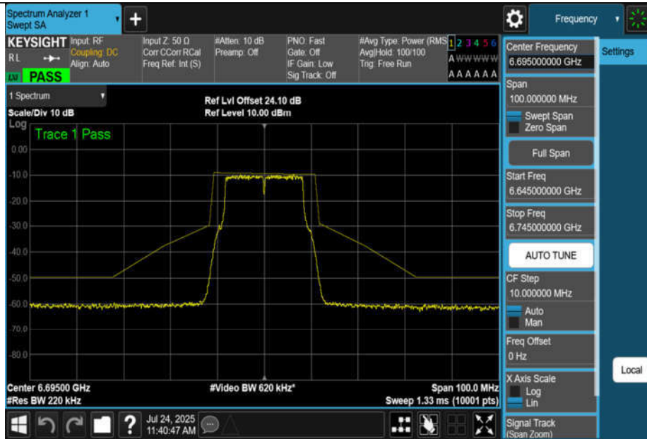
NTNV-11A-CDD-Ant1-6695-PASS
