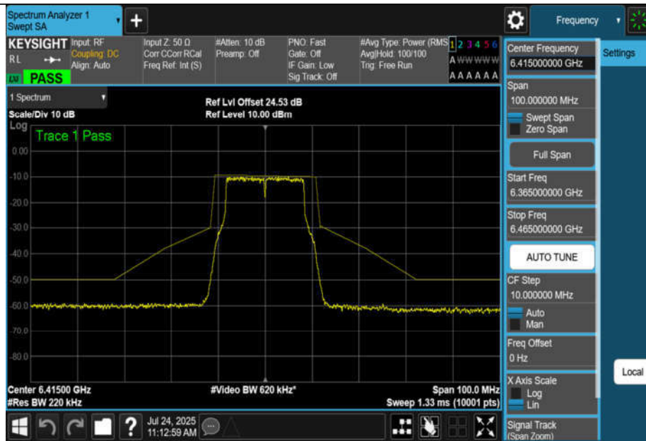
NTNV-11A-CDD-Ant1-6415-PASS
