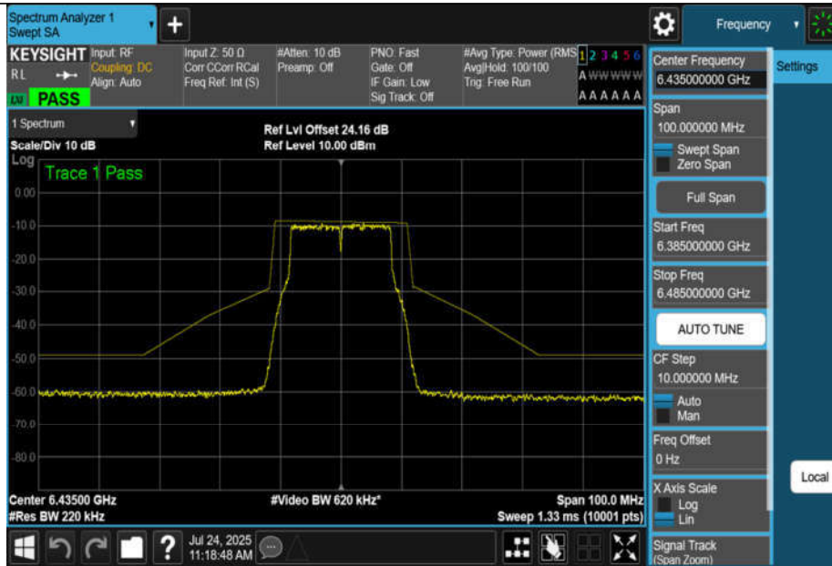
NTNV-11A-CDD-Ant1-6435-PASS
