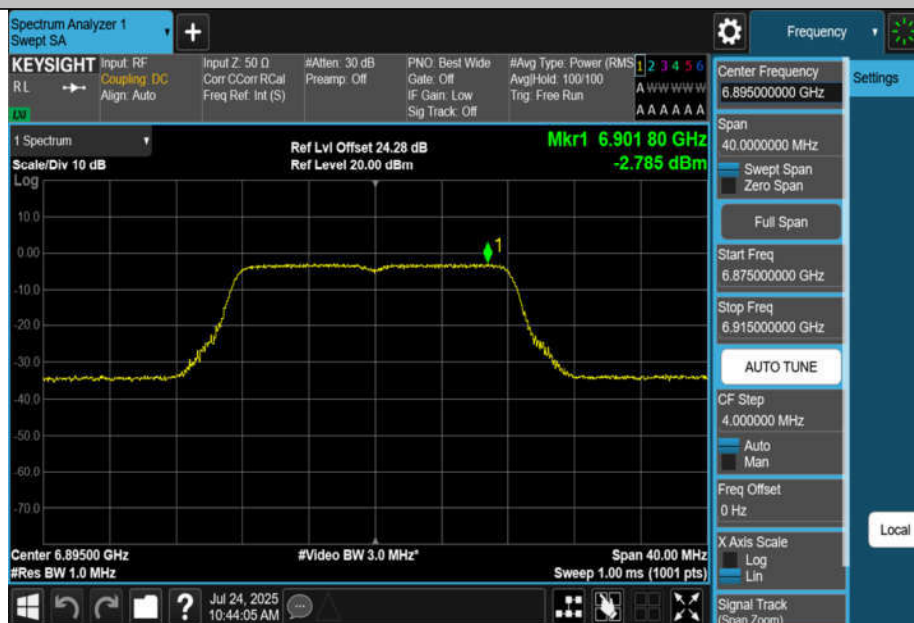
11BE20MIMO-Ant1-6895-PASS
