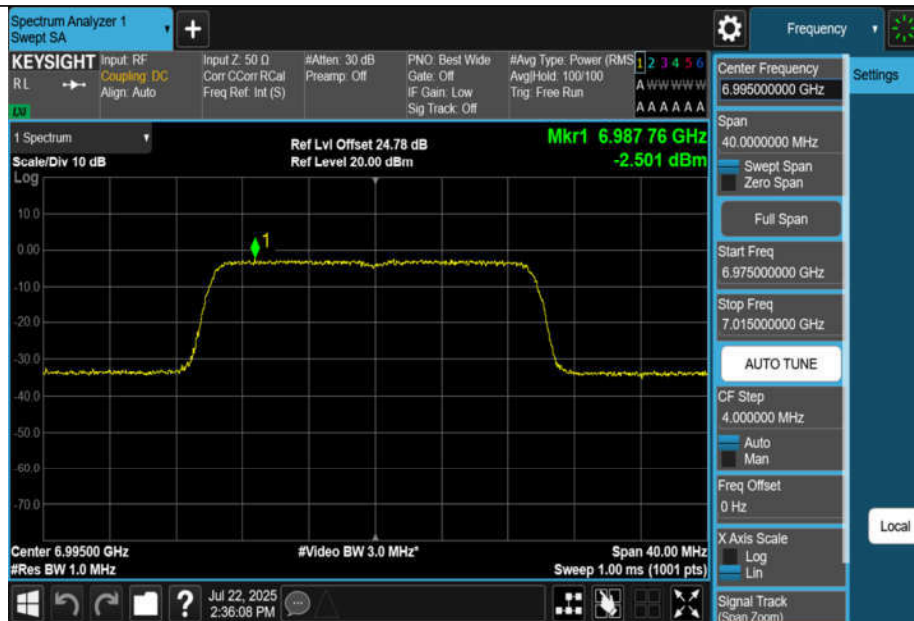
11BE20MIMO-Ant1-6995-PASS
