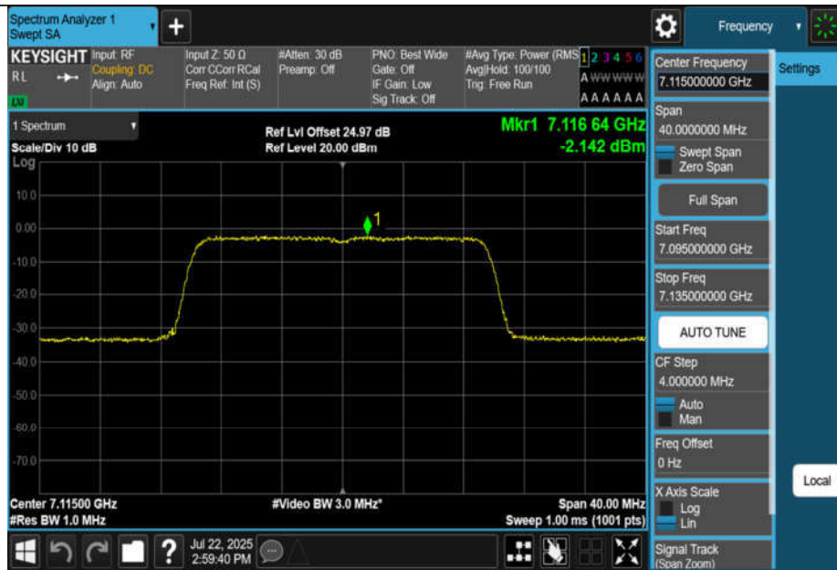
11BE20MIMO-Ant3-7115-PASS
