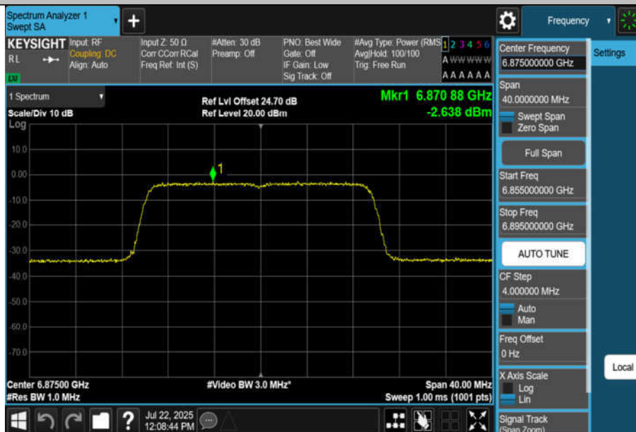
11BE20MIMO-Ant4-6875-PASS
