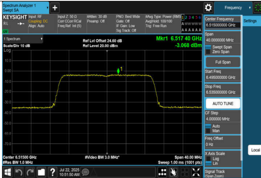
11BE20MIMO-Ant1-6515-PASS
