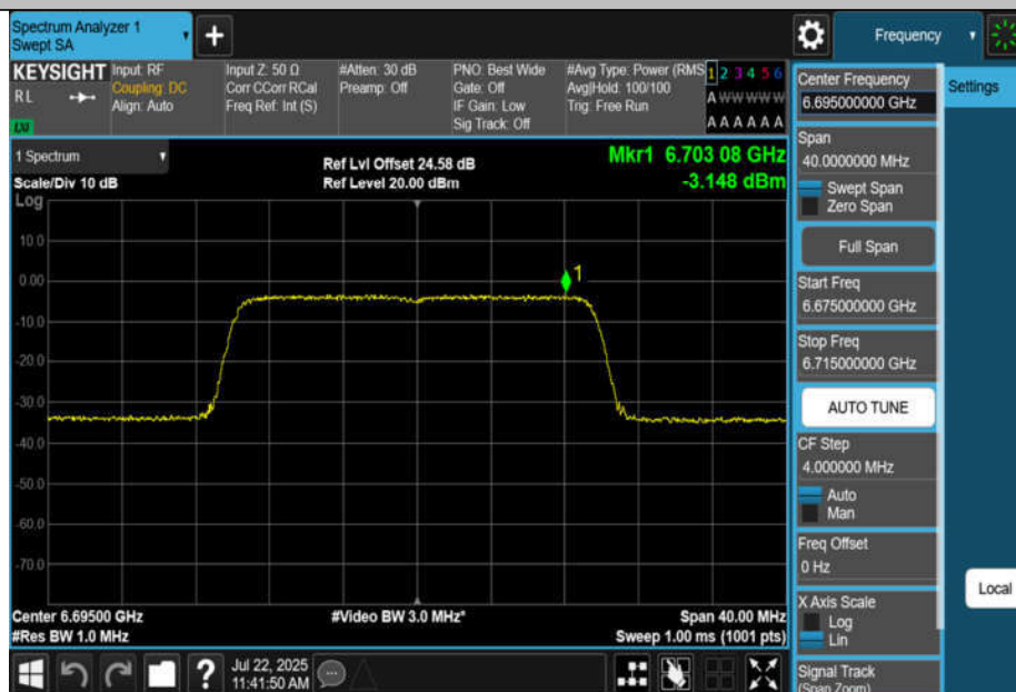
11BE20MIMO-Ant4-6695-PASS
