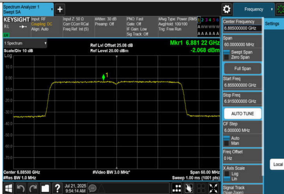
11AX40MIMO-Ant4-6885-PASS
