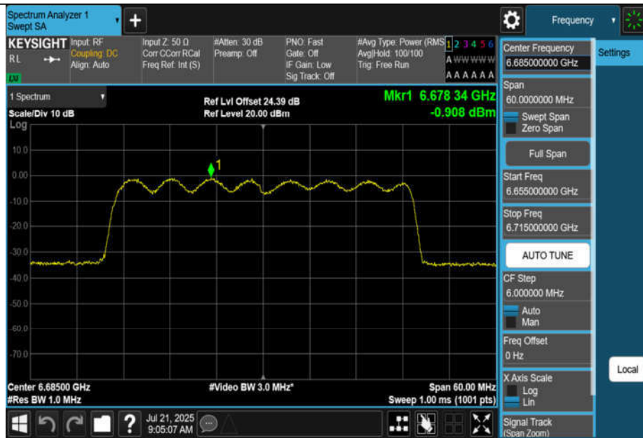
11AX40MIMO-Ant3-6685-PASS
