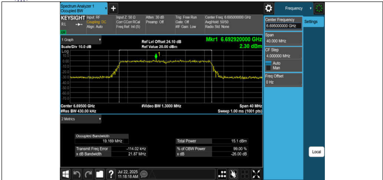
11BE20MIMO-Ant1-6695-PASS
