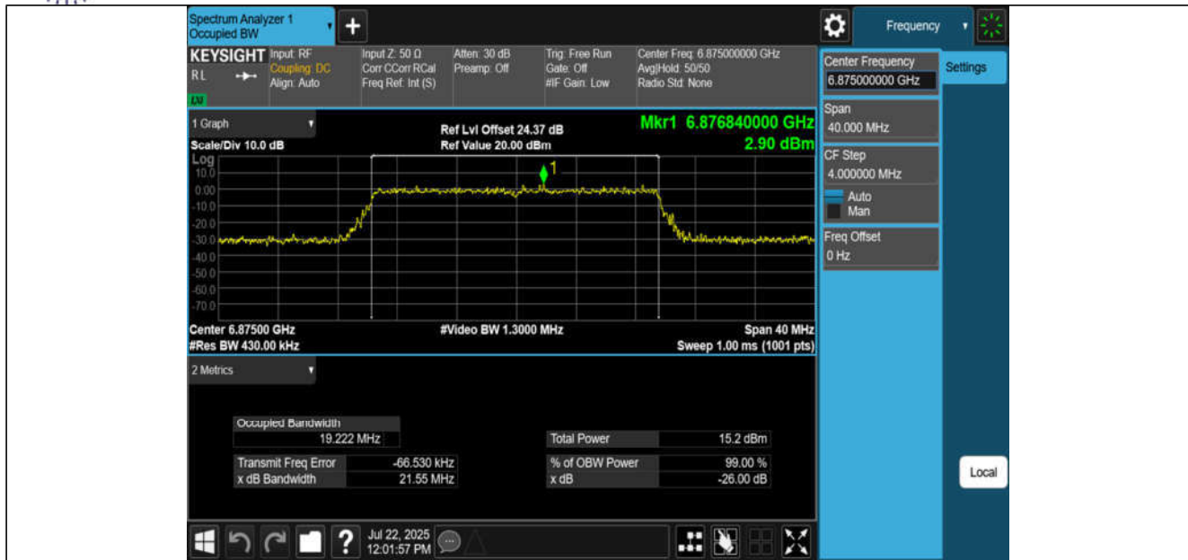
11BE20MIMO-Ant1-6875-PASS
