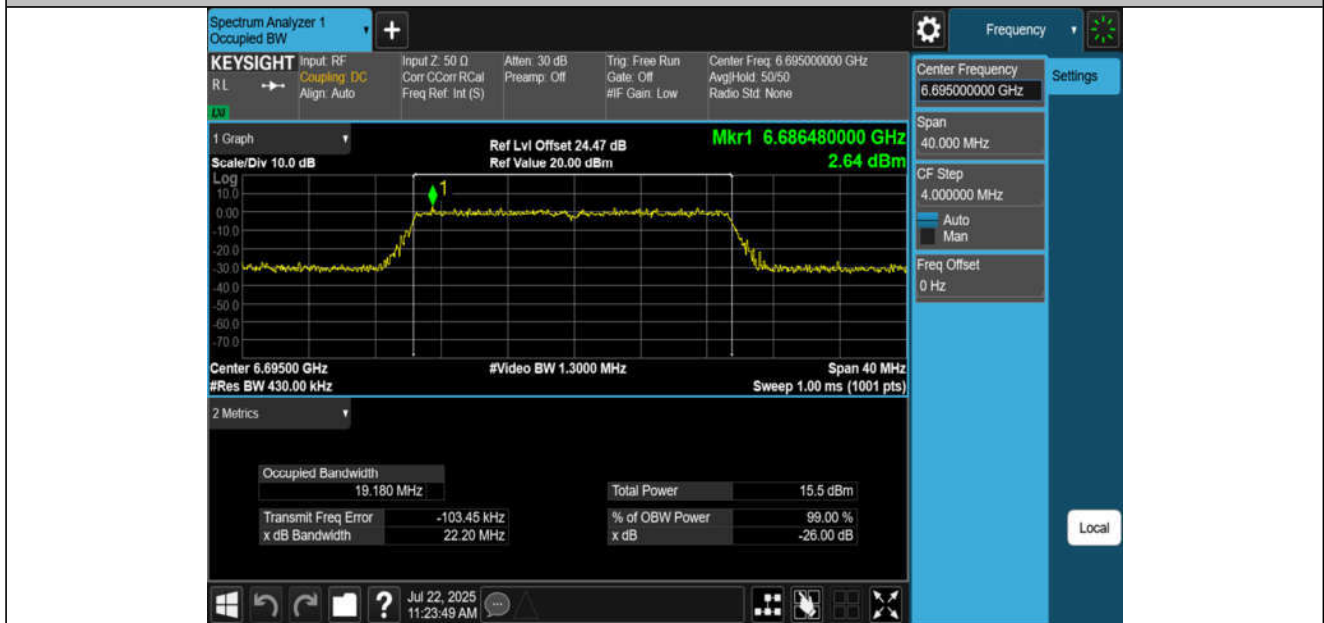
11BE20MIMO-Ant4-6695-PASS
