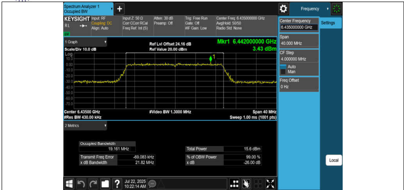
11BE20MIMO-Ant1-6435-PASS
