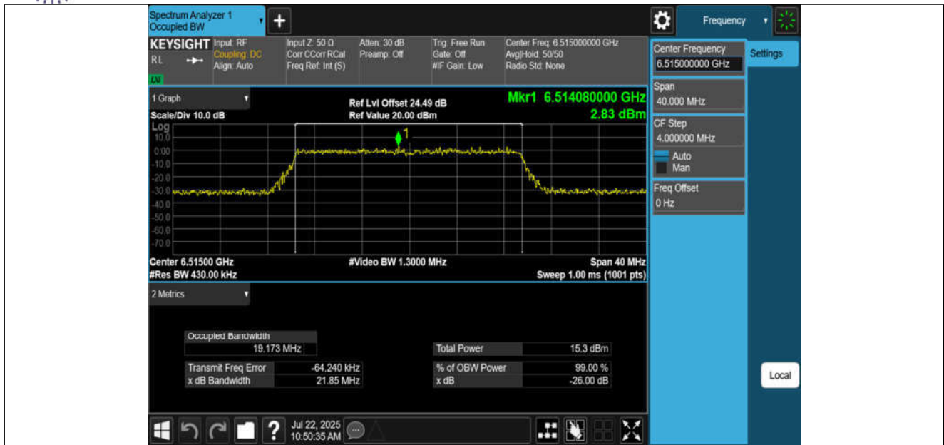
11BE20MIMO-Ant1-6515-PASS
