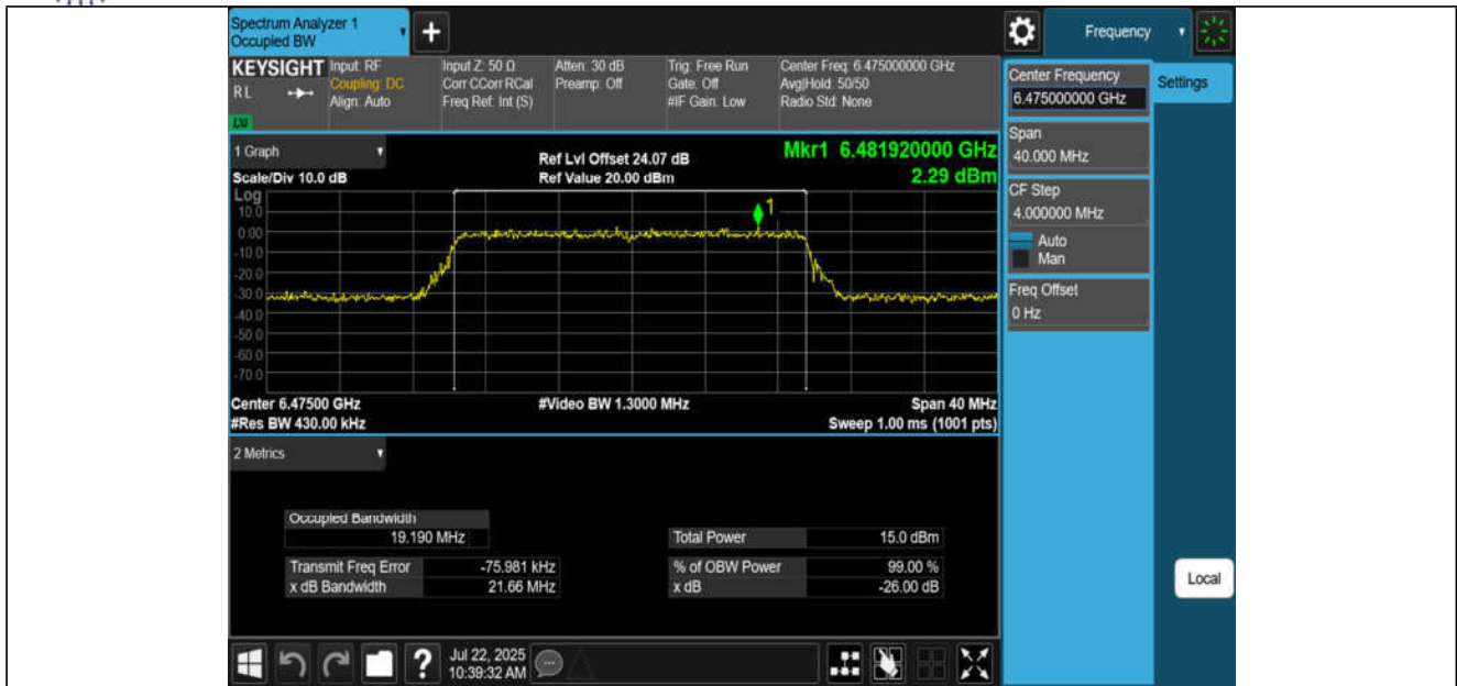
11BE20MIMO-Ant1-6475-PASS
