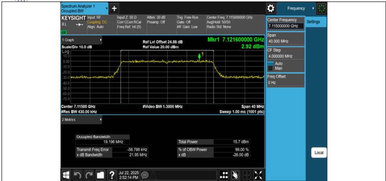
11BE20MIMO-Ant3-7115-PASS
