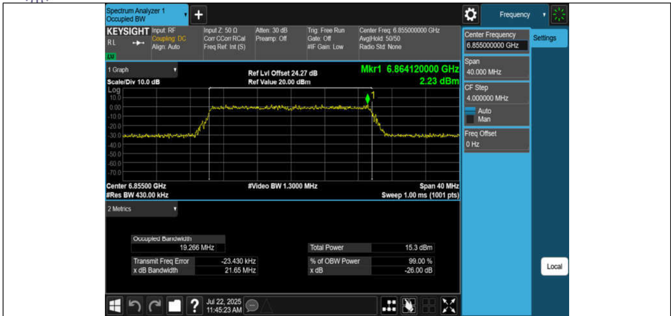
11BE20MIMO-Ant1-6855-PASS
