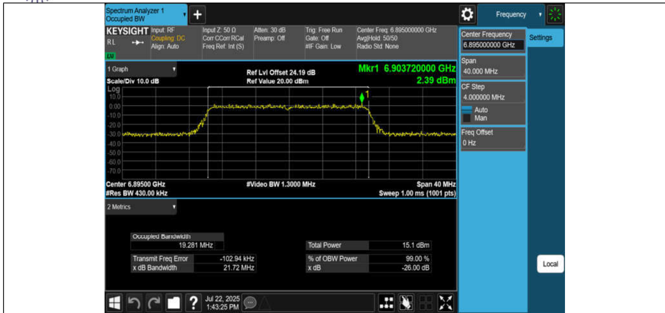
11BE20MIMO-Ant1-6895-PASS
