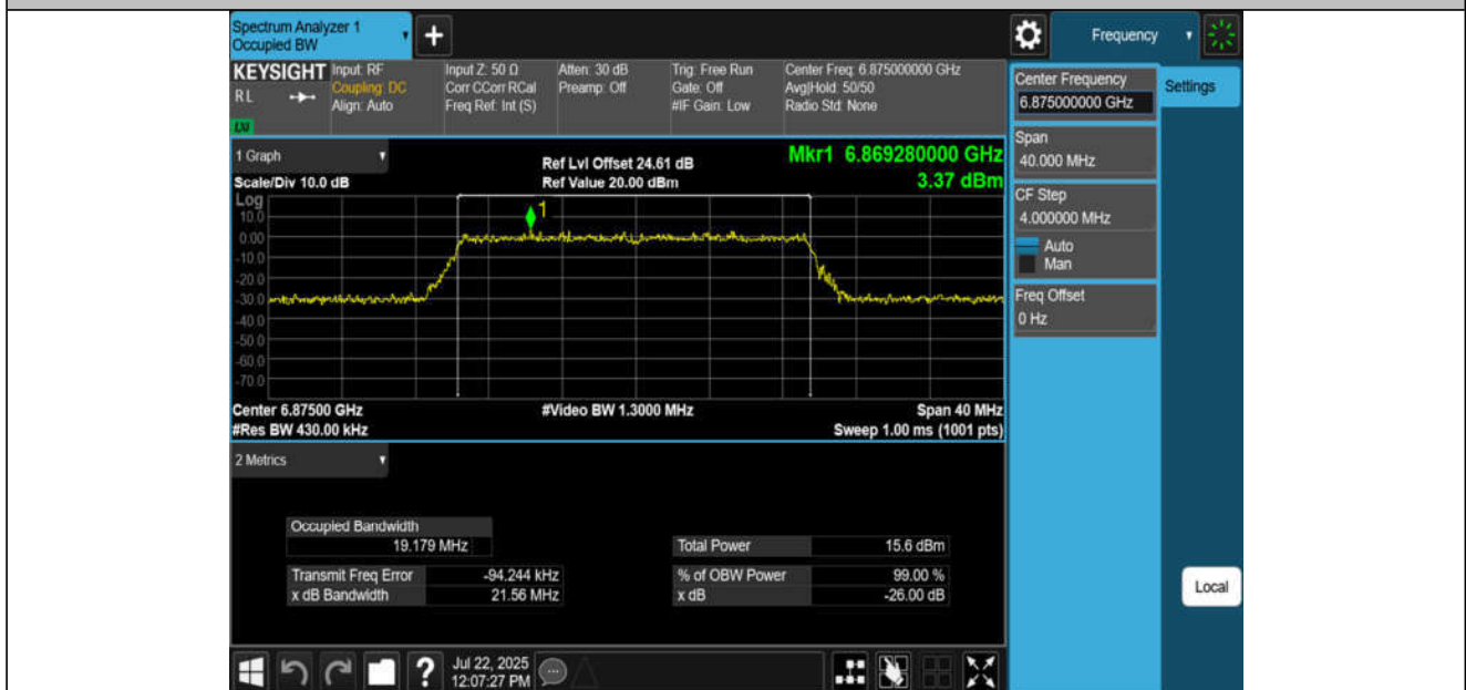
11BE20MIMO-Ant4-6875-PASS
