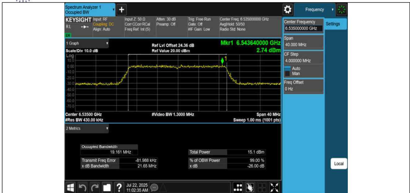
11BE20MIMO-Ant1-6535-PASS
