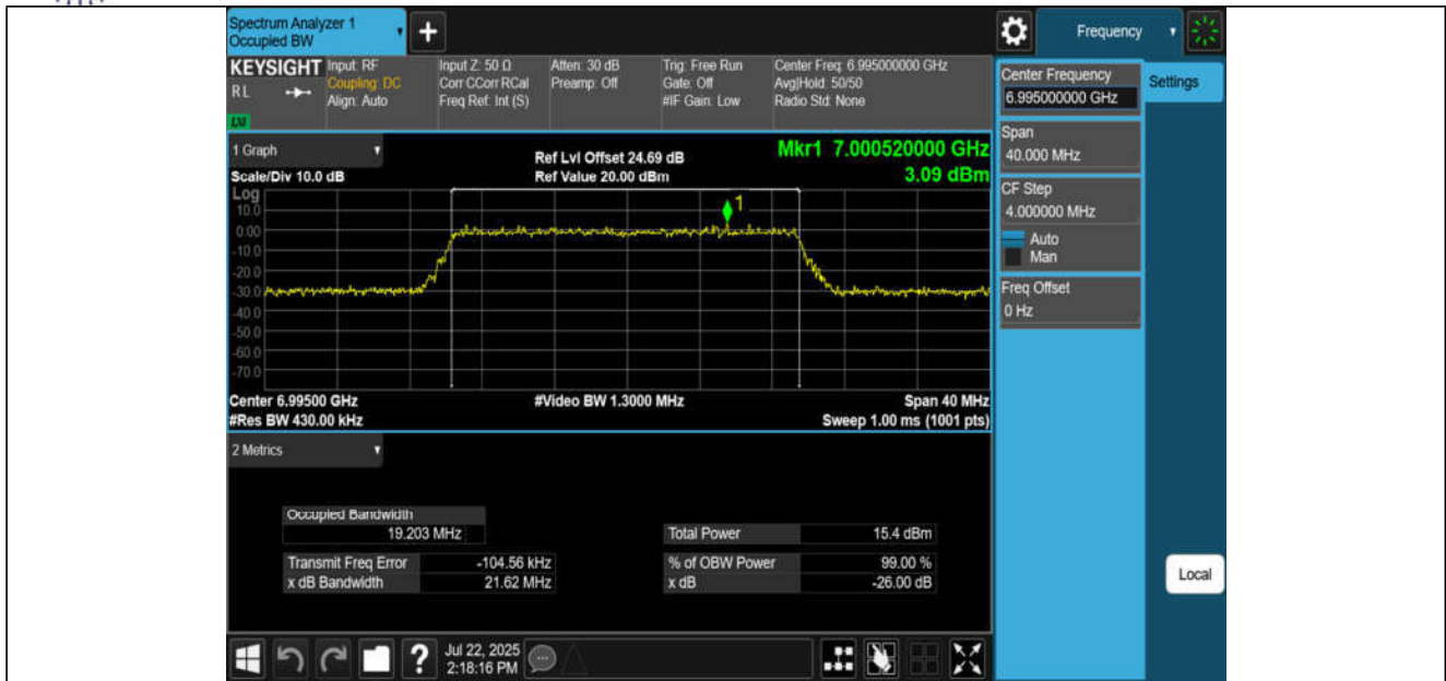
11BE20MIMO-Ant1-6995-PASS
