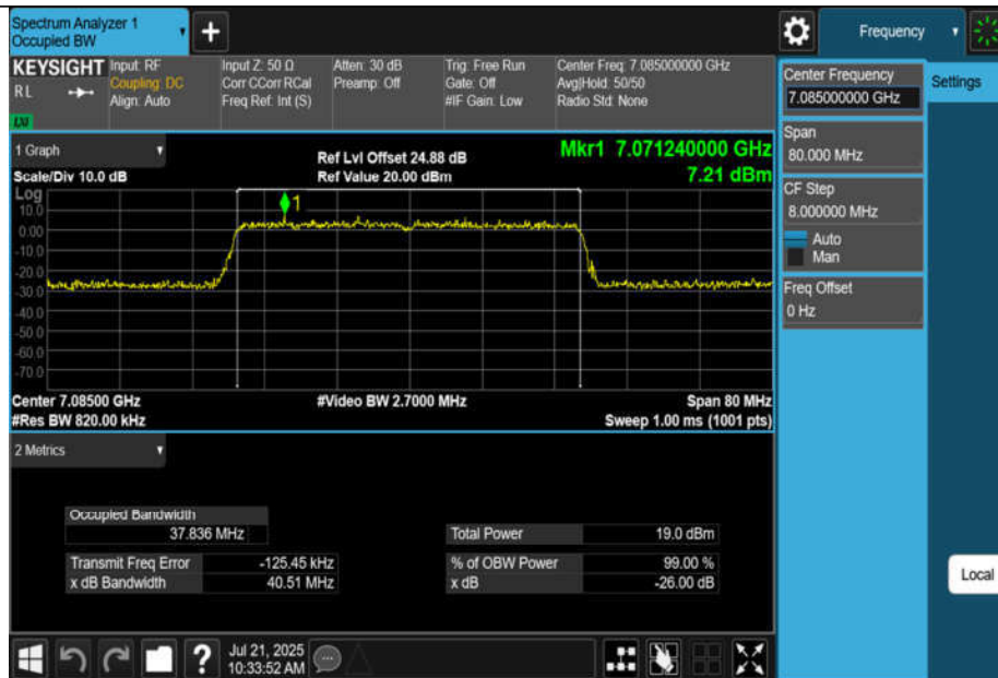
11AX40MIMO-Ant3-7085-PASS
