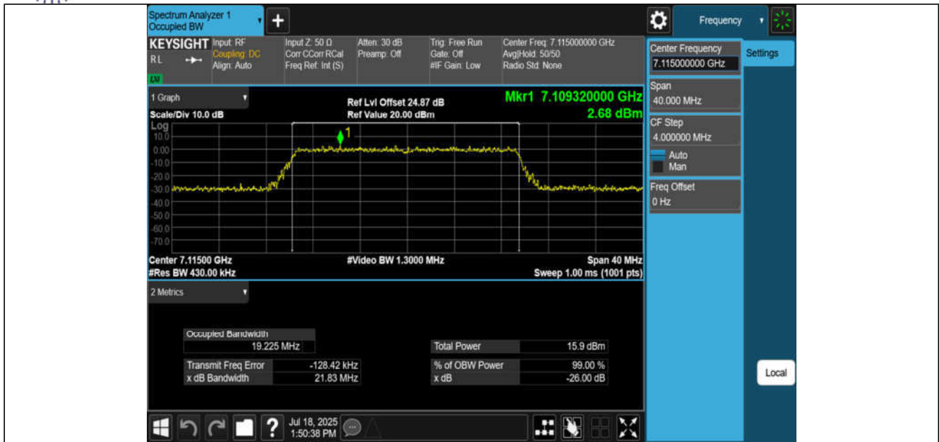
11AX20MIMO-Ant1-7115-PASS
