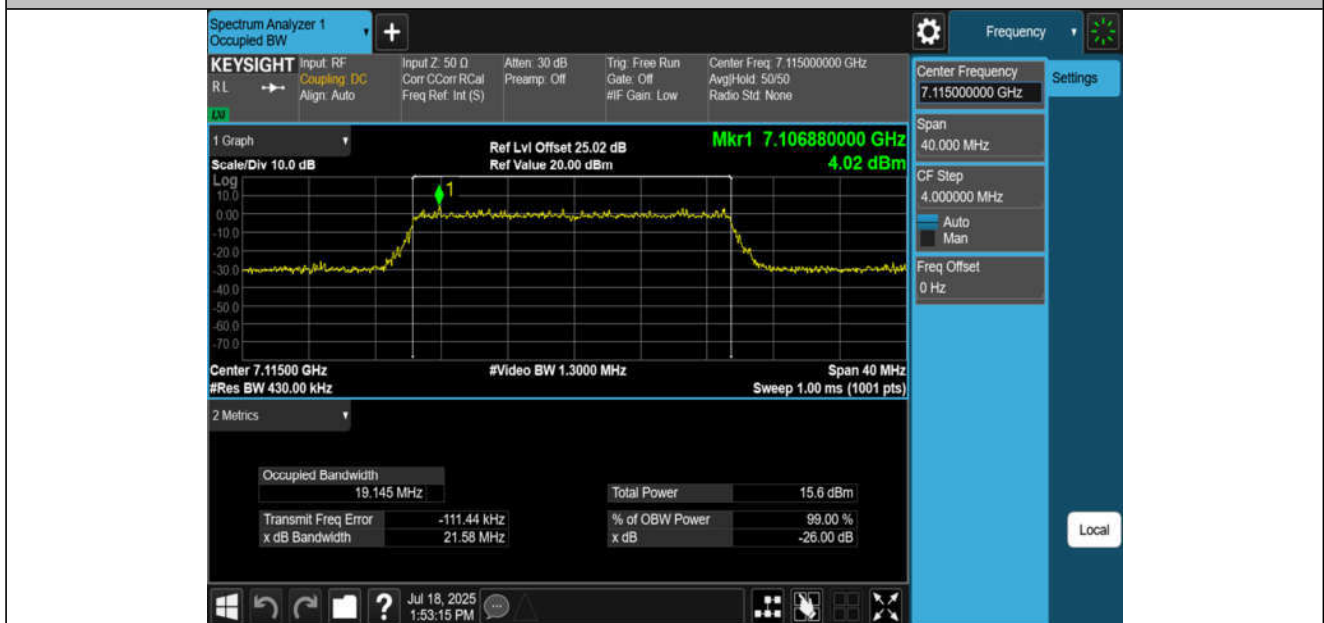
11AX20MIMO-Ant4-7115-PASS
