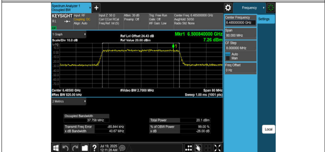
11AX40MIMO-Ant4-6485-PASS
