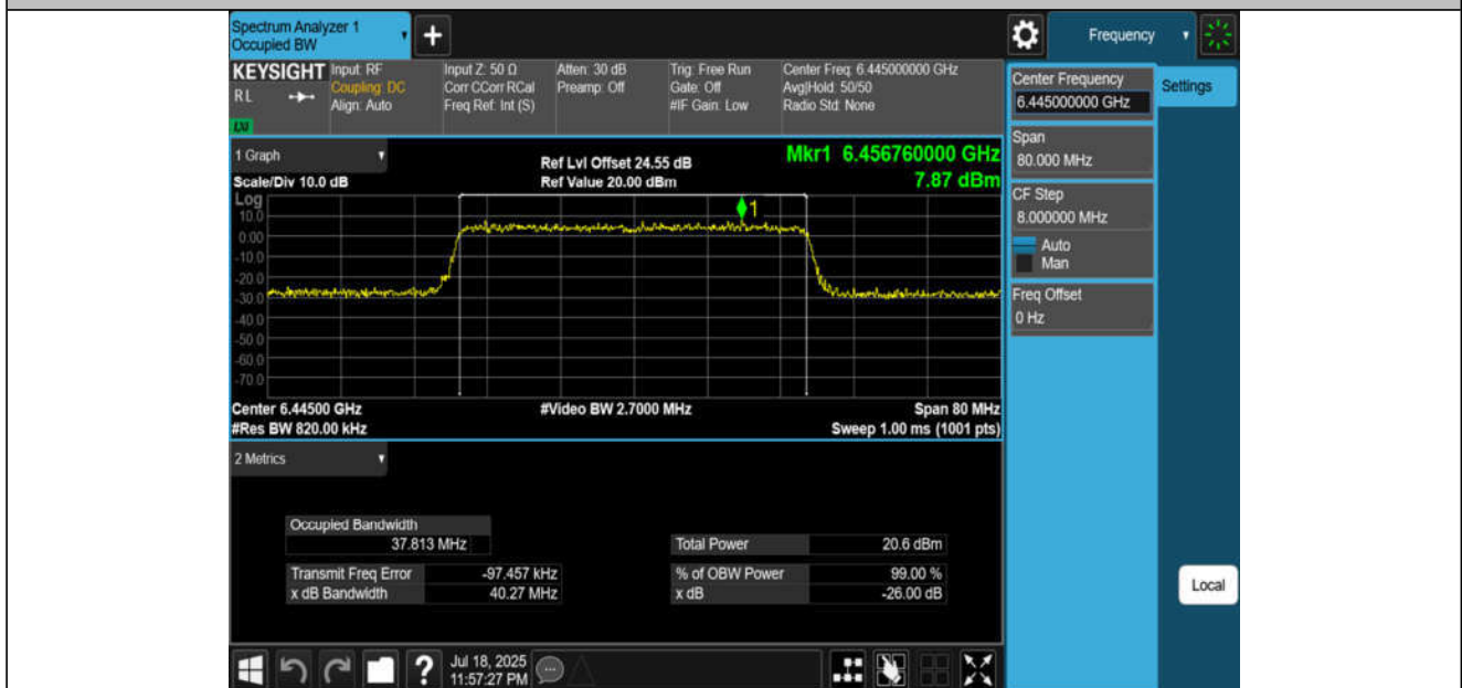
11AX40MIMO-Ant4-6445-PASS
