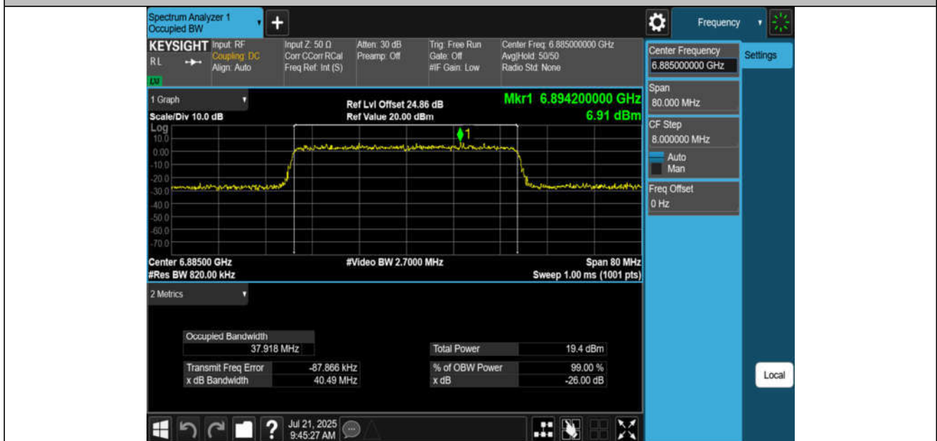
11AX40MIMO-Ant4-6885-PASS
