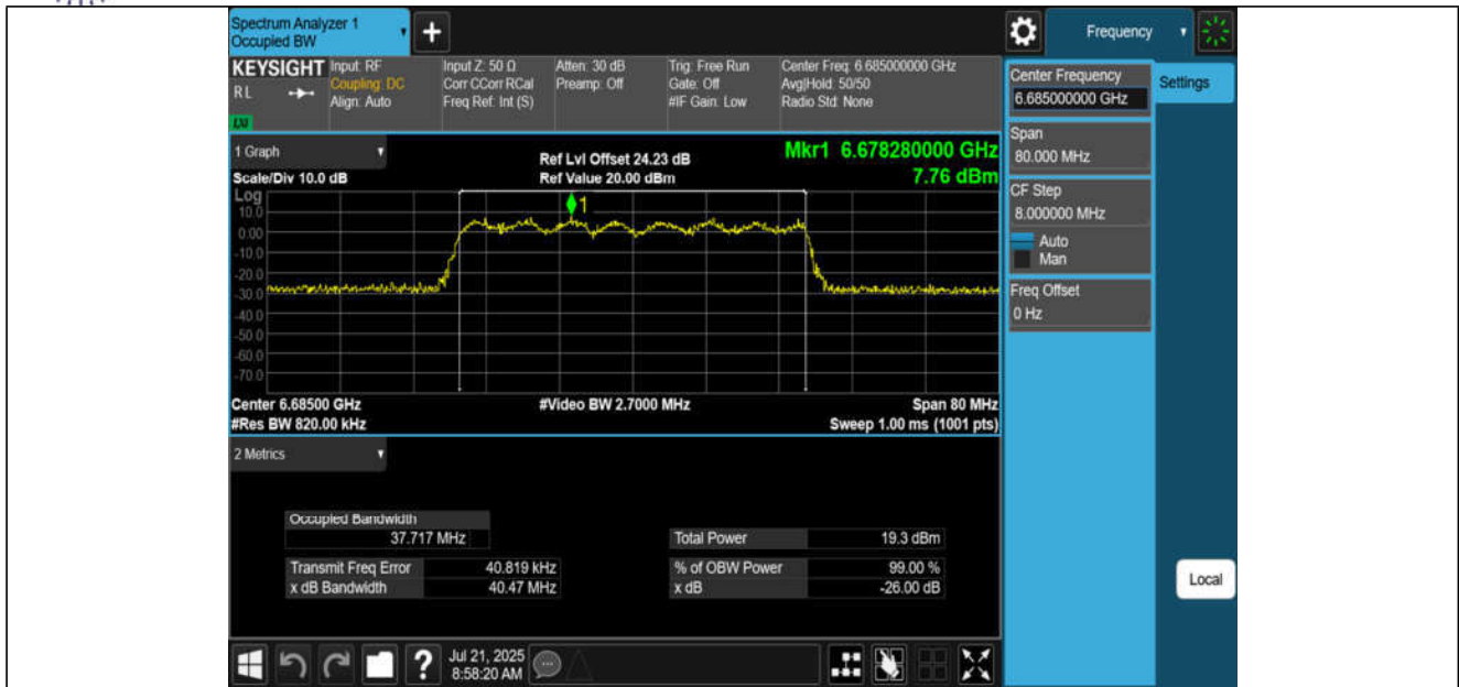
11AX40MIMO-Ant3-6685-PASS
