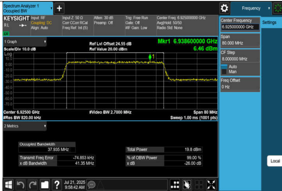
11AX40MIMO-Ant3-6925-PASS
