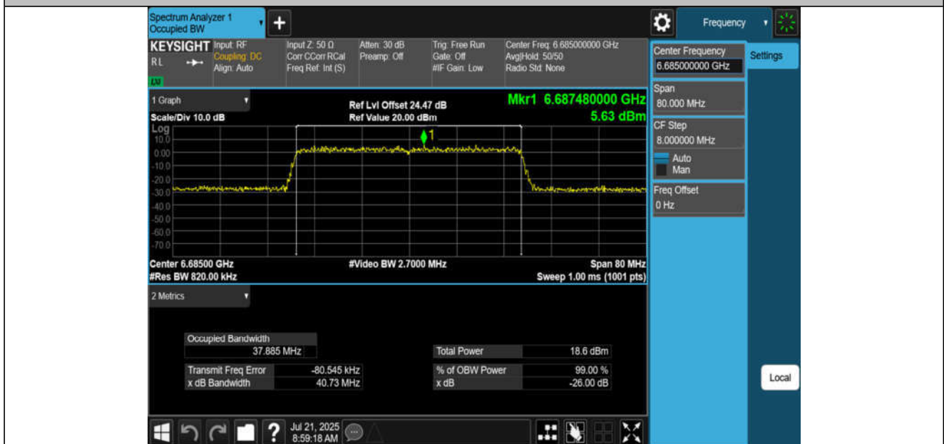
11AX40MIMO-Ant4-6685-PASS
