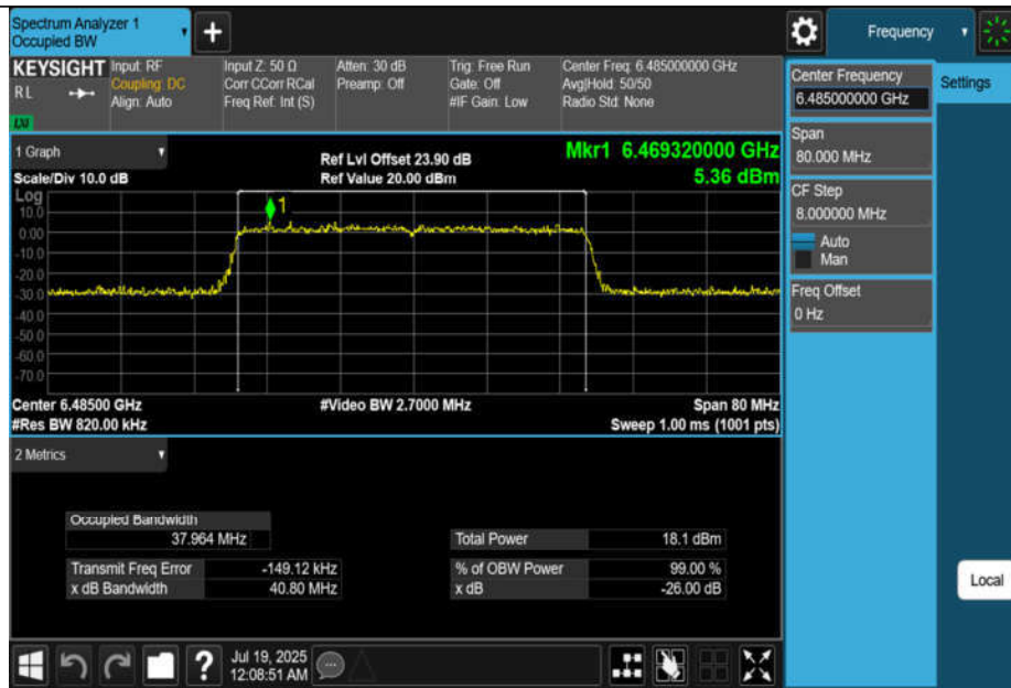
11AX40MIMO-Ant1-6485-PASS
