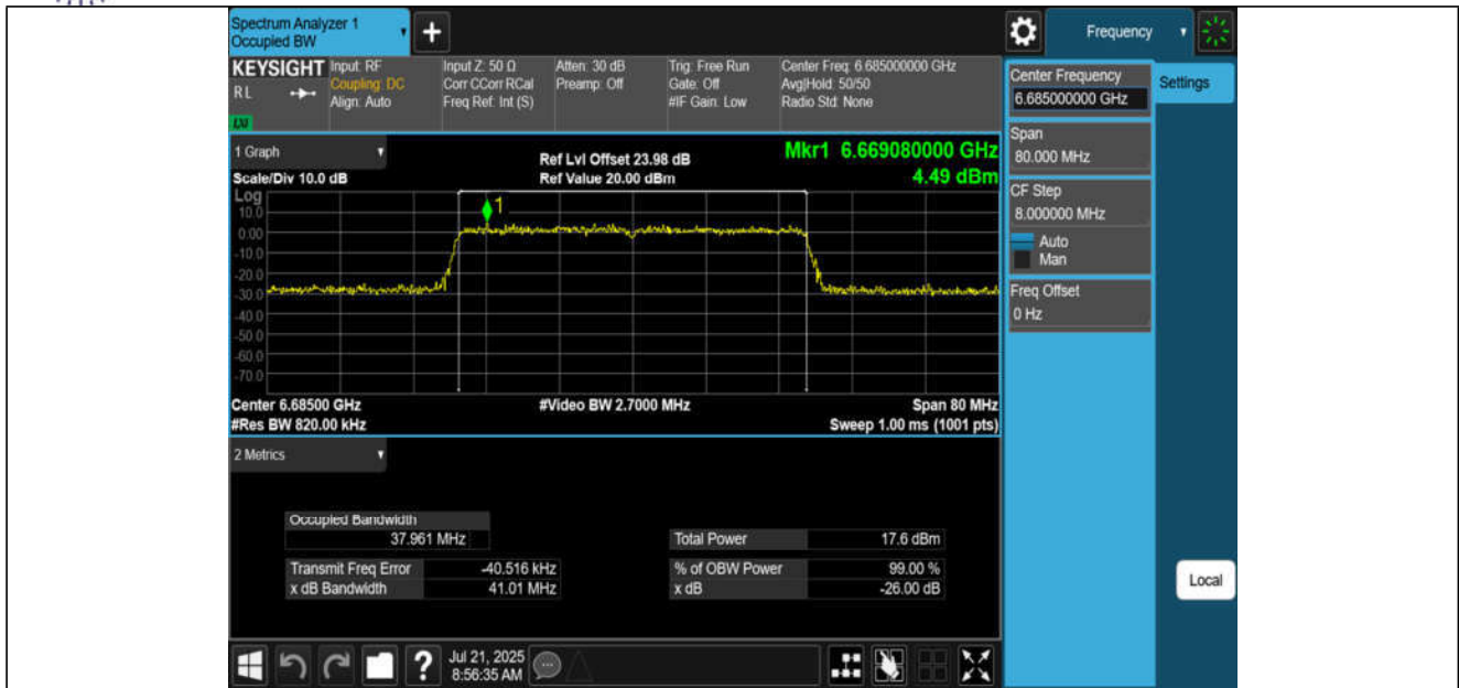
11AX40MIMO-Ant1-6685-PASS
