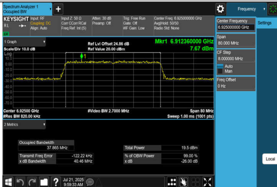
11AX40MIMO-Ant4-6925-PASS
