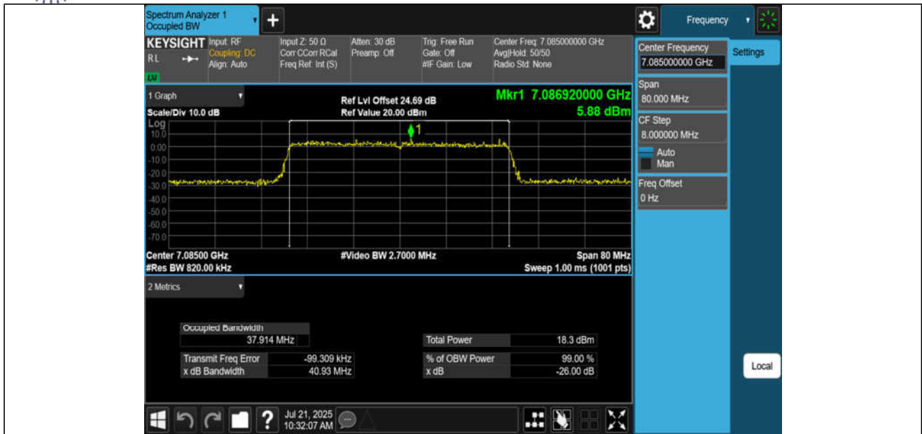
11AX40MIMO-Ant1-7085-PASS
