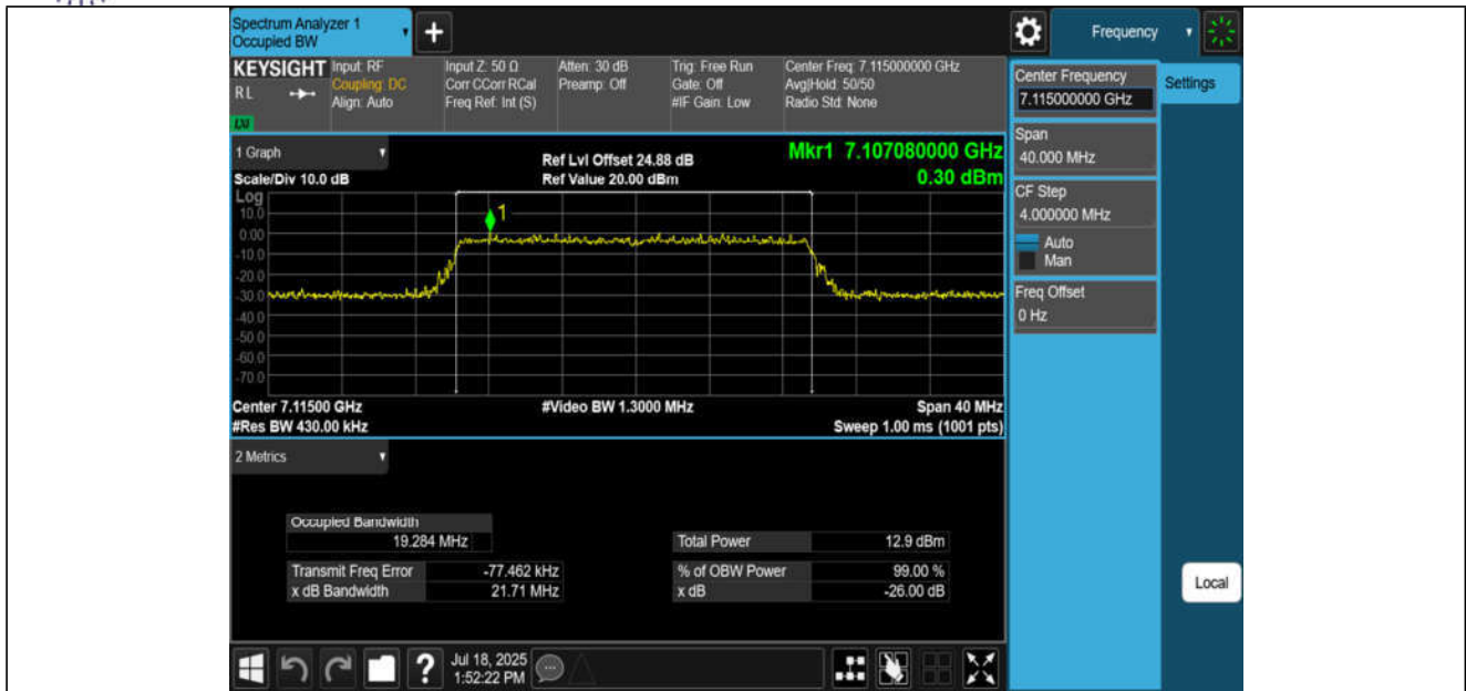
11AX20MIMO-Ant3-7115-PASS
