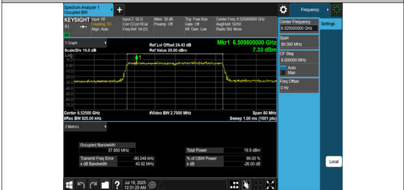
11AX40MIMO-Ant4-6525-PASS
